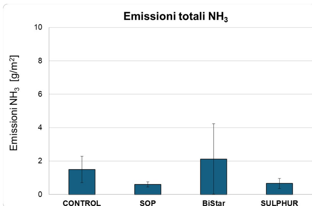
Fig. 7. Emissioni cumulative di ammoniaca
