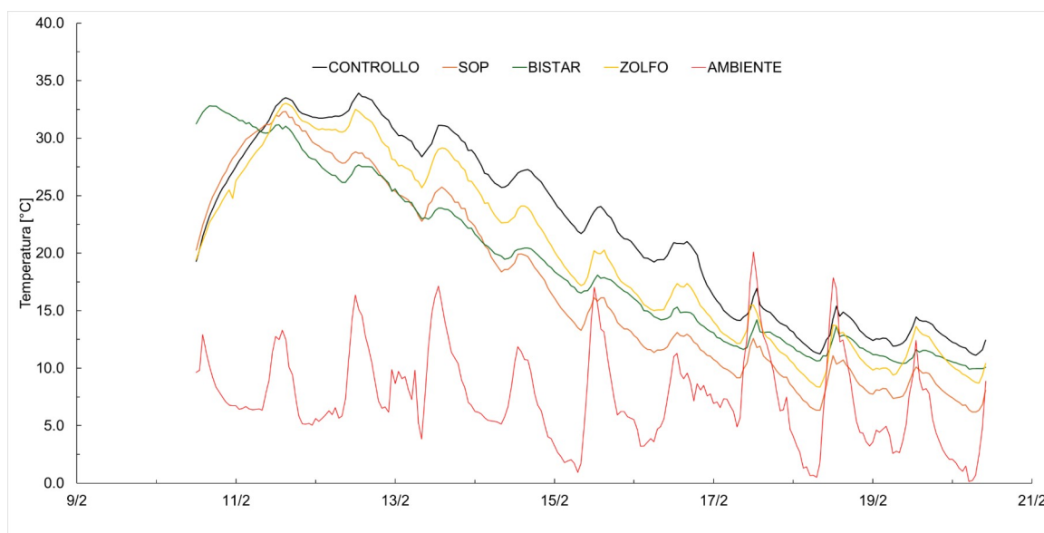
Fig. 9 Andamento della temperatura del letame durante il periodo sperimentale
