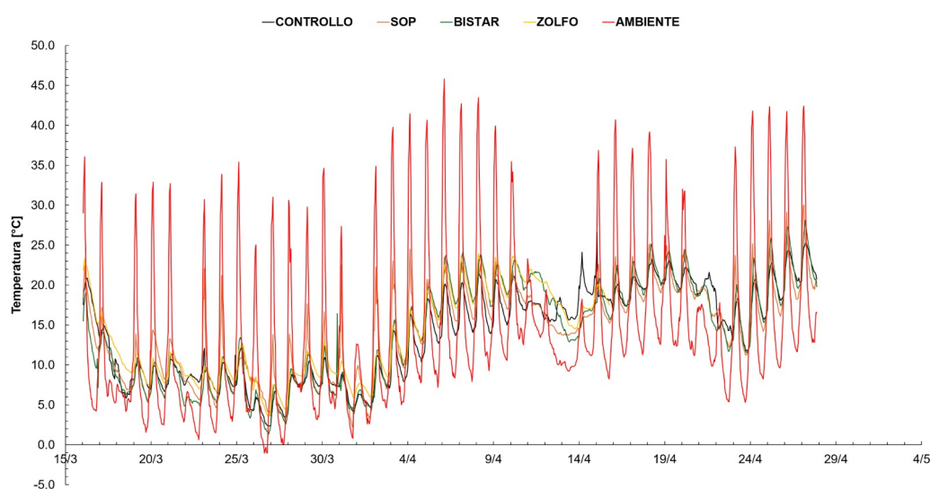
Fig. 14 Andamento della temperatura del letame durante il periodo sperimentale
