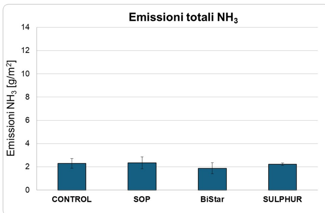
Fig. 17. Emissioni cumulative di ammoniaca
