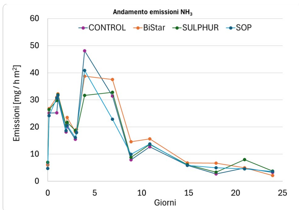
Fig. 20. Andamento temporale dei flussi emissivi di ammoniaca
