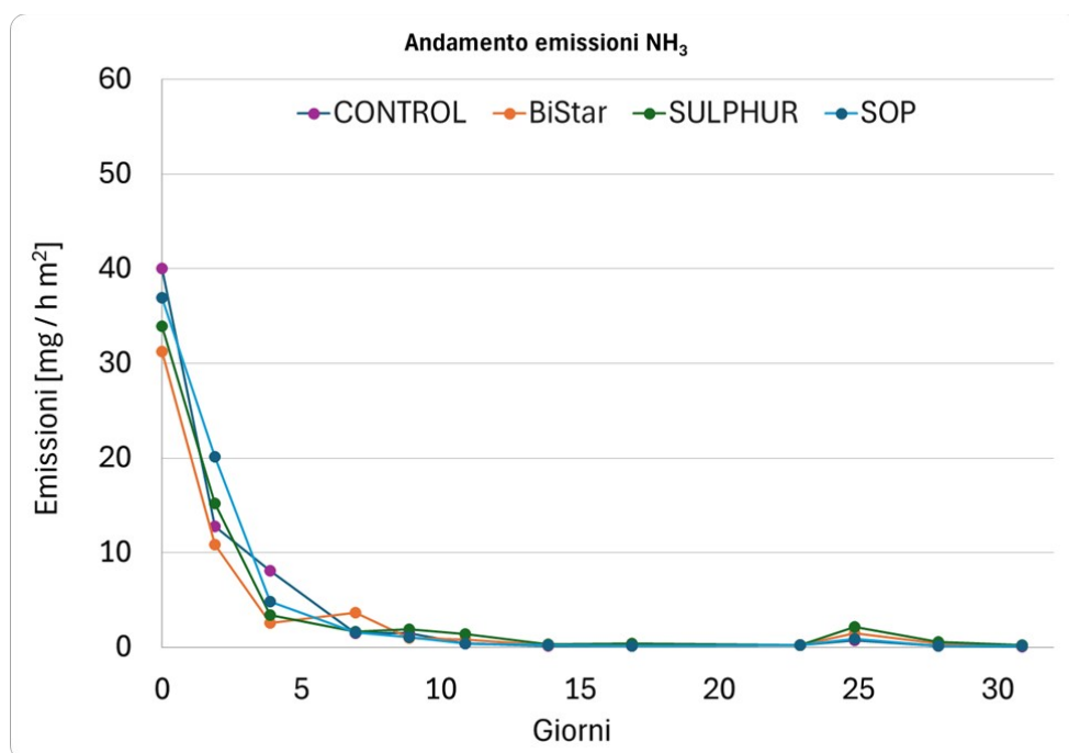
Fig. 16. Andamento temporale dei flussi emissivi di ammoniaca
