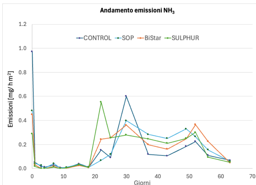
Fig. 11. Andamento temporale dei flussi emissivi di ammoniaca.
