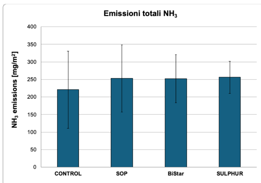
Fig. 12. Emissioni cumulative di ammoniaca.
