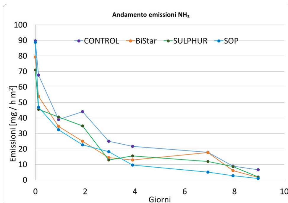
Fig. 3. Andamento temporale dei flussi emissivi di ammoniaca.
