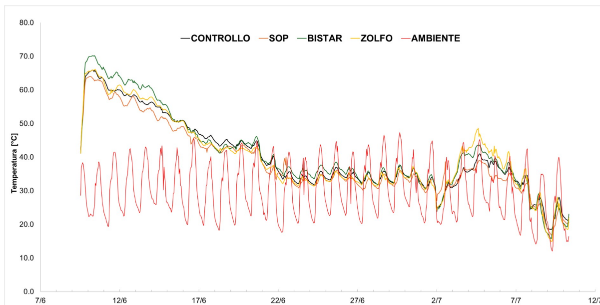
Fig. 19. Andamento della temperatura del letame durante il periodo sperimentale
