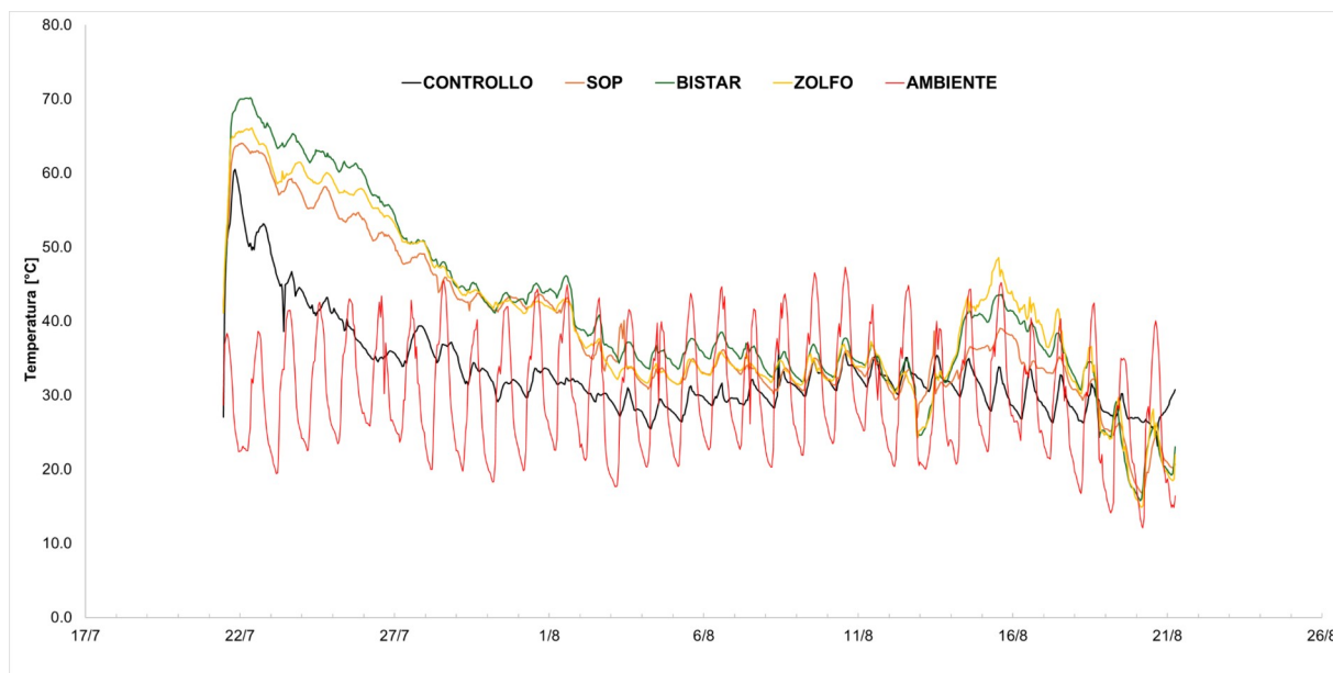
Fig. 23. Andamento della temperatura del letame durante il periodo sperimentale
