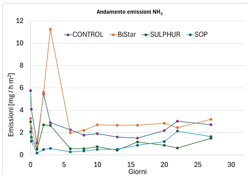
Fig. 6. Andamento temporale dei flussi emissivi di ammoniaca
