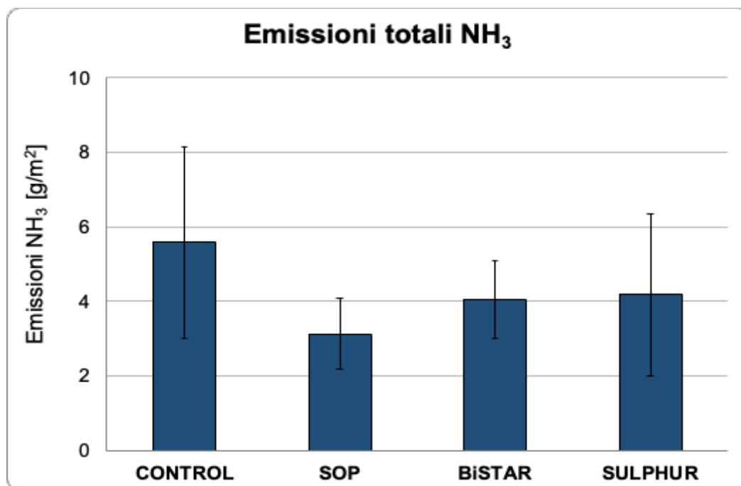
Fig. 4. Emissioni cumulative di ammoniaca
