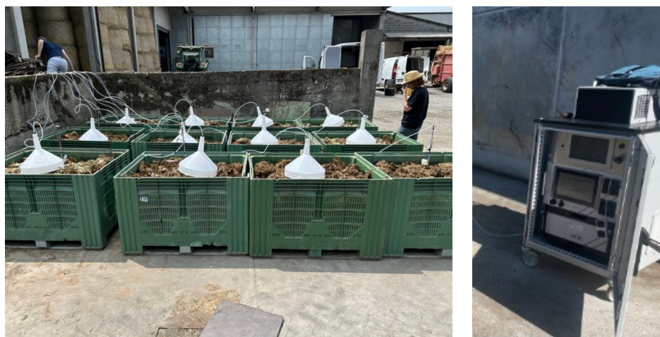
Fig. 2. Apparato sperimentale per la misura delle emissioni di \text{NH}_3 : a) installazione delle camere dinamiche di campionamento (funnel system) sulle unità sperimentali; b) analizzatore di gas ad alta risoluzione (ETG 8900 QEPAS) collegato al sistema di campionamento multipunto e di acquisizione automatica dei dati.
