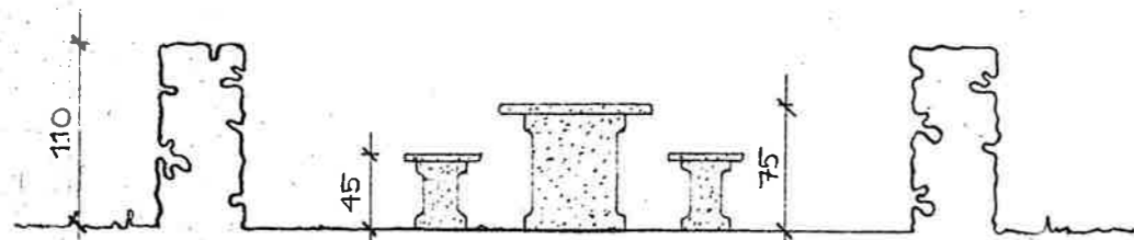
SEZIONI BB
