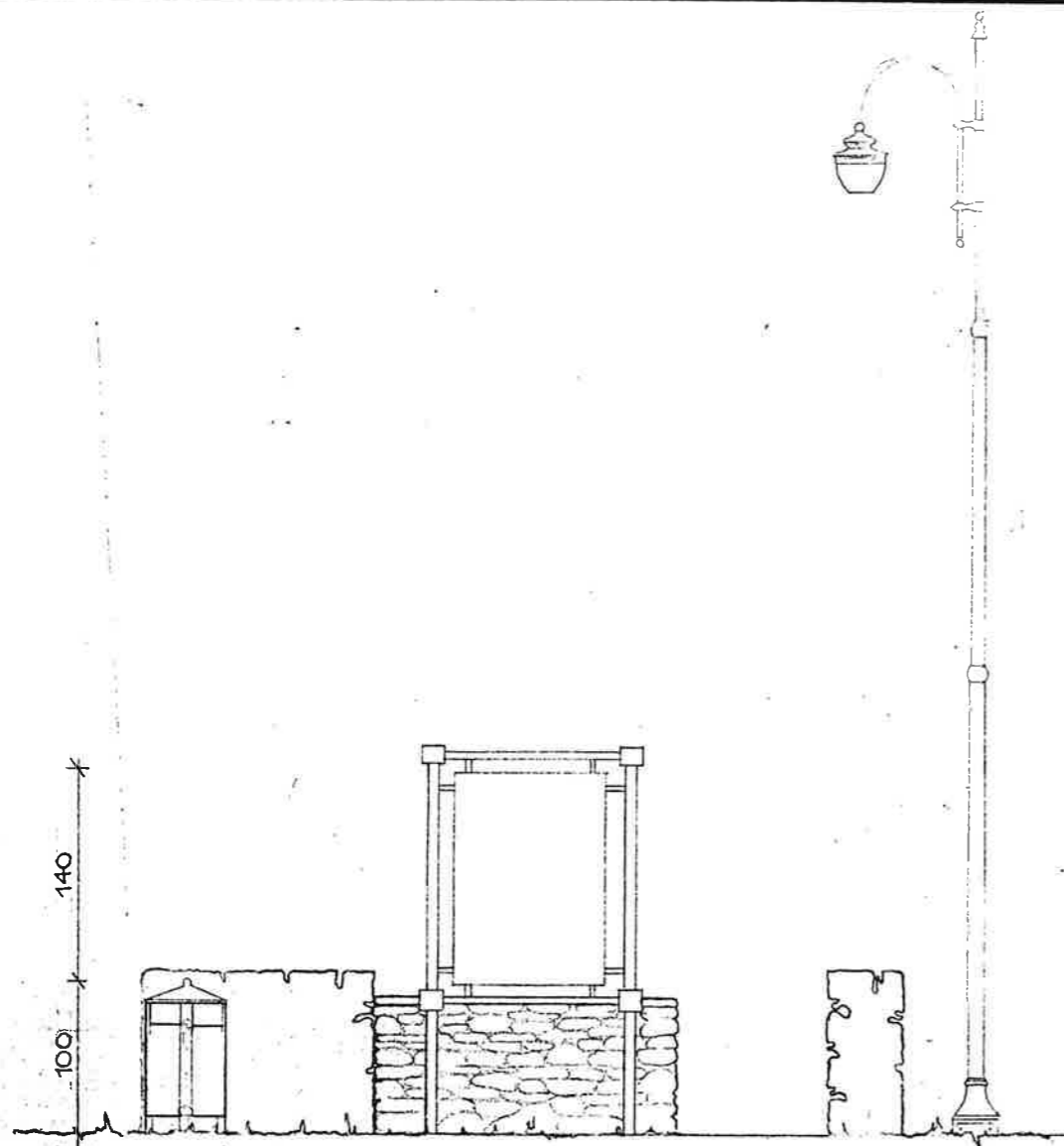
PROSPETTO AA
