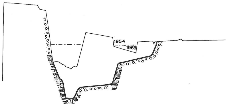
Fig. 5b - Evoluzione dell'alveo evidenziata dal confronto tra i rilievi del 1971 e del 1986; sono inoltre rappresentati il livello di massima piena raggiunto nel 1968 ed i canali attivi nell'anno indicato.
