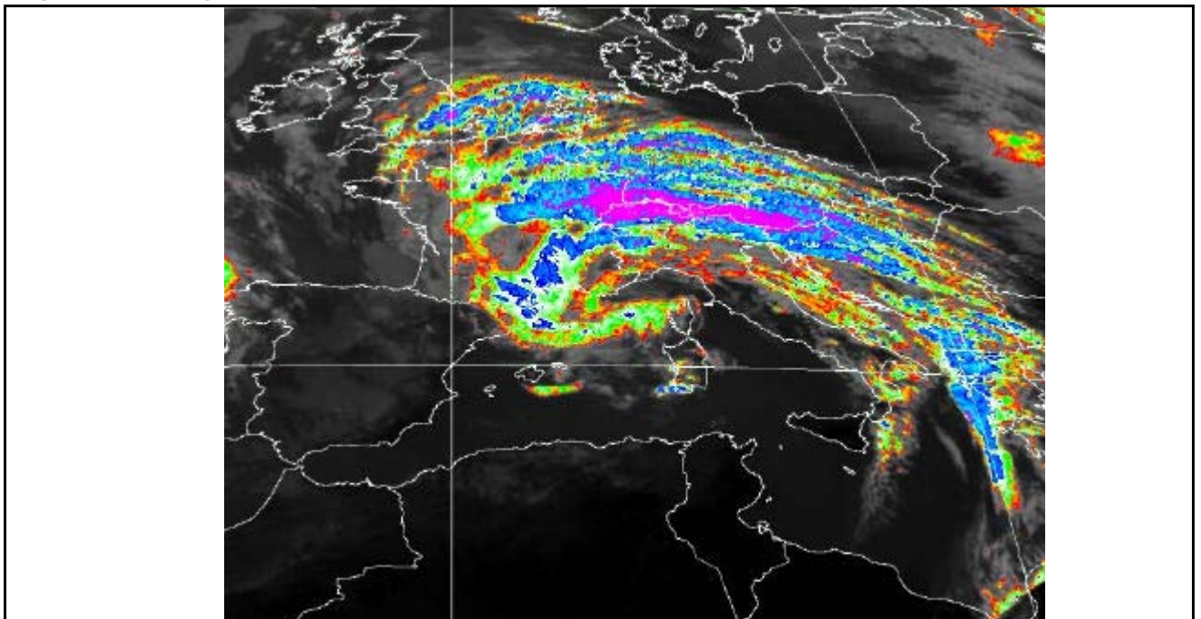
Figura 13 : immagine METEOSAT delle 8:30 UTC del 4/5/99 (infrarosso)
