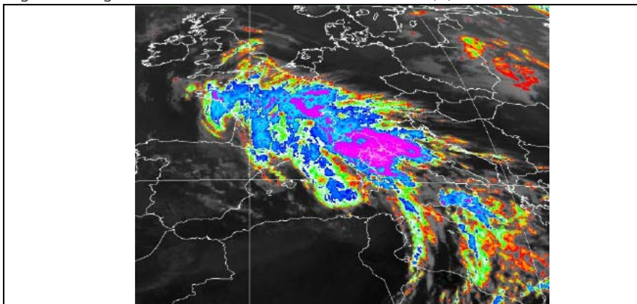
Figura 4: Immagine METEOSAT nell'infrarosso delle 2130 UTC del 3/5/99
