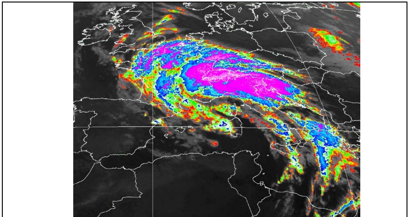
Figura 11: immagini METEOSAT delle 2 30 UTC del 4/5/99 (infrarosso)
