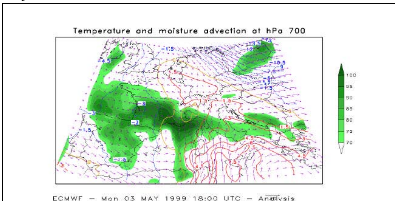
Figura 3: Analisi delle 18 UTC del 3/5/99 dei campi di umidità relativa (livelli di colore), temperatura (linee) e vento (freccette) a 700 hPa
