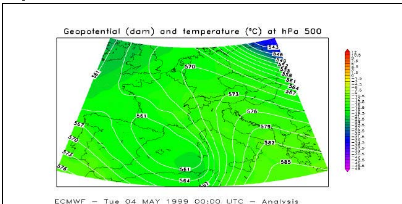
Figura 6 : Analisi delle 00 UTC del 4/5/99 dei campi di altezza geopotenziale (linee continue) e temperatura (livello di cobre) a 500 hPa
