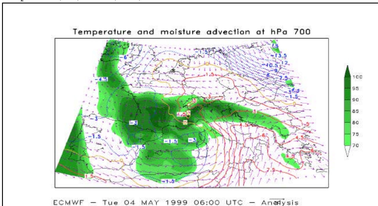
Figura 20 : Analisi delle 6 UTC del 4/5/99 dei campi di umidità relativa (livelli di colore), temperatura (linee) e vento (freccie) a 700 hPa
