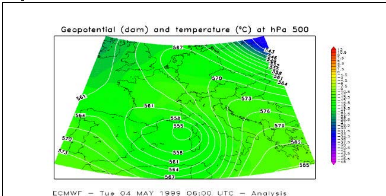
Figura 7 : Analisi delle 06 UTC del 4/5/99 dei campi di altezza geopotenziale (linee continue) e temperatura (livello di cobre) a 500 hPa
