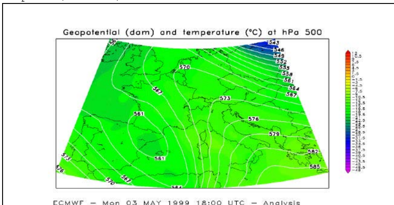
Figura 2: Analisi delle 18 UTC del 3/5/99 dei campi di altezza geopotenziale (linee continue) e temperatura (livello di cobre) a 500 hPa
