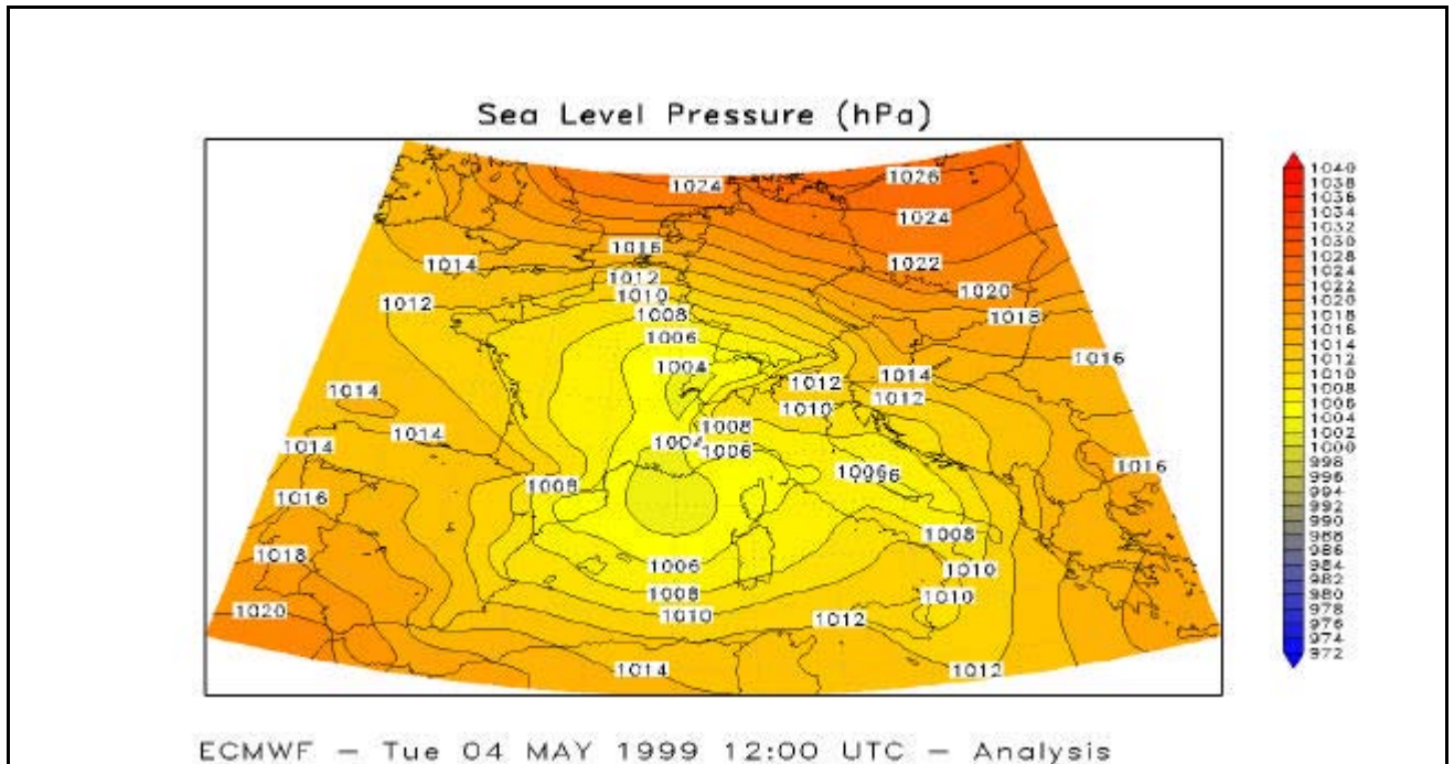
Figura 10 :Analisi delle 12 UTC del 4/5/99 del campo di pressione ridotta al livello del mare
