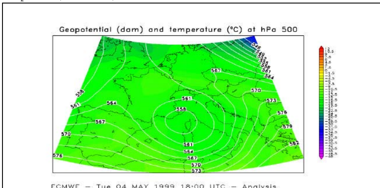
Figura 9 : Analisi delle 18 UTC del 4/5/99 dei campi di altezza geopotenziale (linee continue) e temperatura (livello di colore) a 500 hPa
