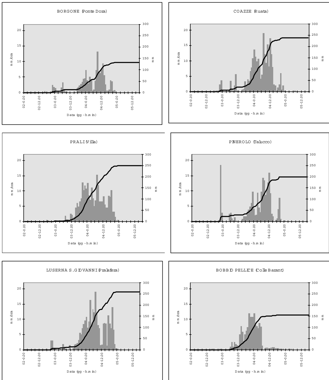
Figura 26 : Pioggia cumulata e intensità di alcune stazioni significative per i giorni 03 - 04 - maggio 1999 - valli Susa, Sangone, Chisone, Germanasca, Pellice e Po
