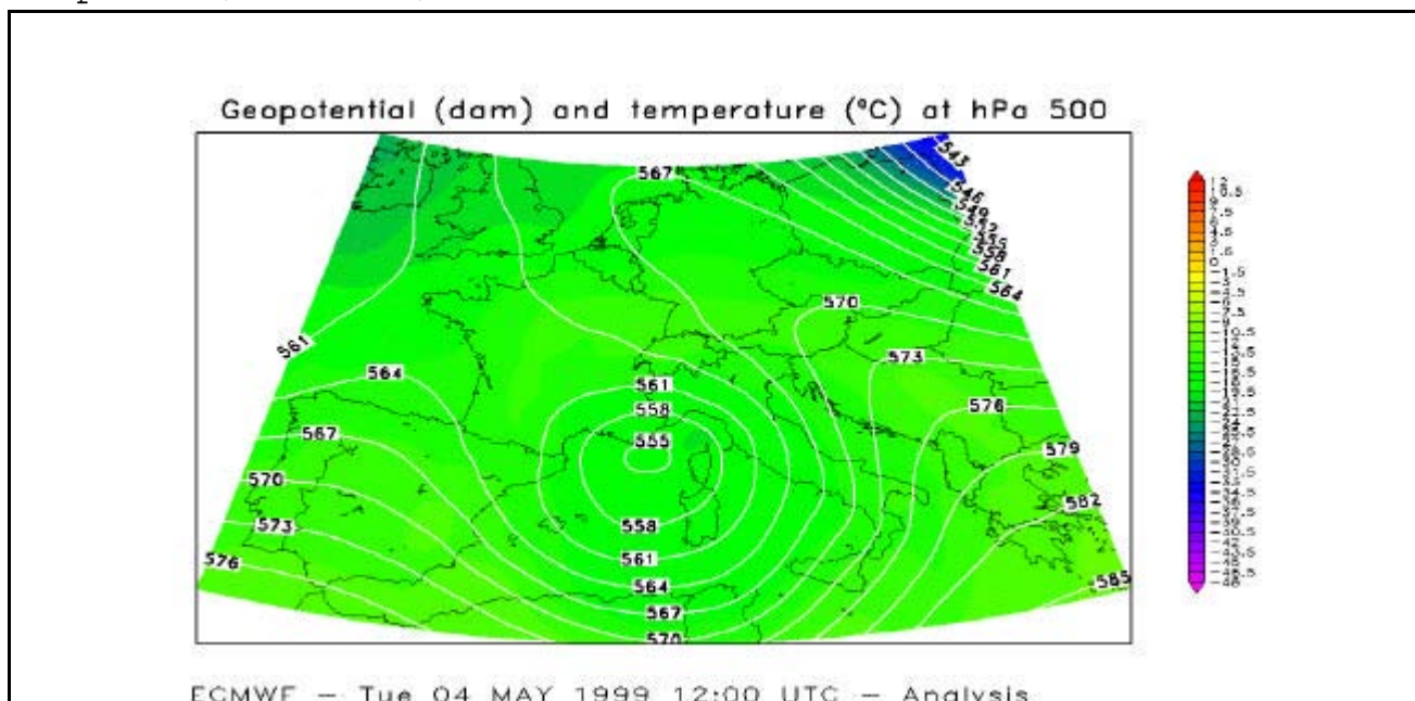
Figura 8 : Analisi delle 12 UTC del 4/5/99 dei campi di altezza geopotenziale (linee continue) e temperatura (livello di colore) a 500 hPa
