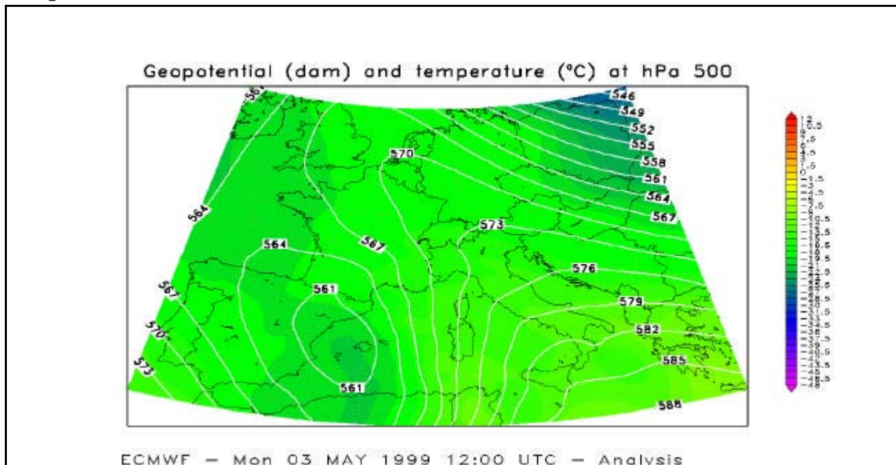
Figura 1: Analisi delle 12 UTC del 3/5/99 dei campi di altezza geopotenziale (linee continue) e temperatura (livello di cobre) a 500 hPa
