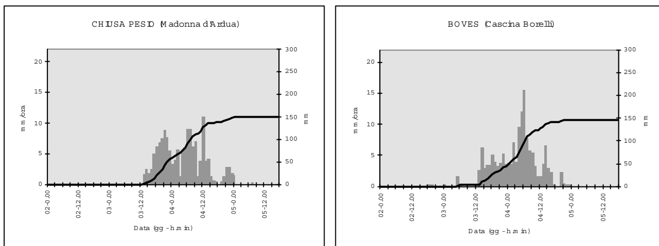
Figura 27: Pieggià cumulatà e intensità di alcune stazioni significatìve per i giorri 03 - 04 maggio 1999 - Cuneese meridionale
