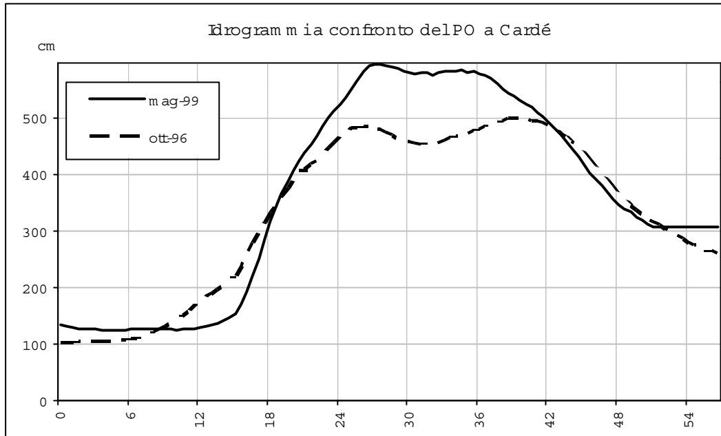
Figura 39 : Livelli idrometrici del Po a Cardè nei due eventi a confronto
