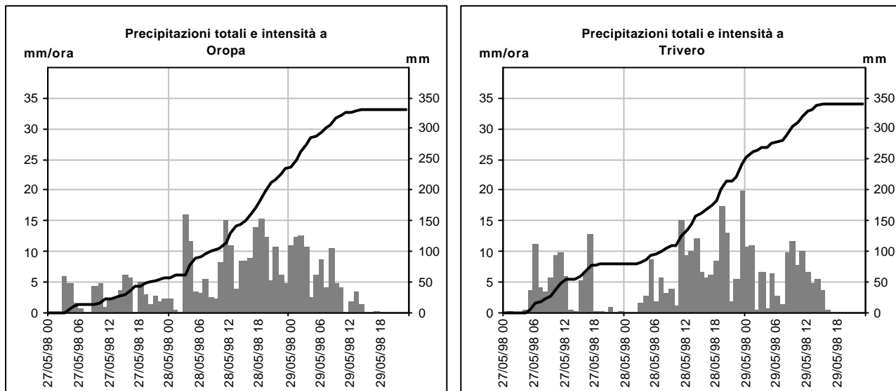
Figura 6 b - Pioggia cumulata e intensità di alcune stazioni significative per i giorni 27-28-29 maggio 1998
