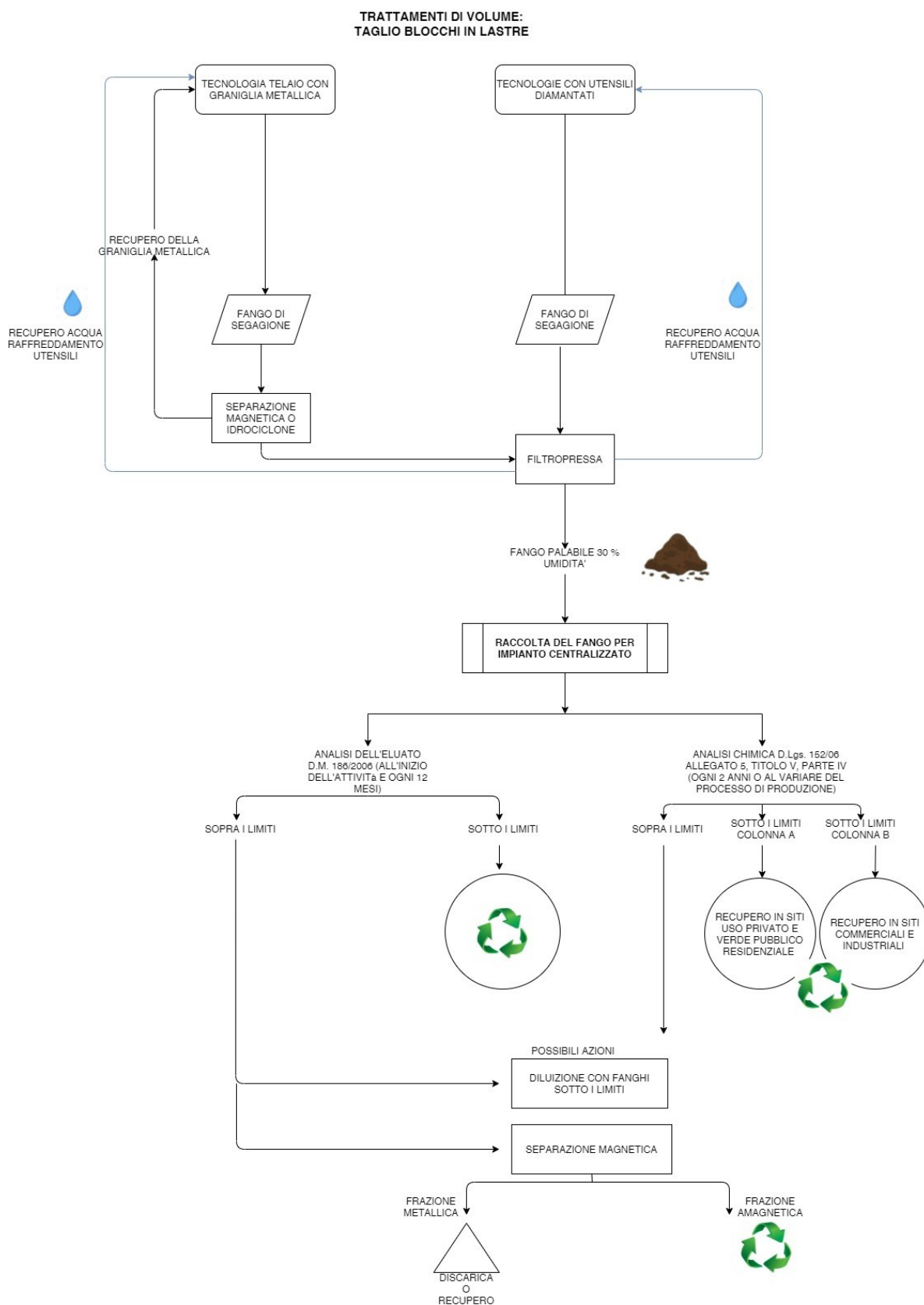
Figura 15.12: Flow chart del funzionamento dell'impianto centralizzato di raccolta dei fanghi derivanti dalla lavorazione delle pietre ornamentali e processo per renderlo sottoprodotto. Elaborazione grafica a cura del Politecnico di Torino.
