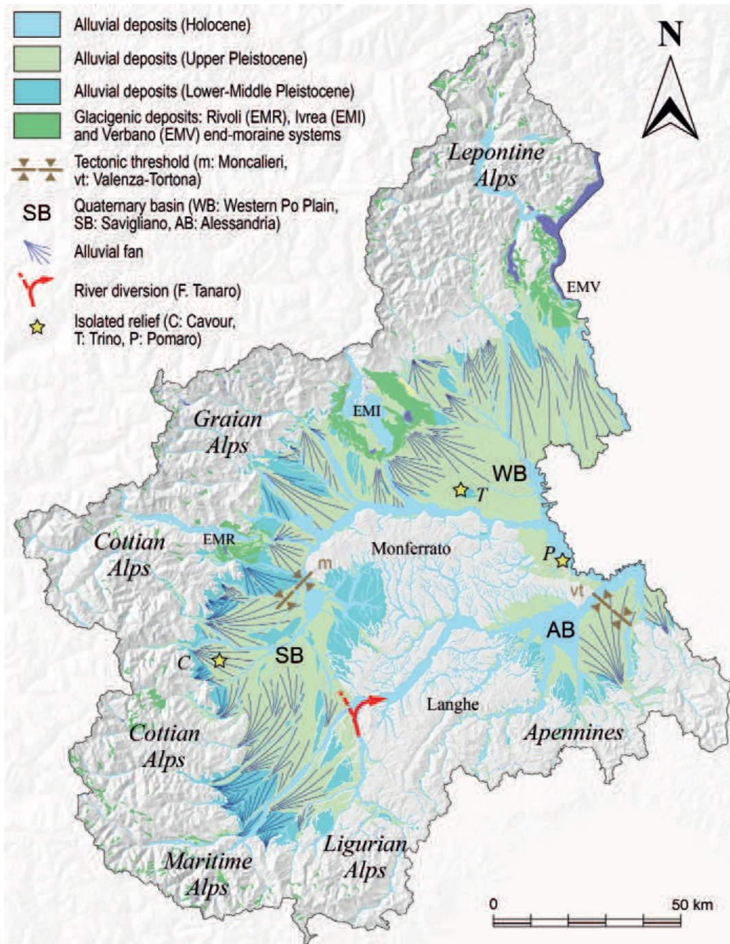
Figura 11.1.8 - Carta con distribuzione dei depositi quaternari e dei bacini sinorogenici quaternari nella regione Piemonte (Piana et al., 2017a).
