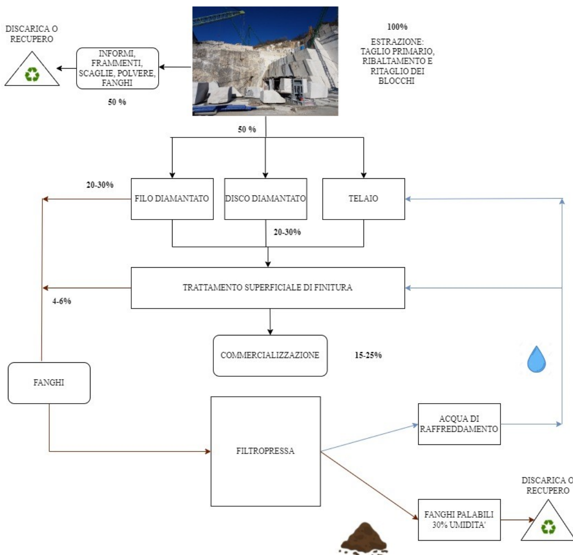
Figura 15.1. Schema rappresentativo del processo di estrazione e lavorazione dei materiali lapidei con indicazione della percentuale di residuo e prodotto derivanti da ogni fase. (Elaborazione grafica a cura del Politecnico di Torino; fonte delle percentuali di residui prodotti.
