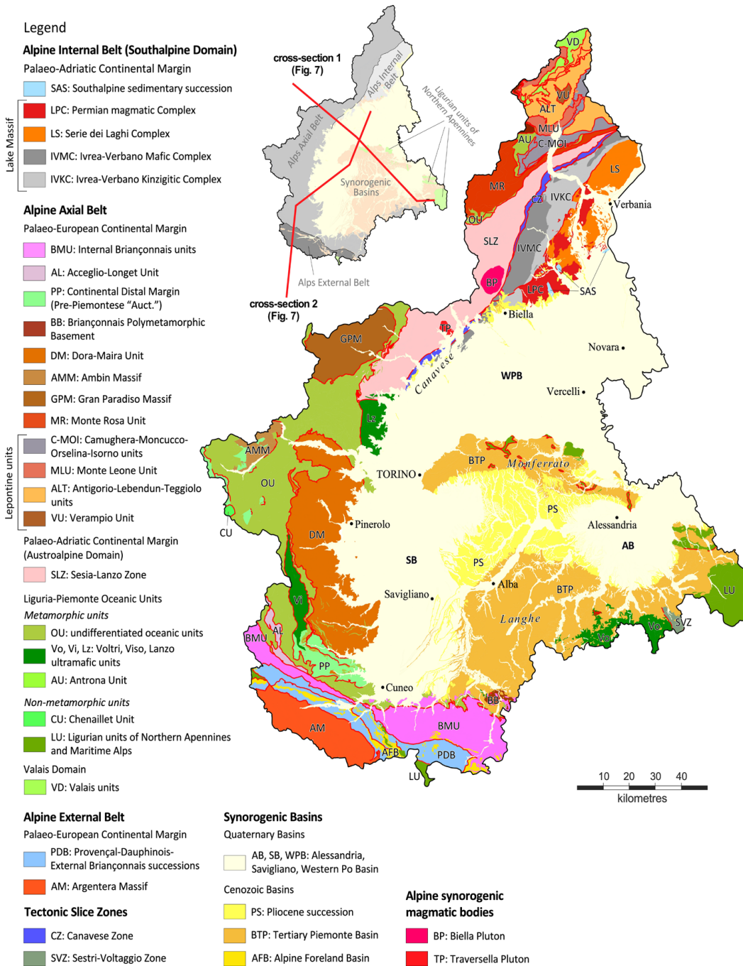
Figura 11.1.7 - Schema tettonico della Regione Piemonte (Piana et al., 2017; Barale et al., 2020).
