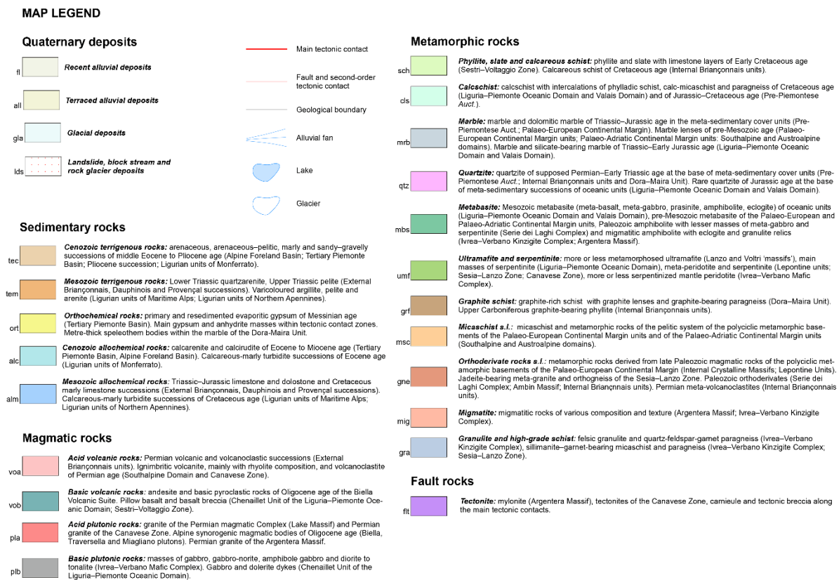
Figura 11.5.6 – Elenco semplificato delle principali tipologie di rocce affioranti nella Regione Piemonte. (Barale et al.,2017).
