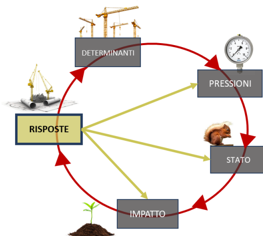
Figura 20.2 Schema del modello DPSIR (Rielaborazione da ISPRA, 2019)
