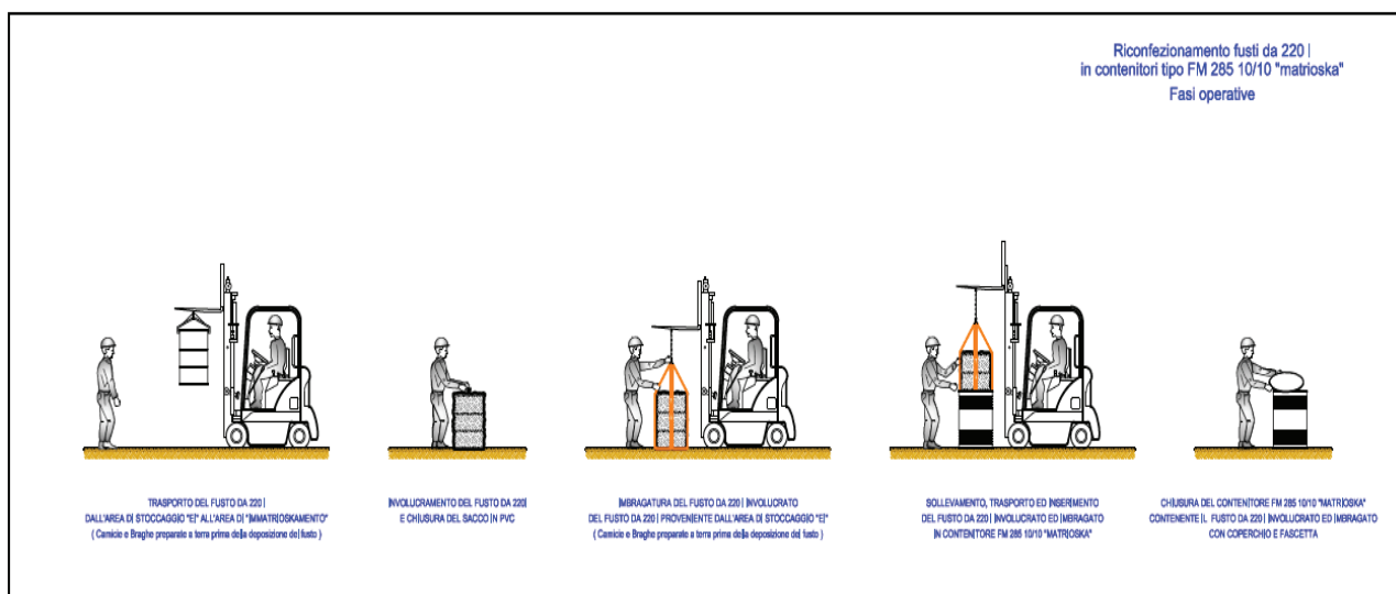
Figura 2-64 – Attività di predisposizione dei fusti al trasporto (schema)
