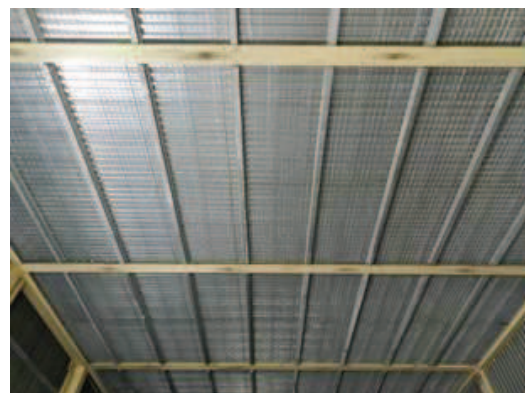
Figura 2-56 – Attività di montaggio della rete per successiva posa dell'intonaco ignifugo
