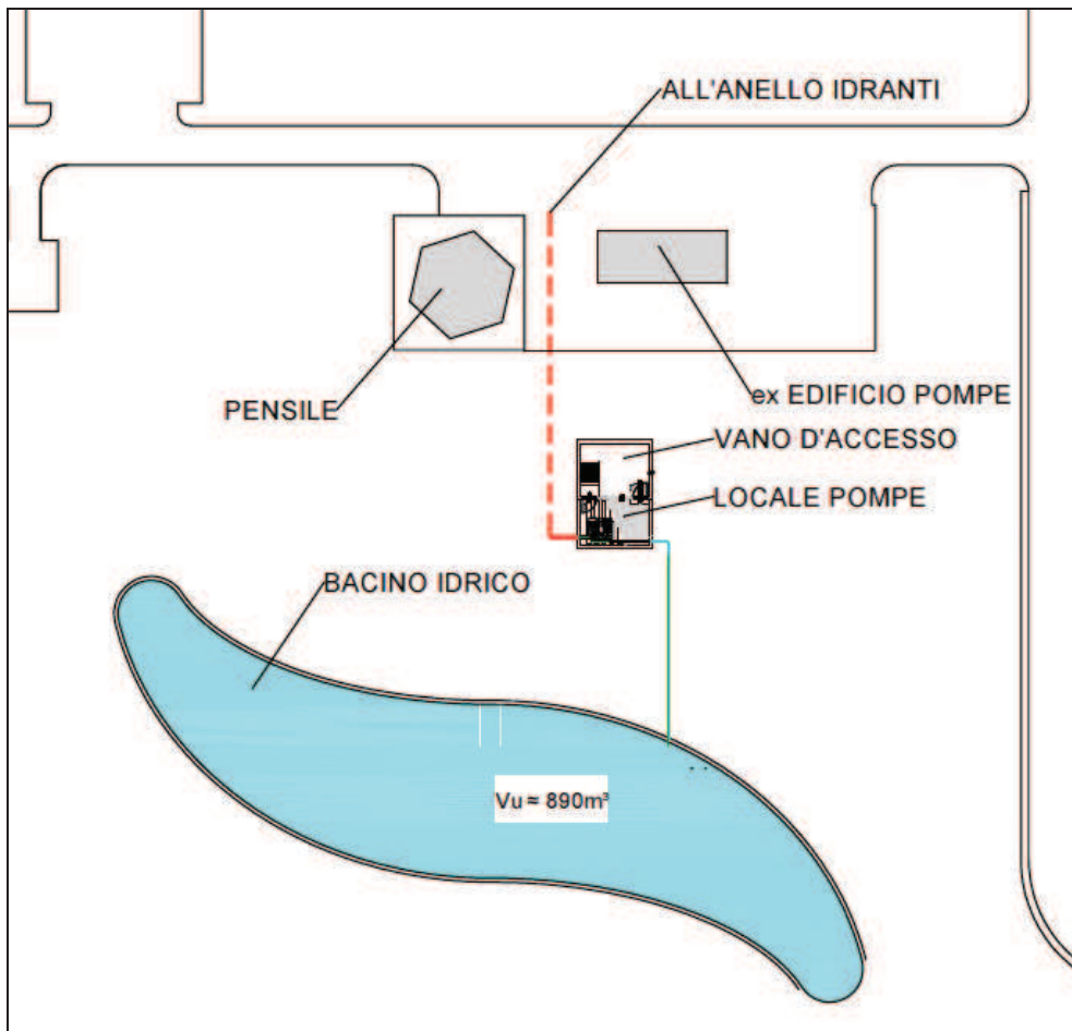
Figura 2-51 – Layout degli interventi previsti
