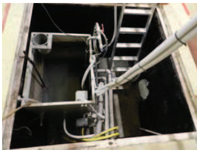
Figura 2-35 – Rimozione del serbatoio SR1 ed inserimento nuovo serbatoio
