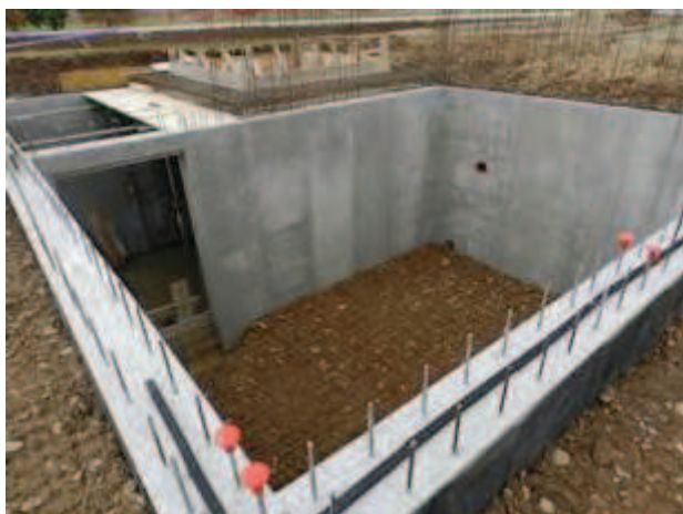
Figura 2-58 – Attività di realizzazione dell'edificio per il posizionamento del sistema di pressurizzazione
