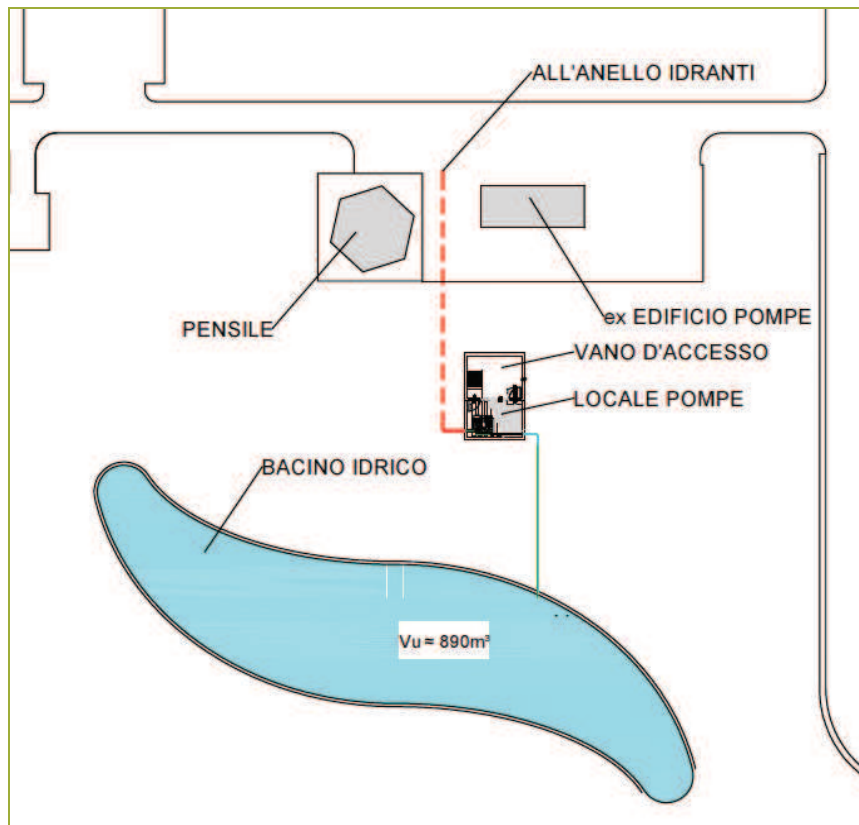
Figura 2-75 – Layout degli interventi previsti
