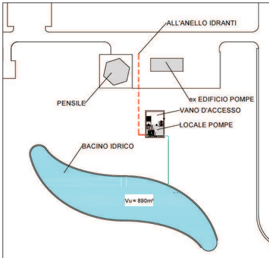
Figura 2-68 – Layout degli interventi previsti
