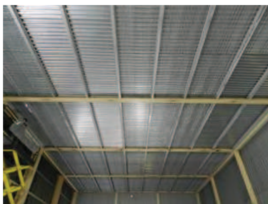
Figura 2-59 – Attività di montaggio della rete per successiva posa dell'intonaco ignifugo
