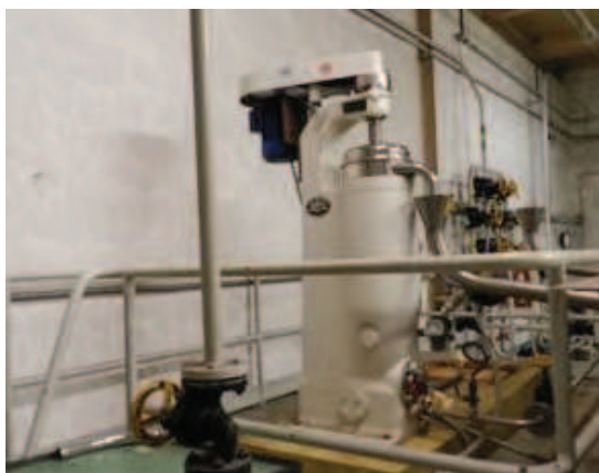
Figura 2-34 – Smantellamento delle supercentrifughe
