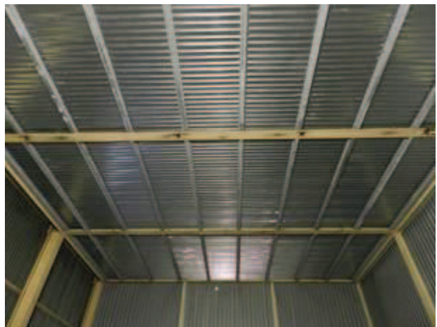
Figura 2-51 – Attività di montaggio della lamiera grecata sul soffitto del locale B106
