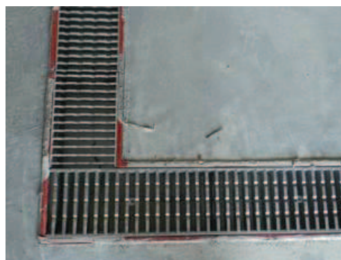
Figura 2-53 – Attività di montaggio delle canaline del sistema drenaggi all'interno del B106
