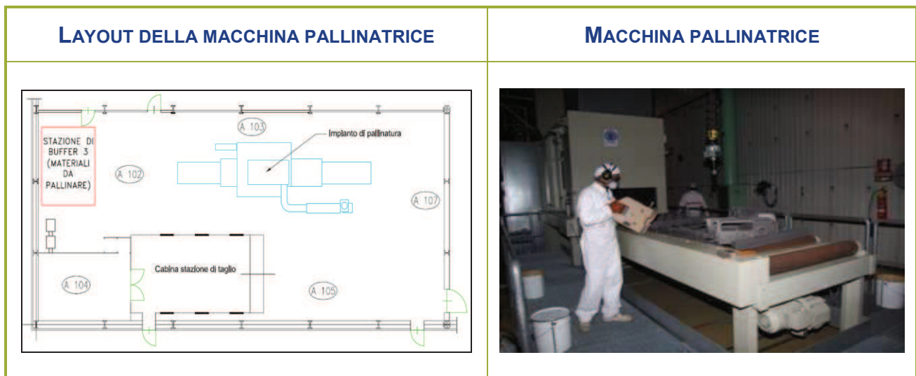
Figura 2-7 – Macchina pallinatrice
