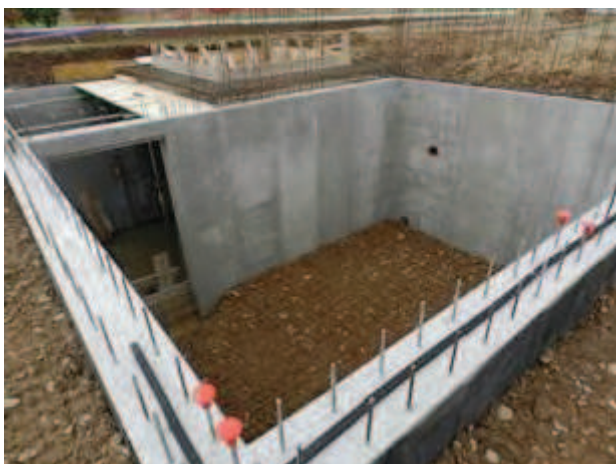
Figura 2-77 – Attività di realizzazione dell'edificio per il posizionamento del sistema di pressurizzazione
