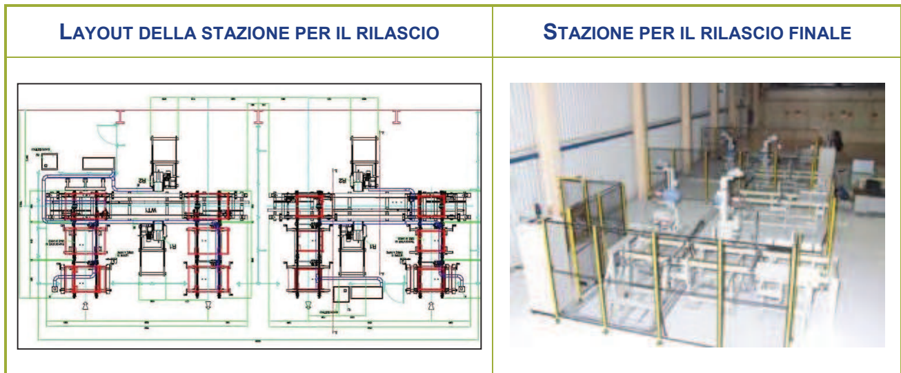
Figura 2-8 – Stazione per il rilascio finale dei materiali smantellati
