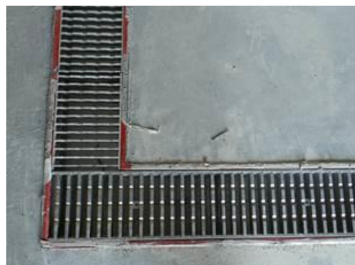
Figura 2-53 – Attività di montaggio delle canaline del sistema drenaggi all'interno del B106
