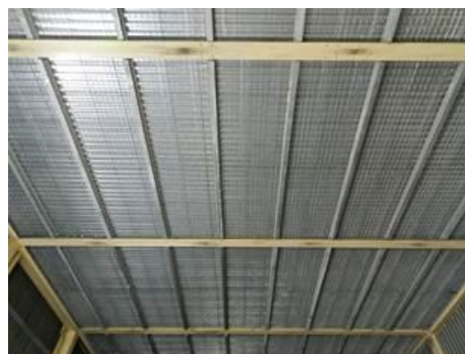
Figura 2-56 – Attività di montaggio della rete per successiva posa dell'intonaco ignifugo
