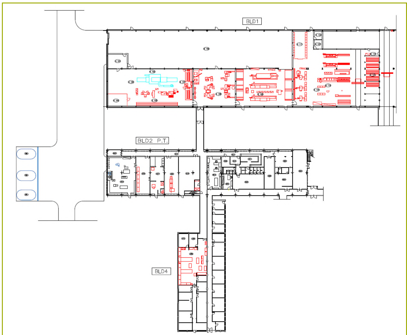
Allegato [A.1.] – Layout Aree di Lavoro (in rosso e in blu le apparecchiature smartellate)
