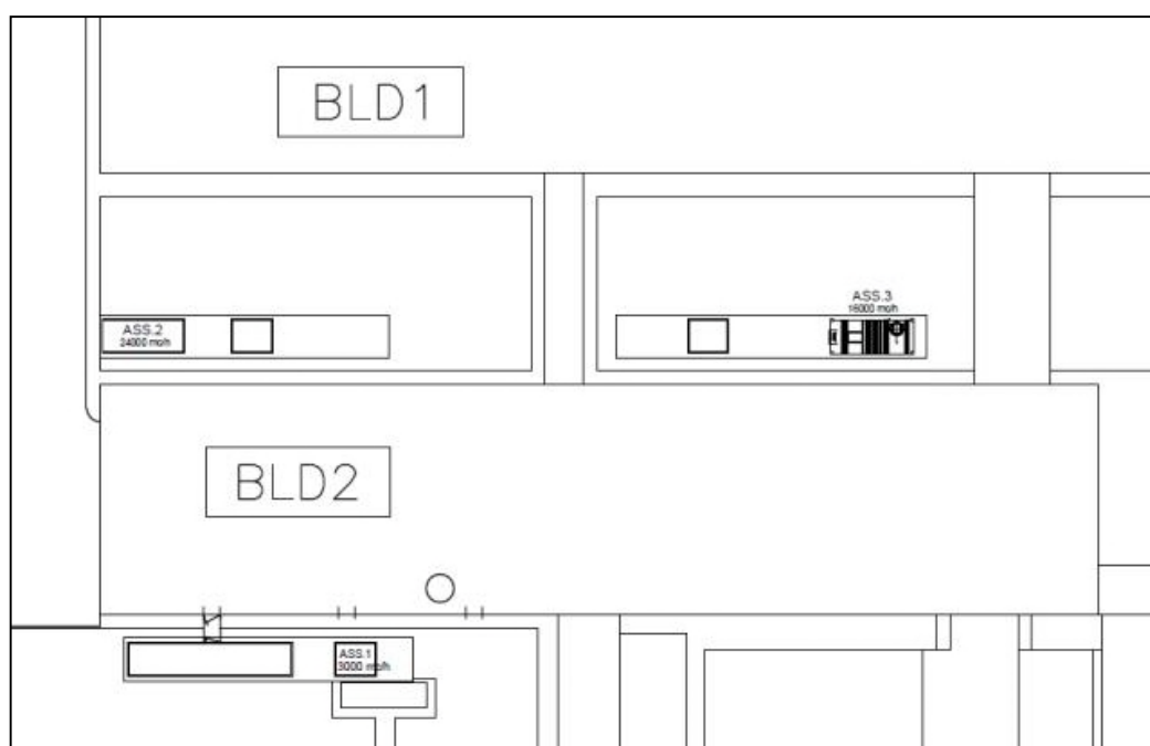
Figura 2-13 – Sistema di ventilazione di cantiere: posizionamento UTA e gruppi di filtrazione assoluta
