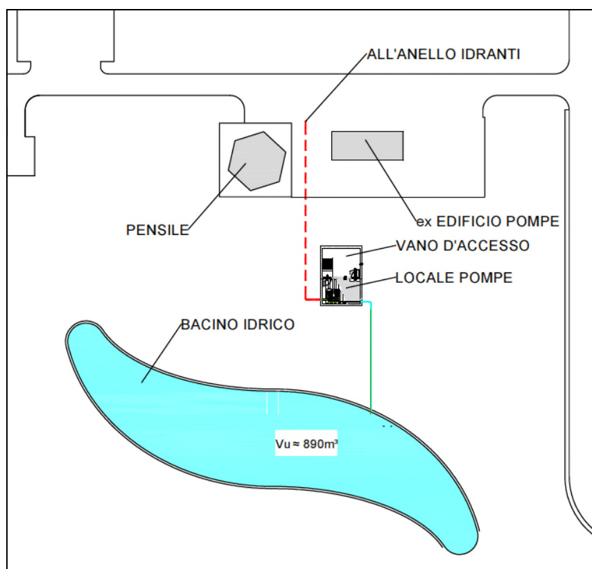
Figura 2-42 – Layout degli interventi previsti
