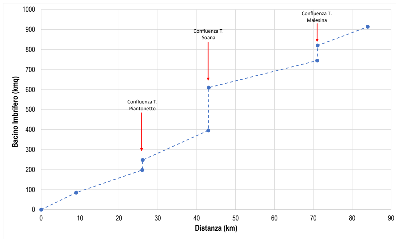
Figura 6-1: andamento superficiale bacino imbrifero in funzione della lunghezza progressiva del corso d'acqua
