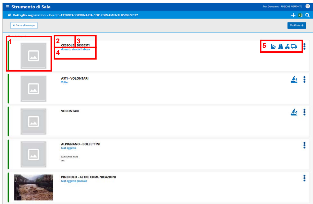
Figura 51: Pagina dettaglio segnalazioni dell'evento
