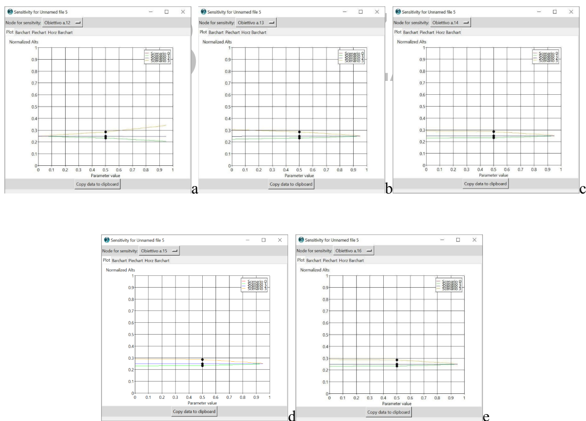
Figura 7.19. Analisi di sensitività a livello di nodo. Obiettivo A, indirizzi territoriali-pianificatori, obiettivi specifici a.12-a.16
