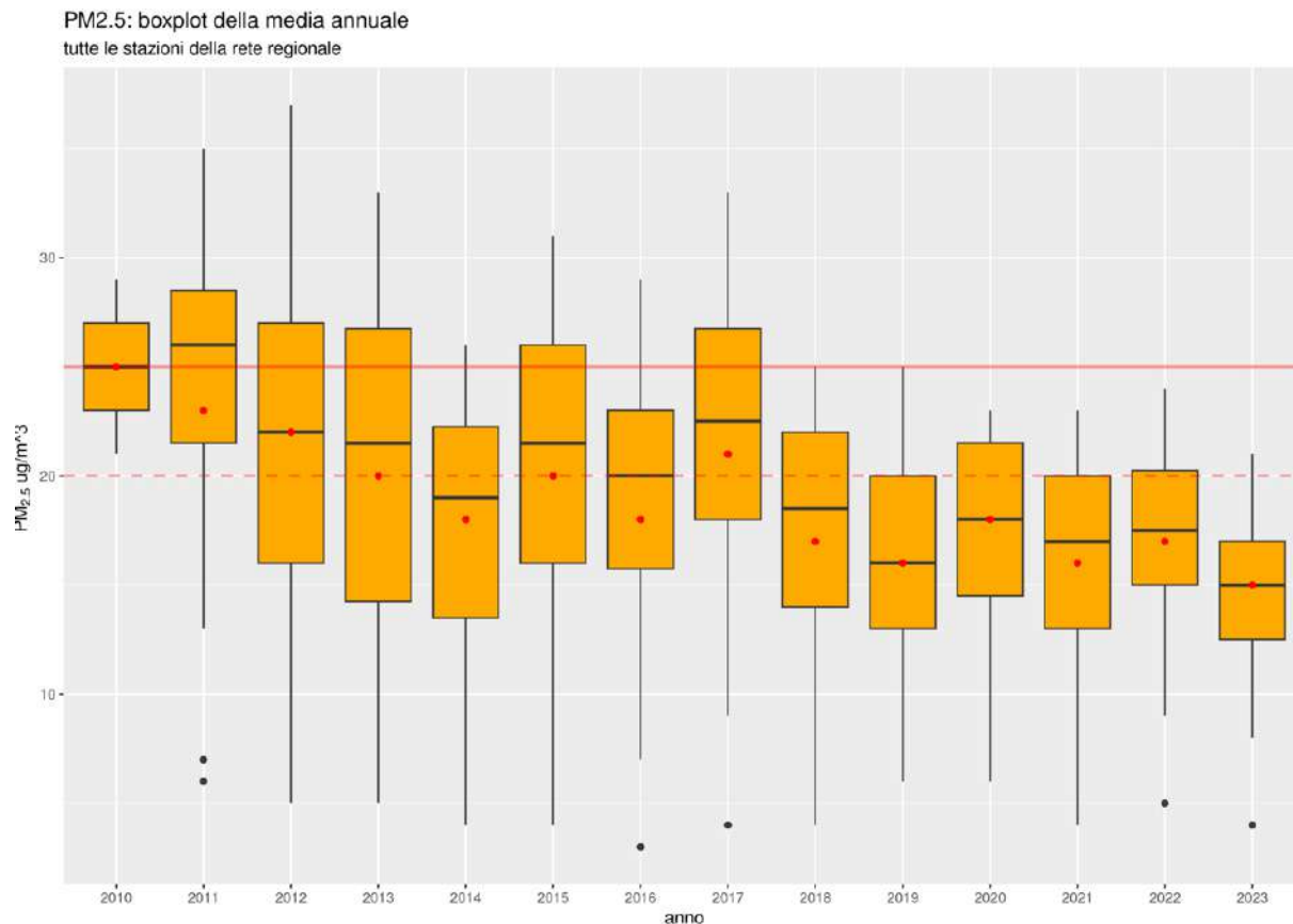
Figura 6.52: Particolato PM2.5 - Boxplot dei valori medi annuali delle stazioni della rete di monitoraggio della qualità dell'aria dal 2010 al 2023. Il pallino rosso rappresenta il valore medio di ciascun anno, la linea rossa
