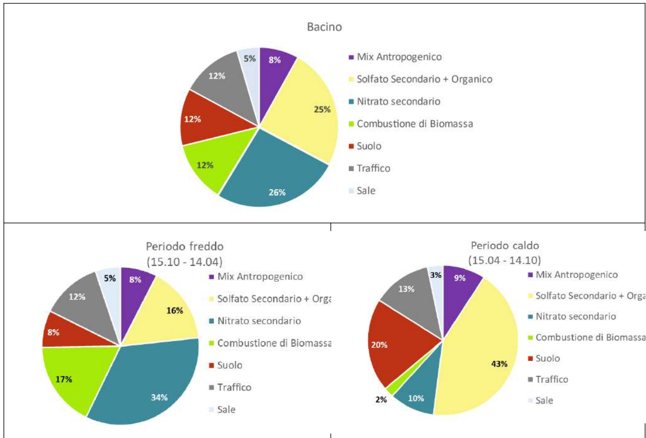
Figura 6.136: Bacino padano: contributo delle diverse sorgenti rispetto al PM10 su tutto il quadriennio (01.04.2018 - 31.03.2022) e suddiviso tra periodo caldo e periodo freddo.
