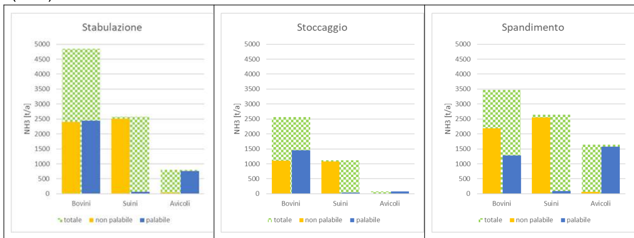
Figura 6.40: Emissioni di \text{NH}_3 relative alla gestione dei reflui azotati e stimate con l'applicativo BAT-tool, suddivise per tipologia di fase e aggregate per tipo di deiezione (IREA 2019)
