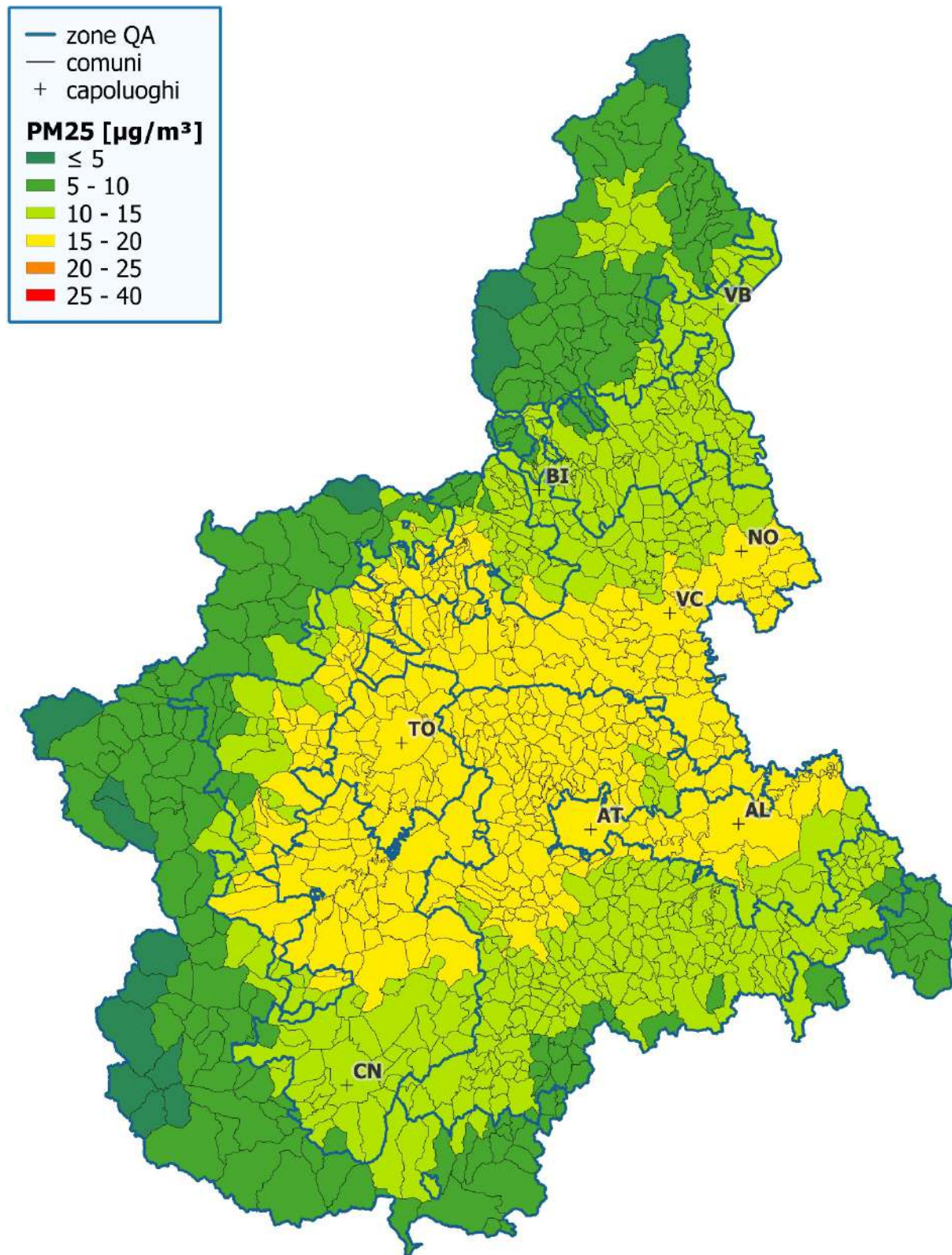
Figura 6.88: Valutazione annuale della qualità dell'aria 2023 – PM2.5: concentrazioni medie annue su base comunale
