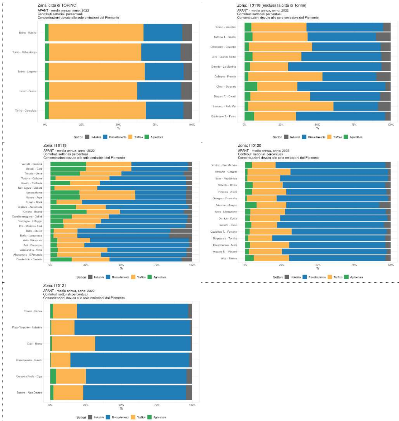
Figura 6.113: Contributo in termini di massa alle concentrazioni medie annue di particolato antropogenico primario da parte dei comparti emissivi individuati per il source apportionment
