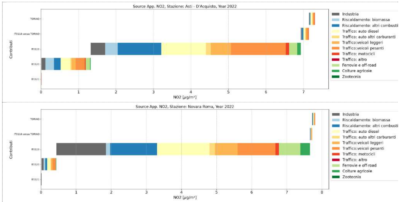
Figura 6.135: NO 2 , media annua calcolata considerando le sole emissioni del Piemonte. Contributi (in mass) dei singoli settori analizzati suddivisi per zona geografica di provenienza su alcune stazioni del SRRQA, partendo dall'alto: Torino – Rebaudengo (traffico), Torino – Lingotto (fondo), Alessandria -Volta (fondo), Asti – Acquisto (fondo), Novara – Roma (traffico).
