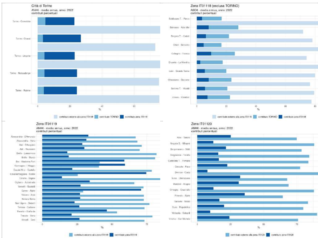
Figura 6.130: ione solfato media annua, contributo percentuale dei raggruppamenti geografici sulle singole stazioni, suddivise per zona di appartenenza. La città di Torino è stata considerata separatamente dal resto della zona IT0118. Per le stazioni della città di Torino e della restante parte della zona IT0118 vengono visualizzati i contributi di Torino, della zona IT0118 escluso Torino, ed il contributo esterno alla zona IT0118. Per tutte le altre stazioni vengono visualizzati i contributi della zona a cui afferiscono ed i contributi esterni alla zona a cui afferiscono.
