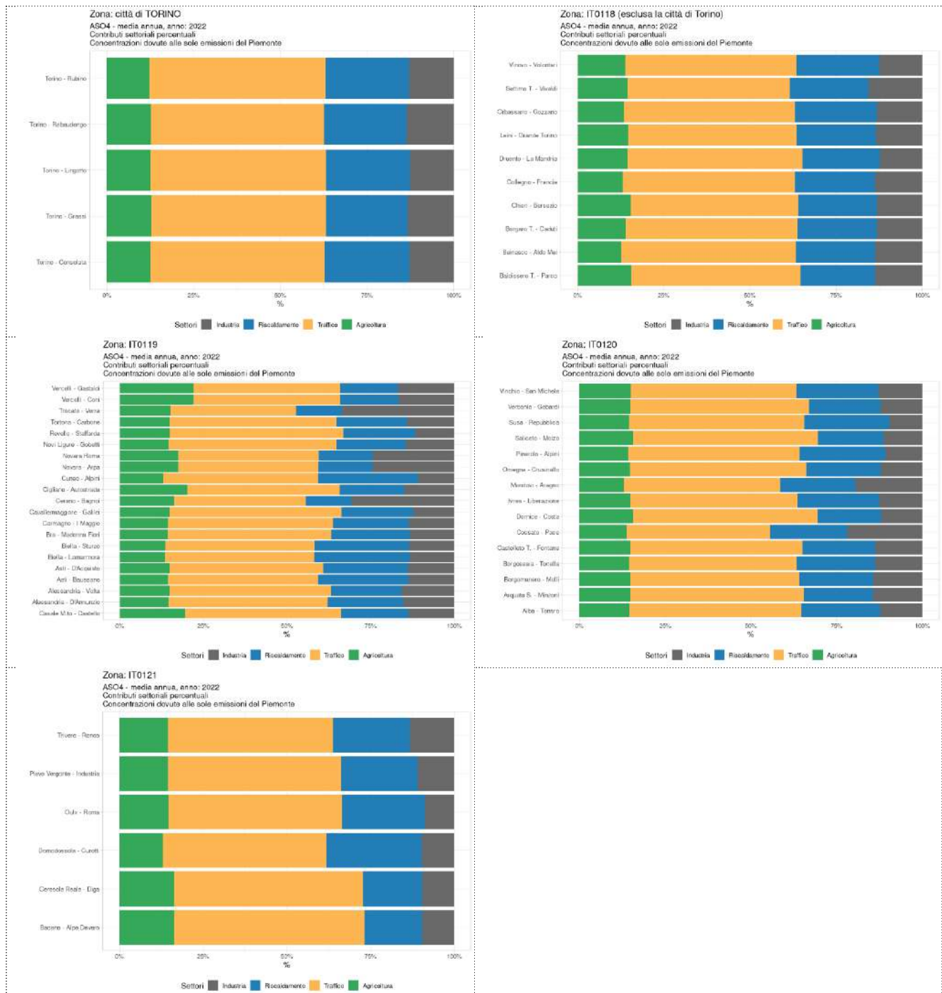
Figura 6.110: Contributo percentuale alle concentrazioni medie annue di ione solfato ( SO_4^{2-} ) presso i punti di misura di SRRQA da parte dei comparti emissivi individuati per il source apportionment. Le percentuali sono calcolate rapportando il contributo di ciascun settore alla concentrazione totale dovuta al solo contributo delle sorgenti localizzate in Piemonte
