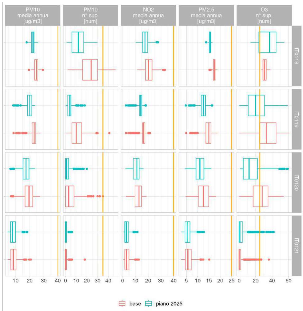
Figura 10.23: distribuzione dei valori assunti dagli indicatori (da sinistra a destra: media annua del PM10, numero di superamenti del valore limite giornaliero per il PM10, media annua di NO 2 , media annua di PM2.5, numero di superamenti del valore obiettivo a lungo termine per O 3 ) sui punti griglia afferenti alle differenti zone di qualità dell'aria (dall'alto in basso, dalla IT0118 alla IT0121). In rosa i valori associati allo scenario base, in azzurro allo scenario di Piano 2025, in arancione la linea esprime il valore limite per ciascun indicatore.
