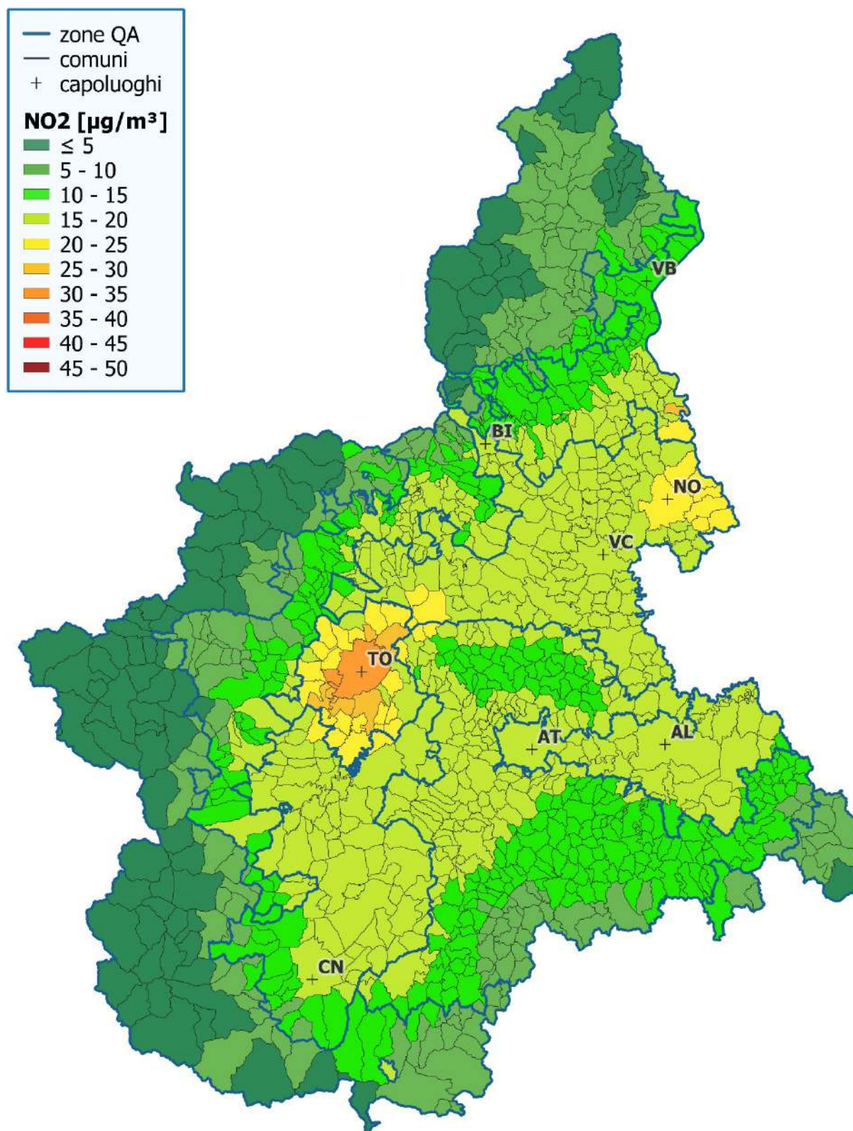
Figura 6.89: Valutazione annuale della qualità dell'aria 2023 – NO 2 : concentrazioni medie annue su base co-
