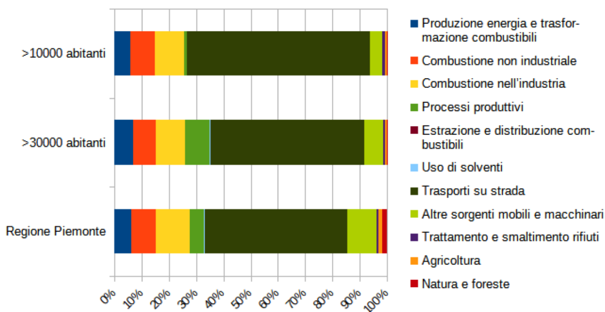
Figura 9.7 -Emissioni di NOX (t/a) per ambito territoriale di intervento (Inventario IREA 2019)
