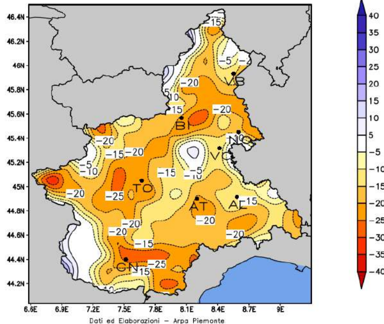
Differenza del numero medio di giorni piovosi tra 2001–2023 e 1971–2000
