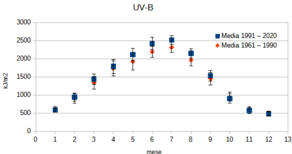
Figura 6.9: Andamento della radiazione UV-b incidente (kJ/m²) sul Piemonte da ERA5 per i periodi climatici 1961-1990 e 1991-2020.
