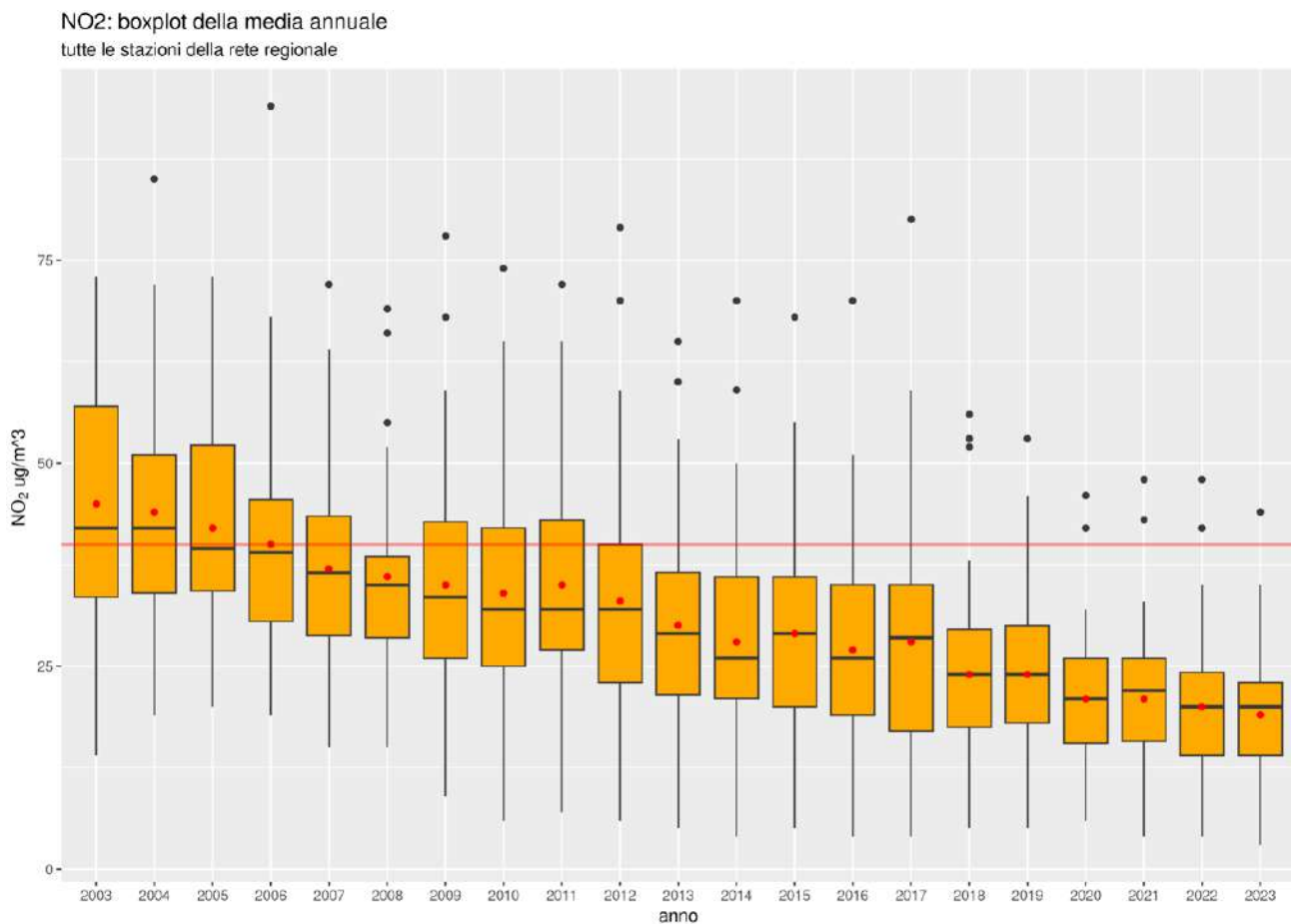
Figura 6.56: Biossido di azoto - boxplot dei valori medi annuali delle stazioni della rete di monitoraggio della qualità dell'aria dal 2003 al 2023. Il pallino rosso rappresenta il valore medio di ciascun anno, la linea rossa continua il limite stabilito dal D.Lgs. 155/2010 per la media annua.
