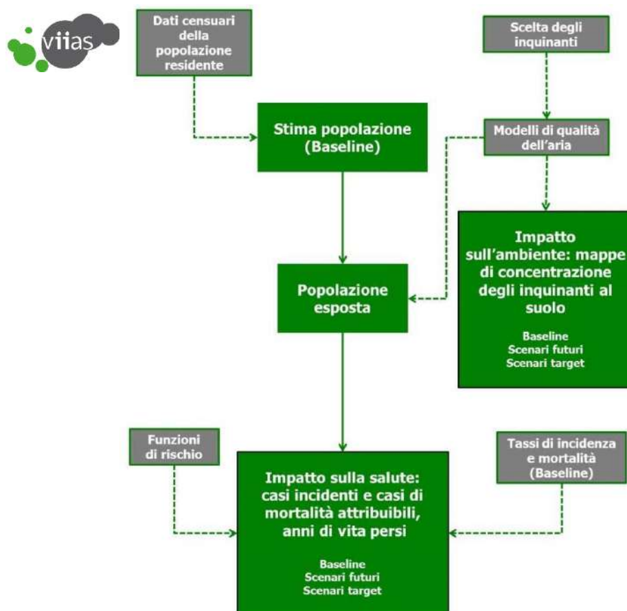
Figura 5: Schema della valutazione dell'impatto dell'inquinamento atmosferico sull'ambiente e sulla salute umana, progetto CCM VIIAS
