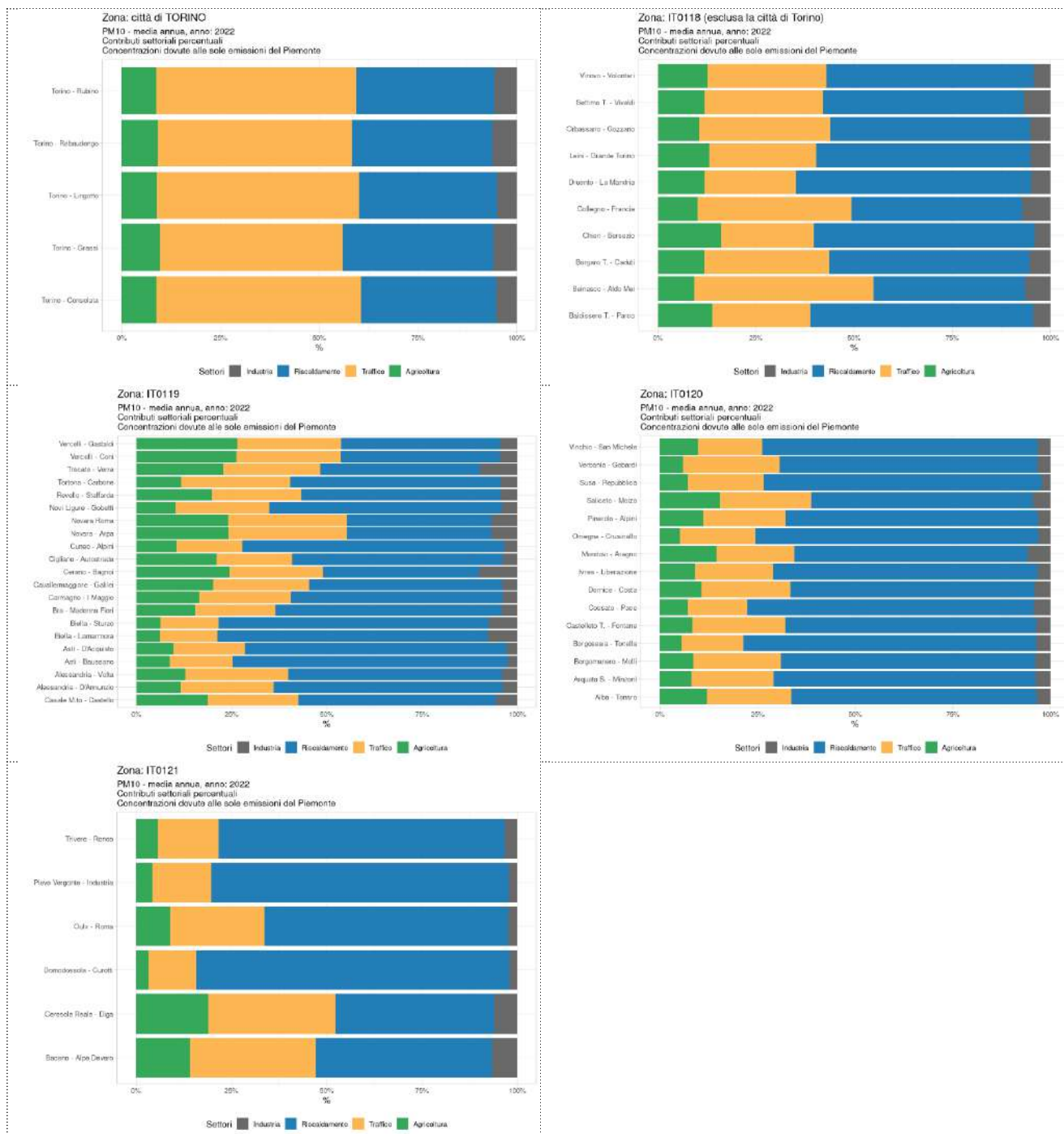
Figura 6.106: Contributo percentuale alle concentrazioni medie annue di particolato PM10 presso i punti di misura di SRRQA da parte dei comparti emissivi individuati per il source apportionment. Le percentuali sono calcolate rapportando il contributo di ciascun settore alla concentrazione totale dovuta al solo contributo delle sorgenti localizzate in Piemonte.
