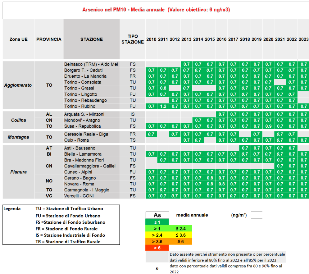
Figura 6.75: Arsenico - concentrazioni medie annue misurate presso le stazioni della rete regionale nel periodo dal 2010 al 2023
