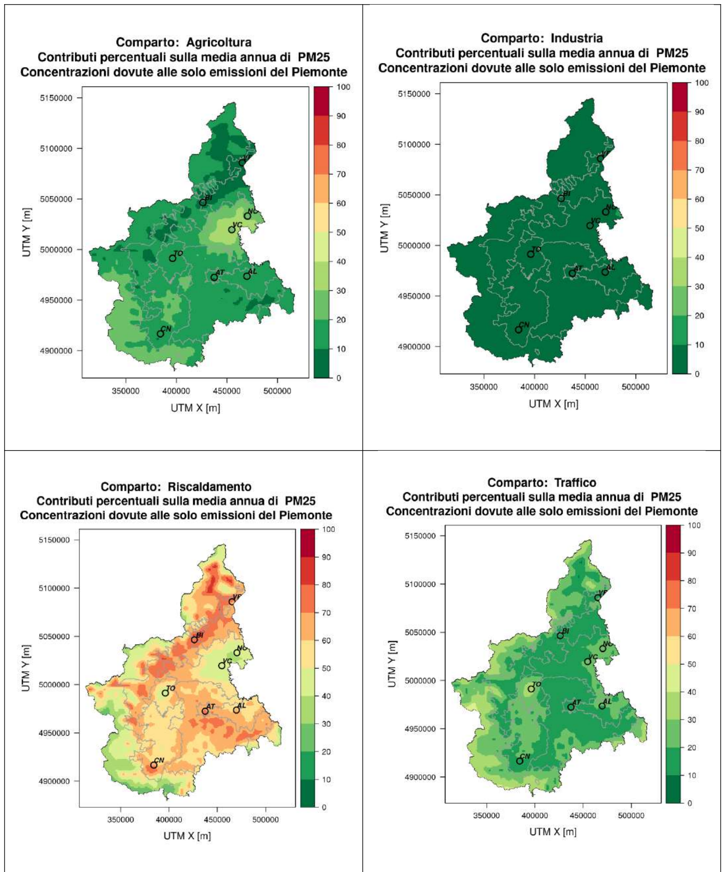
Figura 6.121: Distribuzione spaziale del contributo percentuale alle concentrazioni medie annue di particolato PM2.5 da parte dei comparti emissivi indagati con il source apportionment.
