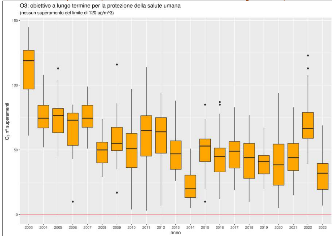
Figura 6.63: Ozono: boxplot dei superamenti annuali del valore obiettivo a lungo termine per le stazioni della
