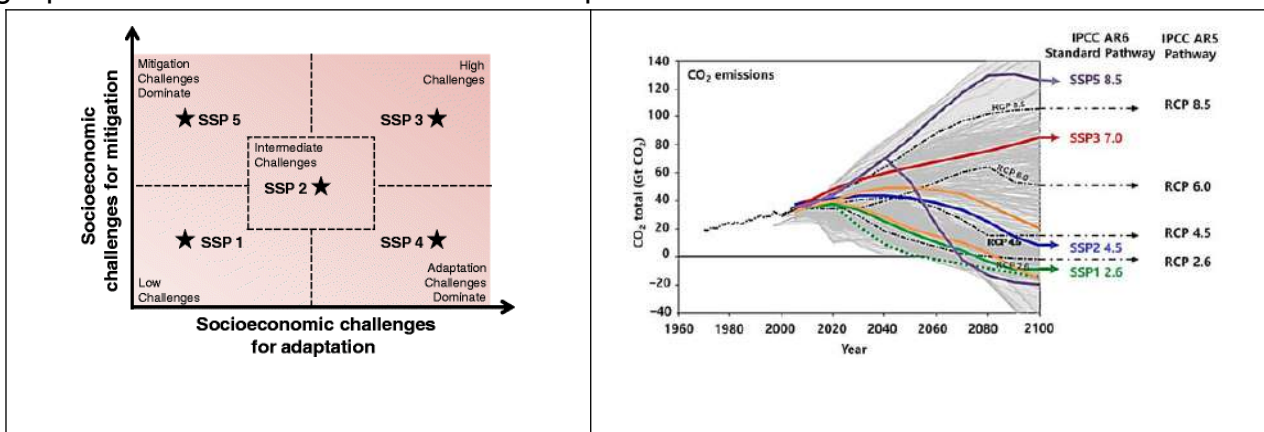
Figura 6.19: A sinistra i nuovi scenari SSP visualizzati nel "challenges to mitigation/adaptation space". A destra il confronto tra i due tipi di scenari.
