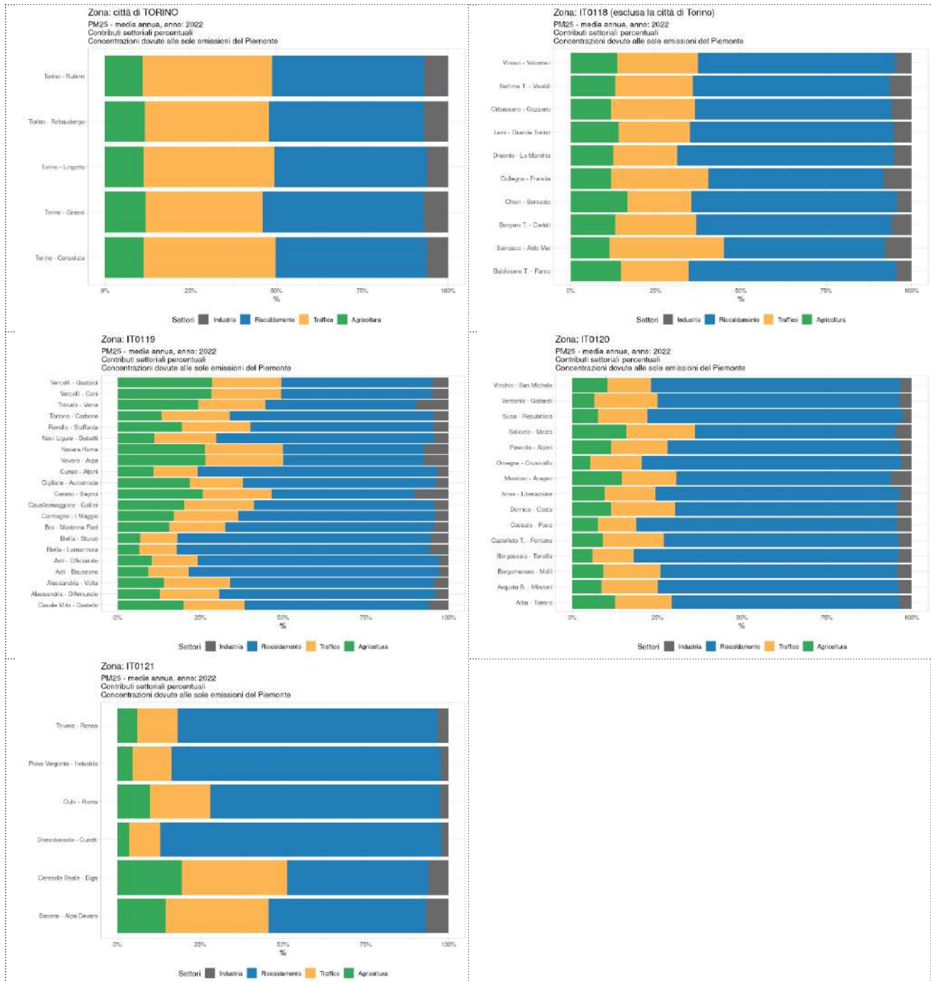
Figura 6.107: Contributo percentuale alle concentrazioni medie annue di particolato PM2.5 presso i punti di misura di SRRQA da parte dei comparti emissivi individuati per il source apportionment. Le percentuali sono calcolate rapportando il contributo di ciascun settore alla concentrazione totale dovuta al solo contributo delle sorgenti localizzate in Piemonte
