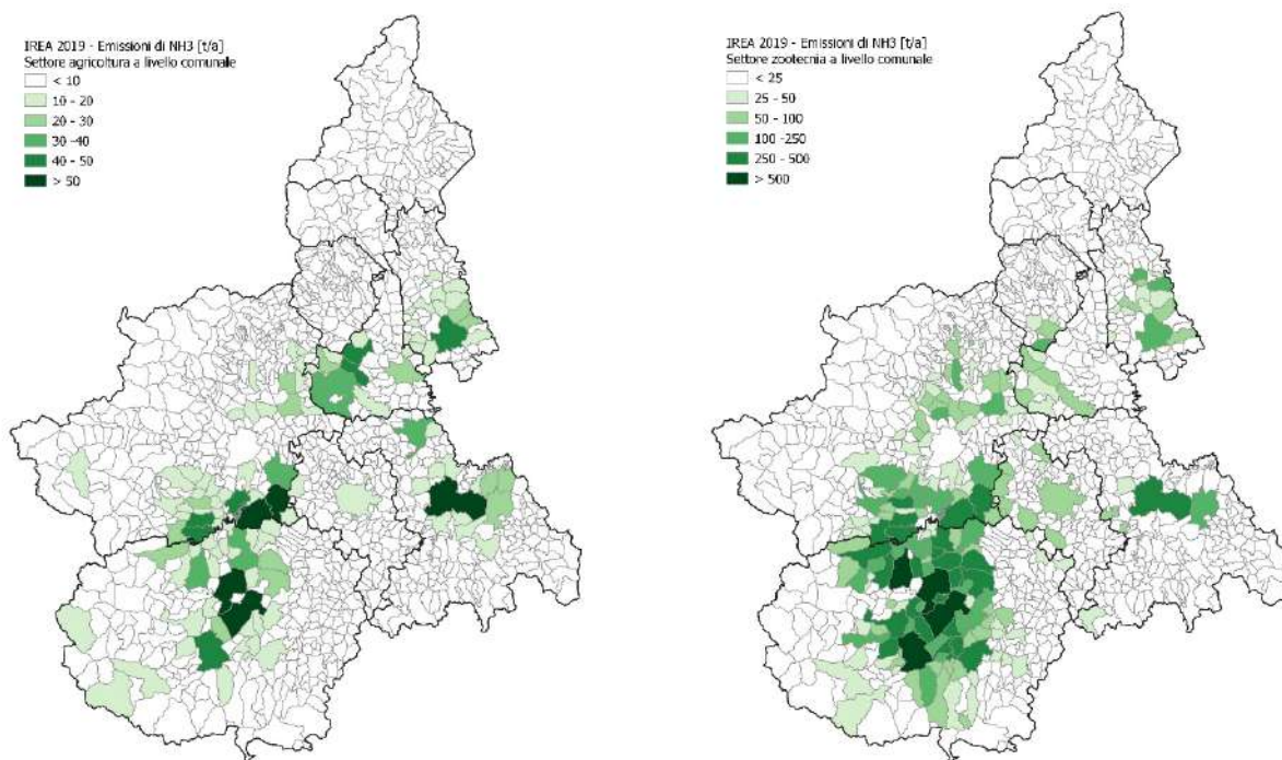
Figura 6.39: Distribuzione sul territorio regionale delle emissioni comunali di ammoniaca legate alle colture agricole a sinistra e alla zootecnia a destra - IREA 2019
