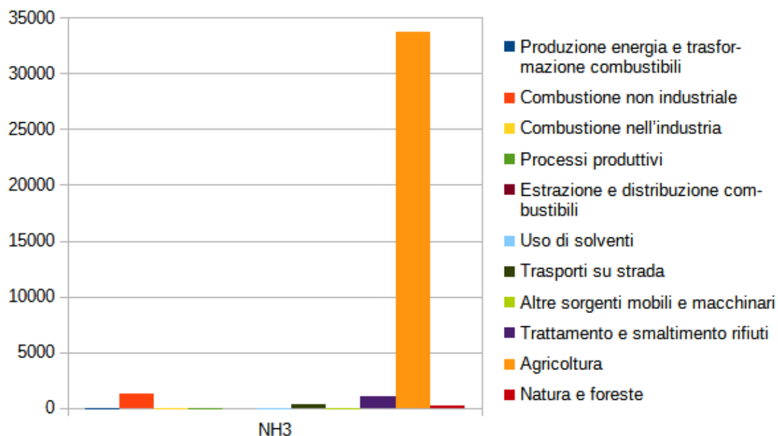
Figura 9.3 - Emissioni di NH3 (t/a) per macrosettore (Inventario IREA 2019)
