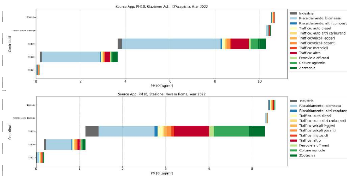
Figura 6.133: PM10, media annua calcolata considerando le sole emissioni del Piemonte. Contributi (in mass) dei singoli settori analizzati suddivisi per zona geografica di provenienza su alcune stazioni del SRR-QA, partendo dall'alto: Torino – Rebaudengo (traffico), Torino – Lingotto (fondo), Alessandria -Volta (fondo), Asti – Acquisto (fondo), Novara – Roma (traffico).
