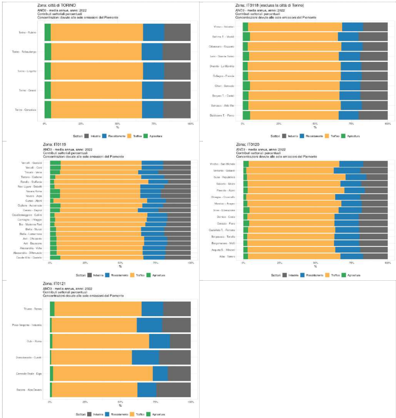
Figura 6.109: Contributo percentuale alle concentrazioni medie annue di ione nitrato ( \text{NO}_3^- ) presso i punti di misura di SRRQA da parte dei comparti emissivi individuati per il source apportionment. Le percentuali sono calcolate rapportando il contributo di ciascun settore alla concentrazione totale dovuta al solo contributo delle sorgenti localizzate in Piemonte
