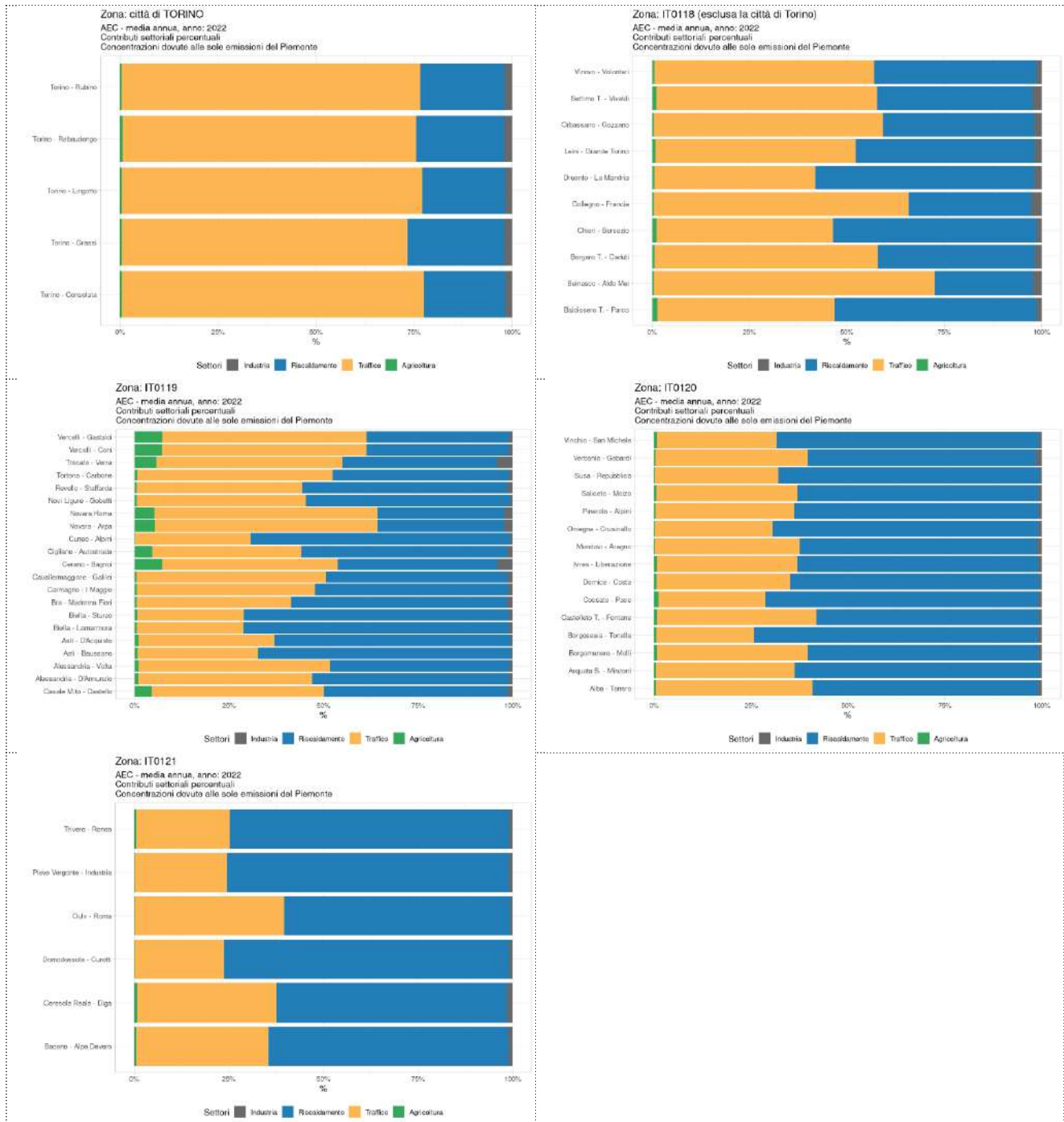
Figura 6.112: Contributo in termini di massa alle concentrazioni medie annue di carbonio elementare (EC) da parte dei comparti emissivi individuati per il source apportionment.
