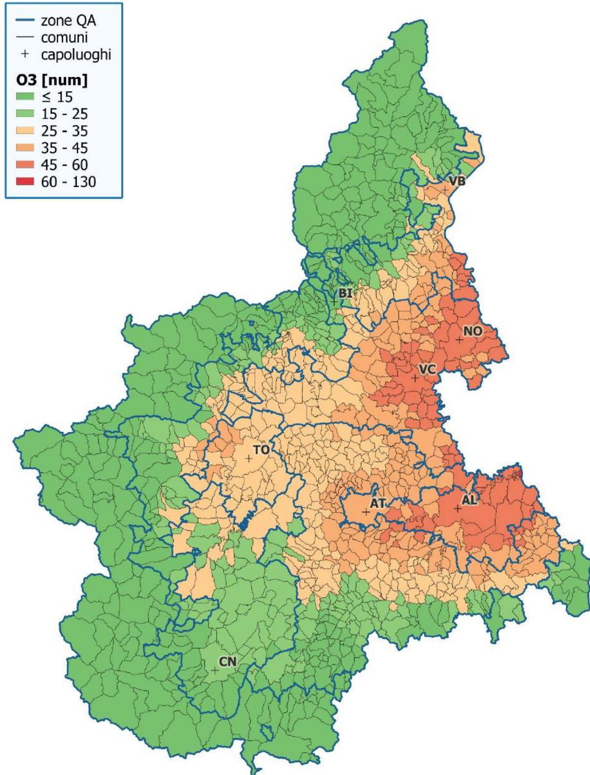
Figura 6.90: Valutazione annuale della qualità dell'aria 2023 – O 3 : numero di superamenti del valore obiettivo
