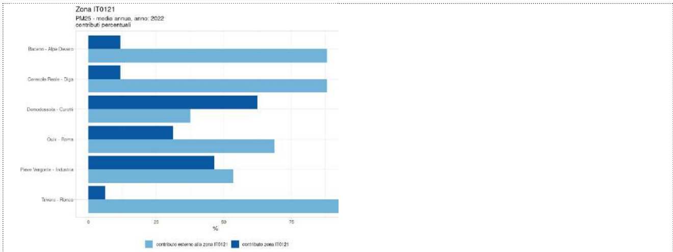
Figura 6.127: PM2.5 media annua, contributo percentuale dei raggruppamenti geografici sulle singole stazioni, suddivise per zona di appartenenza. La città di Torino è stata considerata separatamente dal resto della zona IT0118. Per le stazioni della città di Torino e della restante parte della zona IT0118 vengono visualizzati i contributi di Torino, della zona IT0118 escluso Torino, ed il contributo esterno alla zona IT0118. Per tutte le altre stazioni vengono visualizzati i contributi della zona a cui afferiscono ed i contributi esterni alla zona cui afferiscono
