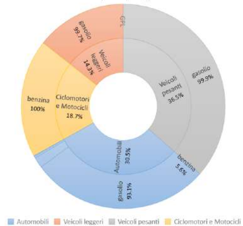
Emissioni PM10 suddivise per tipologia di veicolo e carburanti
