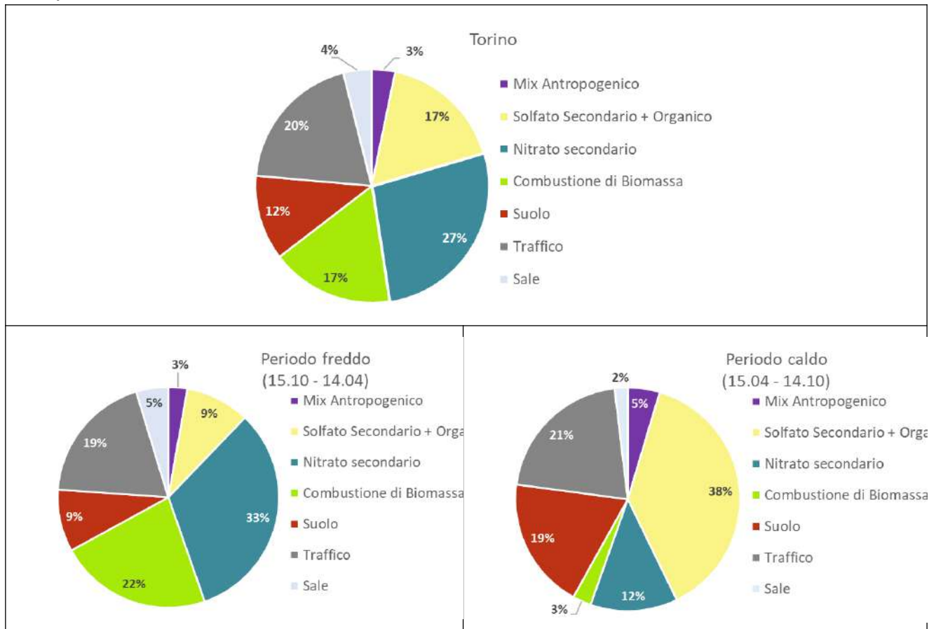
Figura 6.137: Torino: contributo delle diverse sorgenti rispetto al PM10 sull'intero periodo dal 15.09.2018 al 31.03.2022 e suddiviso tra periodo caldo e periodo freddo.
