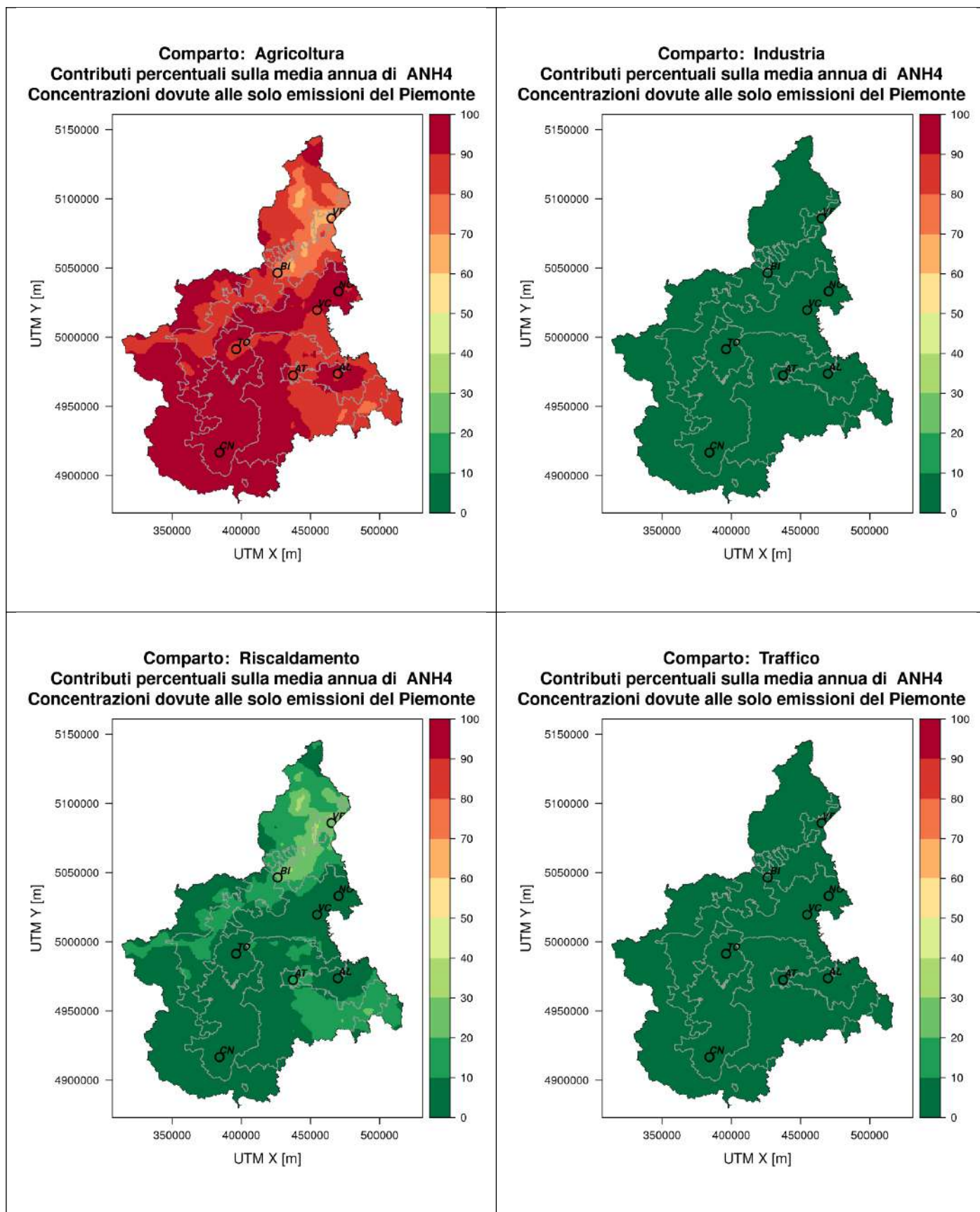
Figura 6.125: Distribuzione spaziale del contributo percentuale alle concentrazioni medie annue di ione ammonio da parte dei comparti emissivi indagati con il source apportionment
