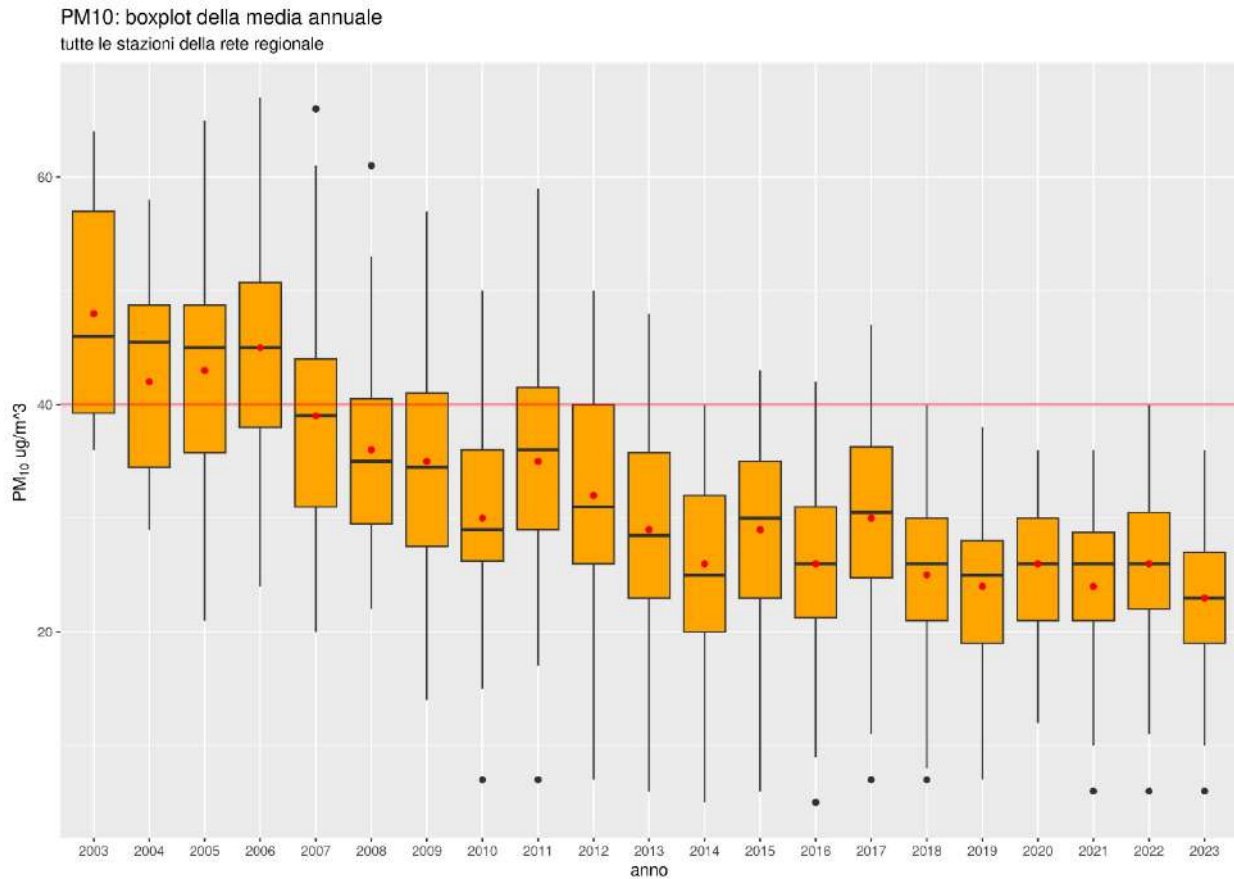
Figura 6.44: PM10 - boxplot delle concentrazioni medie annuali misurate presso le stazioni della rete di monitoraggio della qualità dell'aria dal 2003 al 2023. Il pallino rosso rappresenta il valore medio di ciascun anno, la linea rossa il limite stabilito dal D.Lgs 155/2010 per la media annua.
