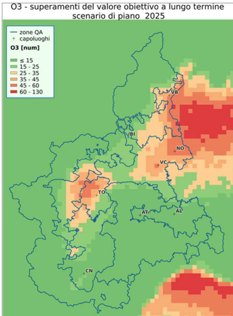
Figura 10.22: mappe di concentrazione sul dominio di simulazione nello scenario di Piano 2025: O 3 , numero di giorni di superamento del valore obiettivo di 120 mg/m 3 per la massima media mobile su otto ore.
