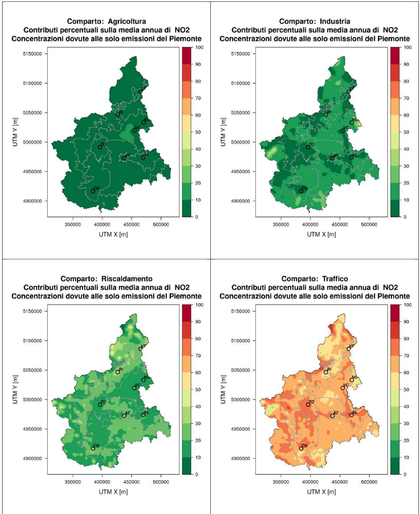
Figura 6.122: Distribuzione spaziale del contributo percentuale alle concentrazioni medie annue di biossido di azoto da parte dei comparti emissivi indagati con il source apportionment.
