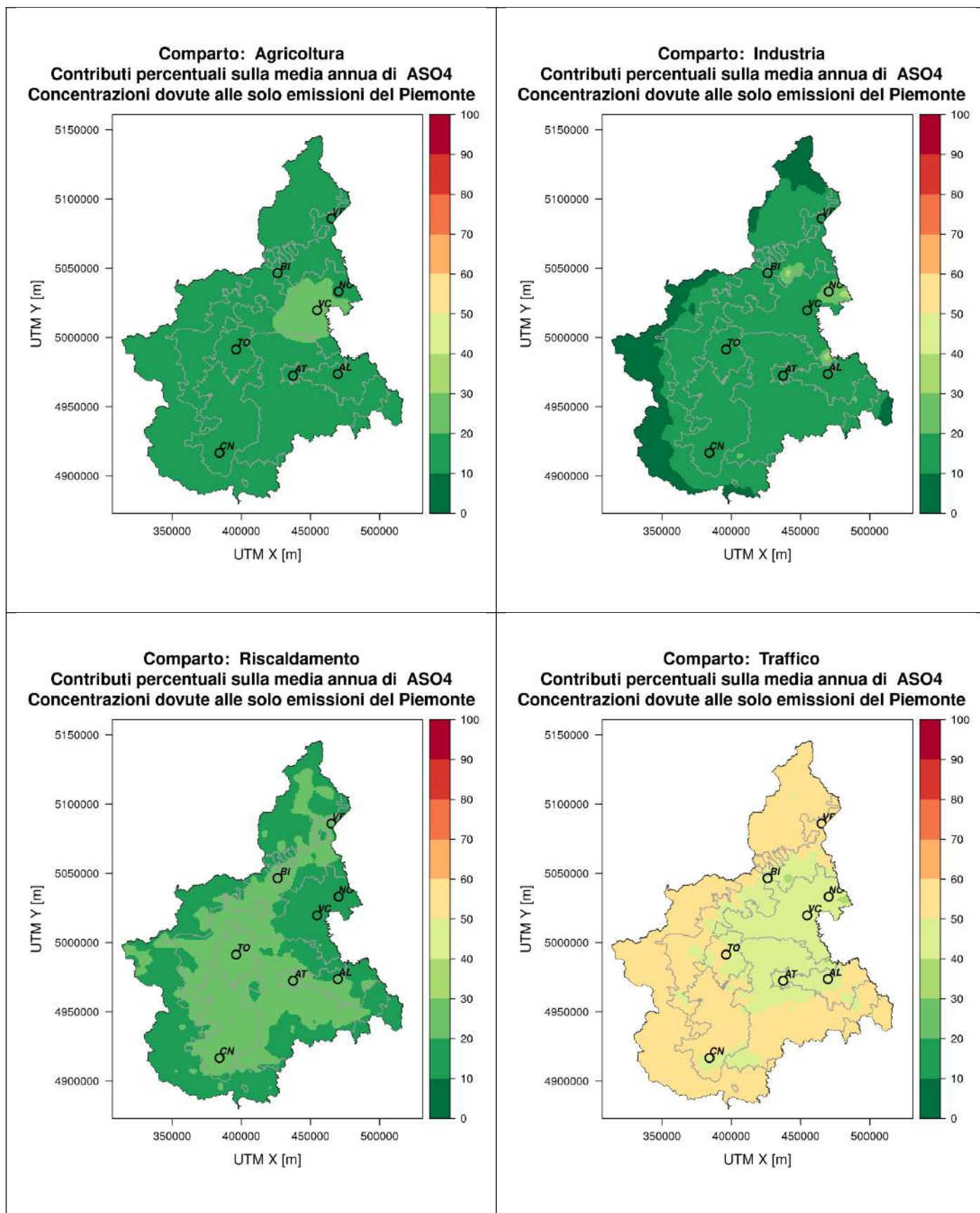
Figura 6.124: Distribuzione spaziale del contributo percentuale alle concentrazioni medie annue di ione solfato da parte dei comparti emissivi indagati con il source apportionment
