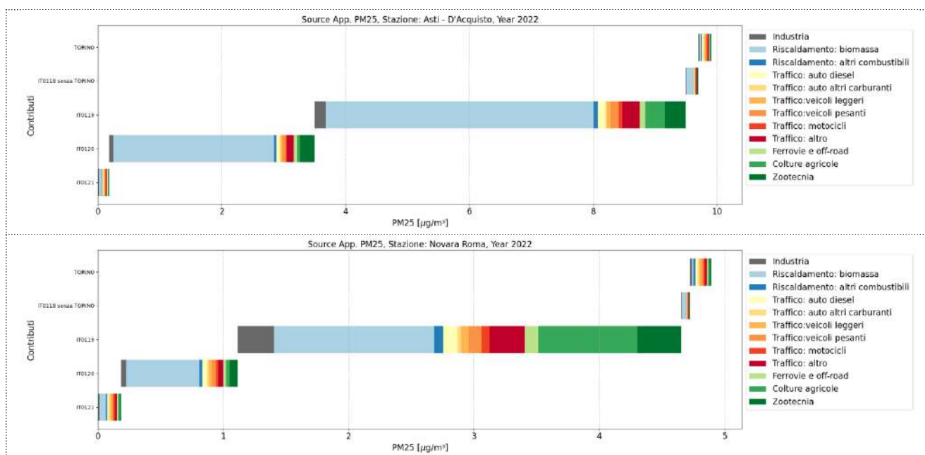
Figura 6.134: PM2.5, media annua calcolata considerando le sole emissioni del Piemonte. Contributi (in mass) dei singoli settori analizzati suddivisi per zona geografica di provenienza su alcune stazioni del SRR-QA, partendo dall'alto: Torino – Rebaudengo (traffico), Torino – Lingotto (fondo), Alessandria -Volta (fondo), Asti – Acquisto (fondo), Novara – Roma (traffico).
