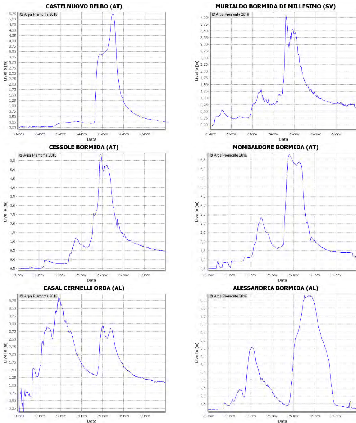
Figura 56. Idrogrammi delle stazioni idrometriche che hanno registrato i colmi più significativi.
