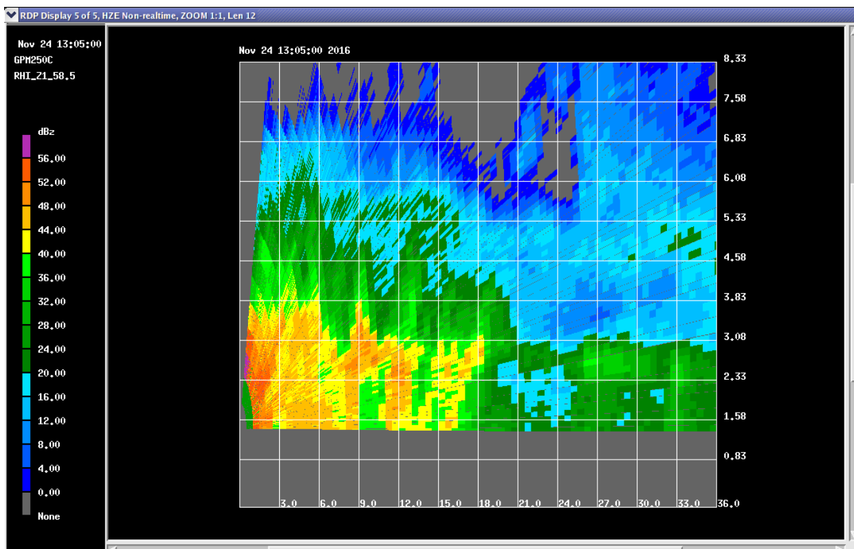
Figura 34. Sezione verticale effettuata dal radar di Monte Settepani in direzione Nord-Est. Si notano valori estremamente elevati (maggiori di 56 dBZ) in prossimità del radar, a quote comprese tra 2.3 e 3 km.
