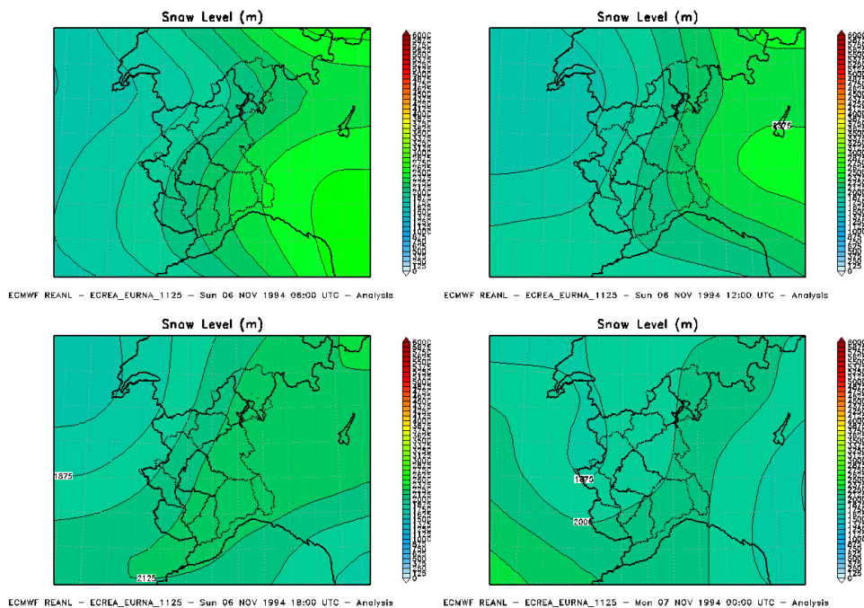
Figura 102. Quota neve tra il 6 novembre 1994 06UTC ed il 7 novembre 1994 00UTC
