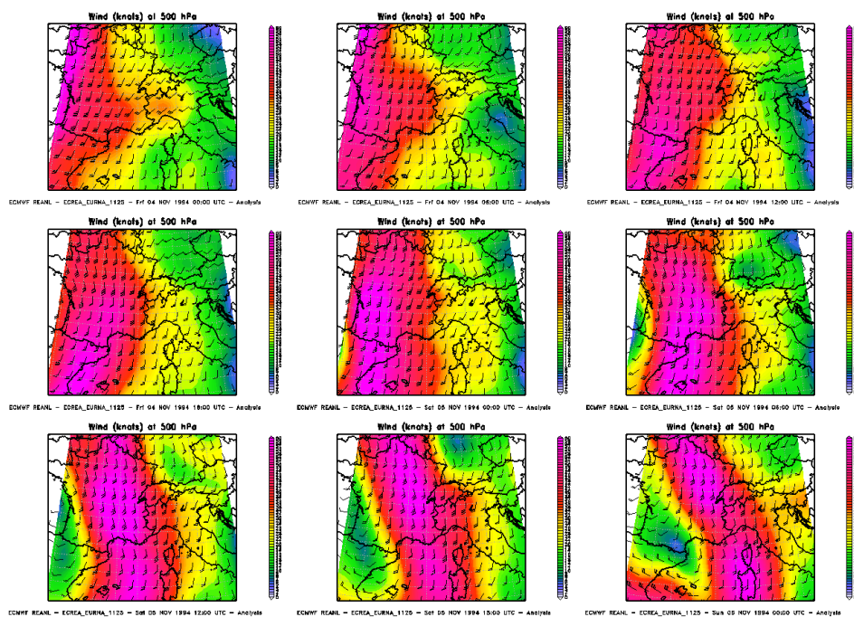
Figura 81. Venti a 500hPa dal 4 novembre 1994 00UTC al 6 novembre 1994 00UTC
