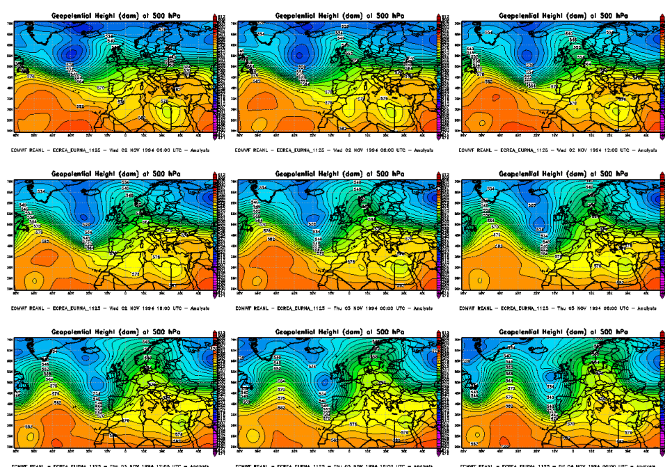
Figura 74. Mappe di analisi di Altezza Geopotenziale a 500hPa dal 2 novembre 1994 00UTC al 4 novembre 1994 00UTC
