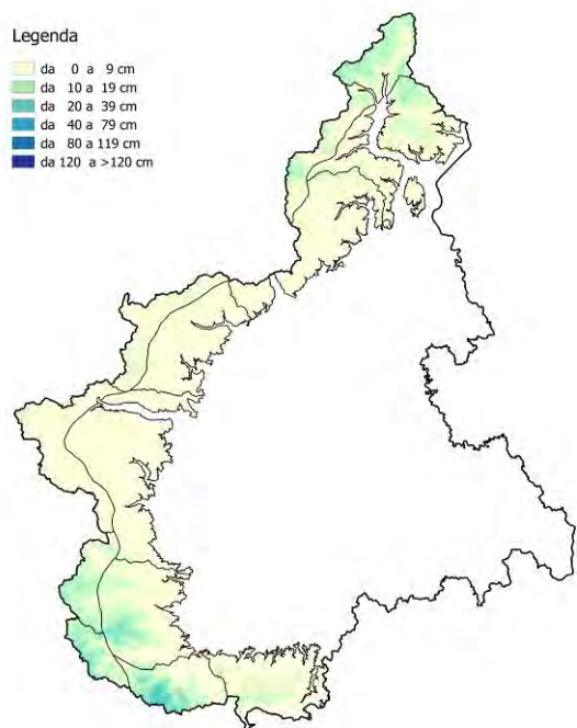
Figura 44. Neve fresca registrata il 21 novembre
