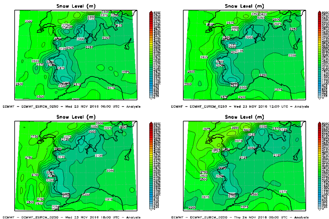
Figura 27. Analisi della quota neve per la giornata del 23 novembre 2016
