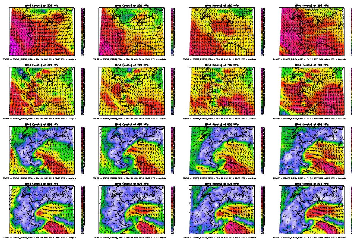
Figura 30. Analisi dei venti alle quote sinottiche principali nella giornata del 24 novembre 2016
