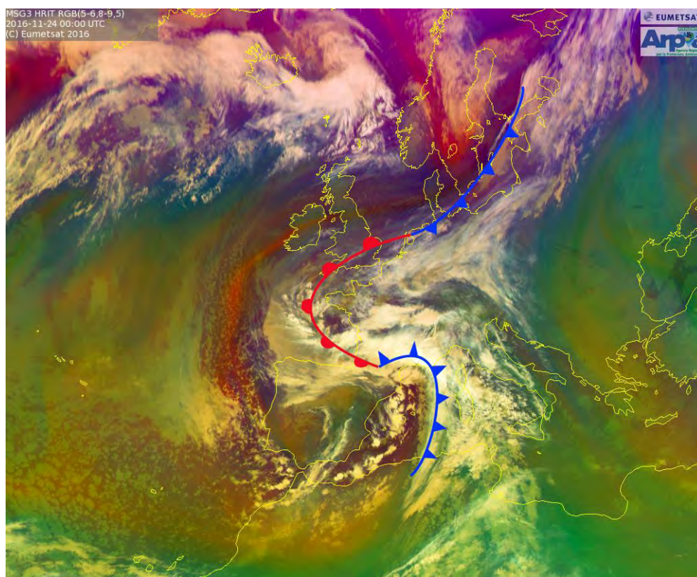
Figura 21. Immagine Meteosat (airmass, composizione di bande di infrarosso) alle 00UTC del 24 novembre 2016 con mappa dei fronti
