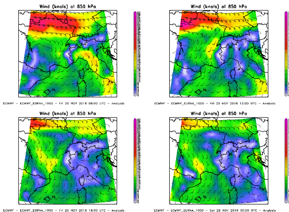
Figura 97. Venti a 850hPa dal 25 novembre 2016 06UTC al 26 novembre 2016 00UTC
