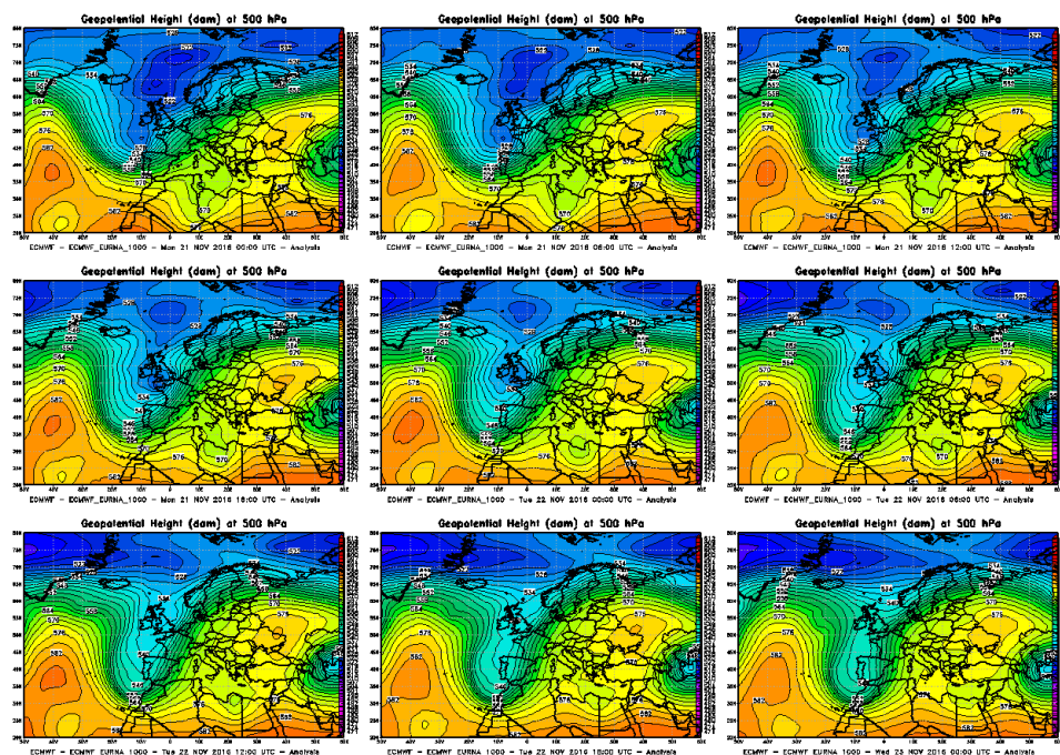
Figura 77. Mappe di analisi di Altezza Geopotenziale a 500hPa dal 21 novembre 2016 00UTC al 23 novembre 2016 00UTC
