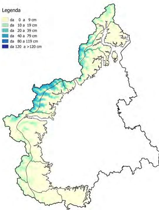
Figura 46. Neve fresca registrata il 23 novembre
