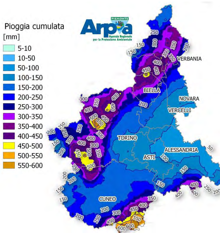
Figura 106. Precipitazioni cumulate dei 3 differenti eventi alluvionali
