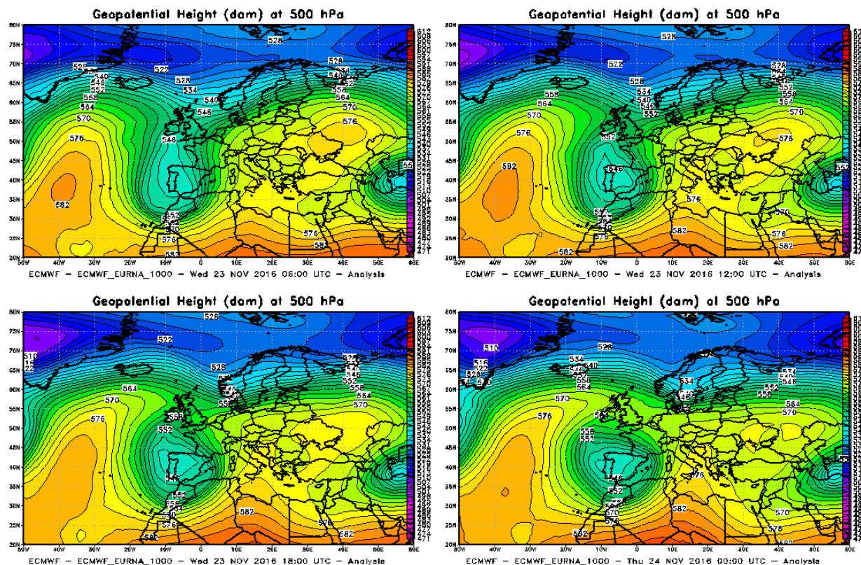
Figura 20. Analisi dell'altezza di geopotenziale a 500hPa nella giornata del 23 novembre 2016
