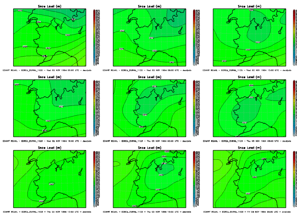
Figura 100. Quota neve tra il 2 novembre 1994 00UTC ed il 4 novembre 1994 00UTC
