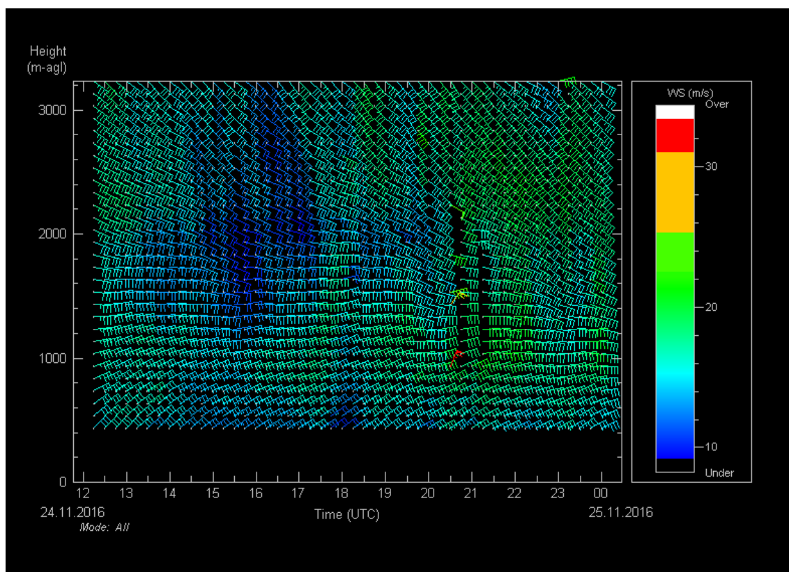
Figura 32. Osservazioni da remoto del vento fino a 3000 metri mediante il wind profiler posizionato a Torino in corso Stati Uniti nella giornata del 24 novembre 2016
