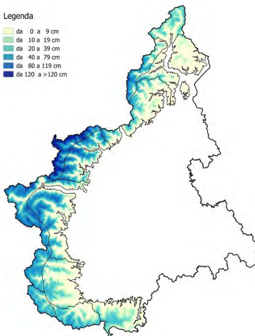
Figura 48. Neve fresca registrata il 25 novembre
