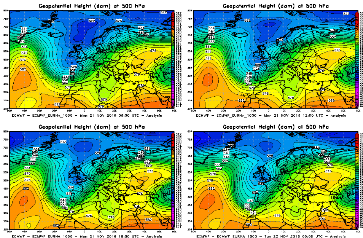
Figura 5. Analisi dell'altezza di geopotenziale a 500hPa nella giornata del 21 novembre 2016
