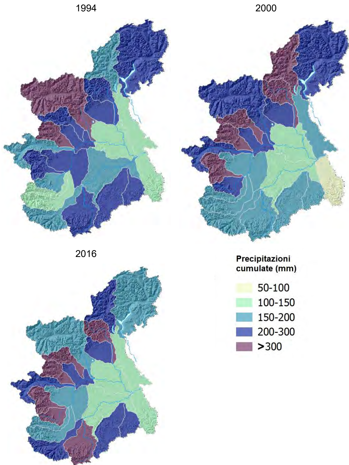
Figura 107. Precipitazioni medie areali per bacino idrografico dei 3 eventi
