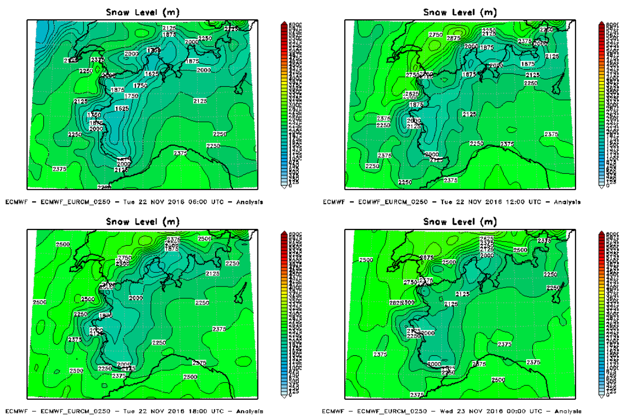
Figura 19. Analisi della quota neve per la giornata del 22 novembre 2016
