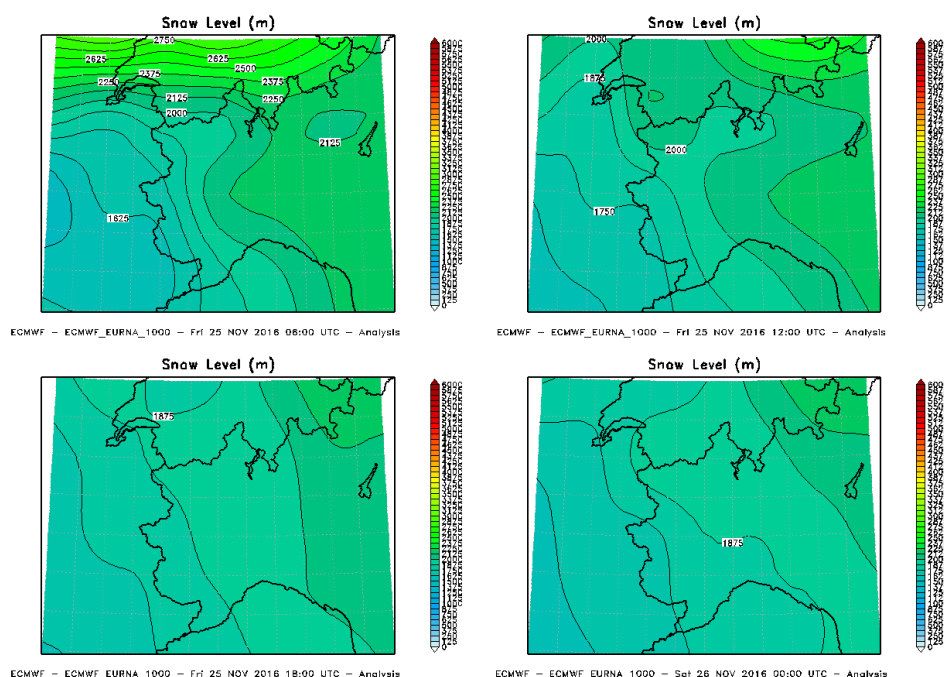
Figura 105. Quota neve dal 25 novembre 2016 06UTC al 26 novembre 2016 00UTC
