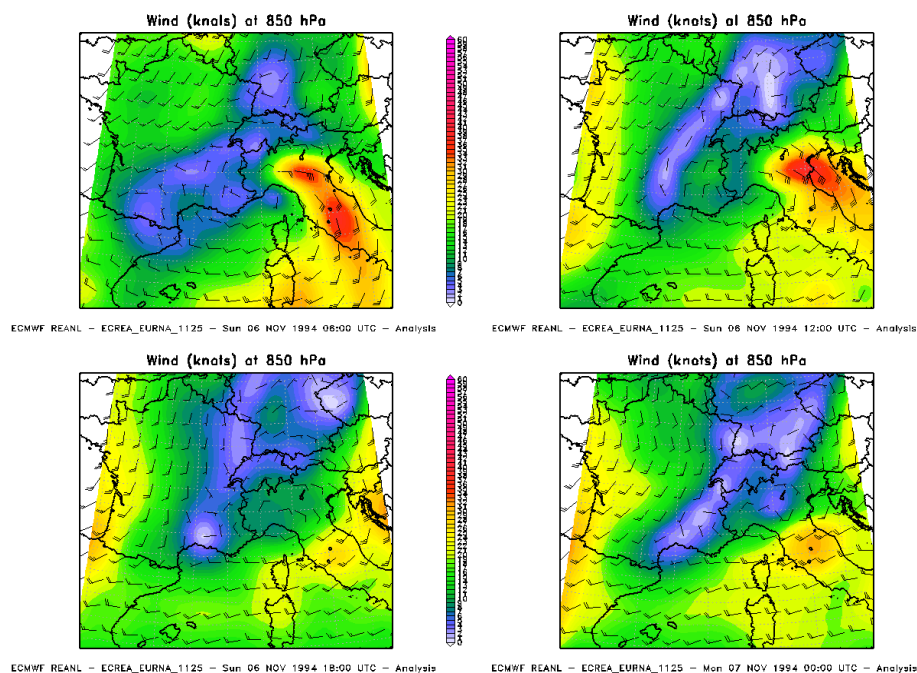
Figura 88. Venti a 850hPa dal 6 novembre 1994 06UTC al 7 novembre 1994 00UTC
