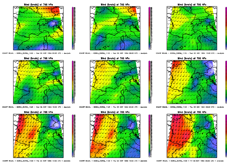
Figura 83. Venti a 700hPa dal 2 novembre 1994 00UTC al 4 novembre 1994 00UTC
