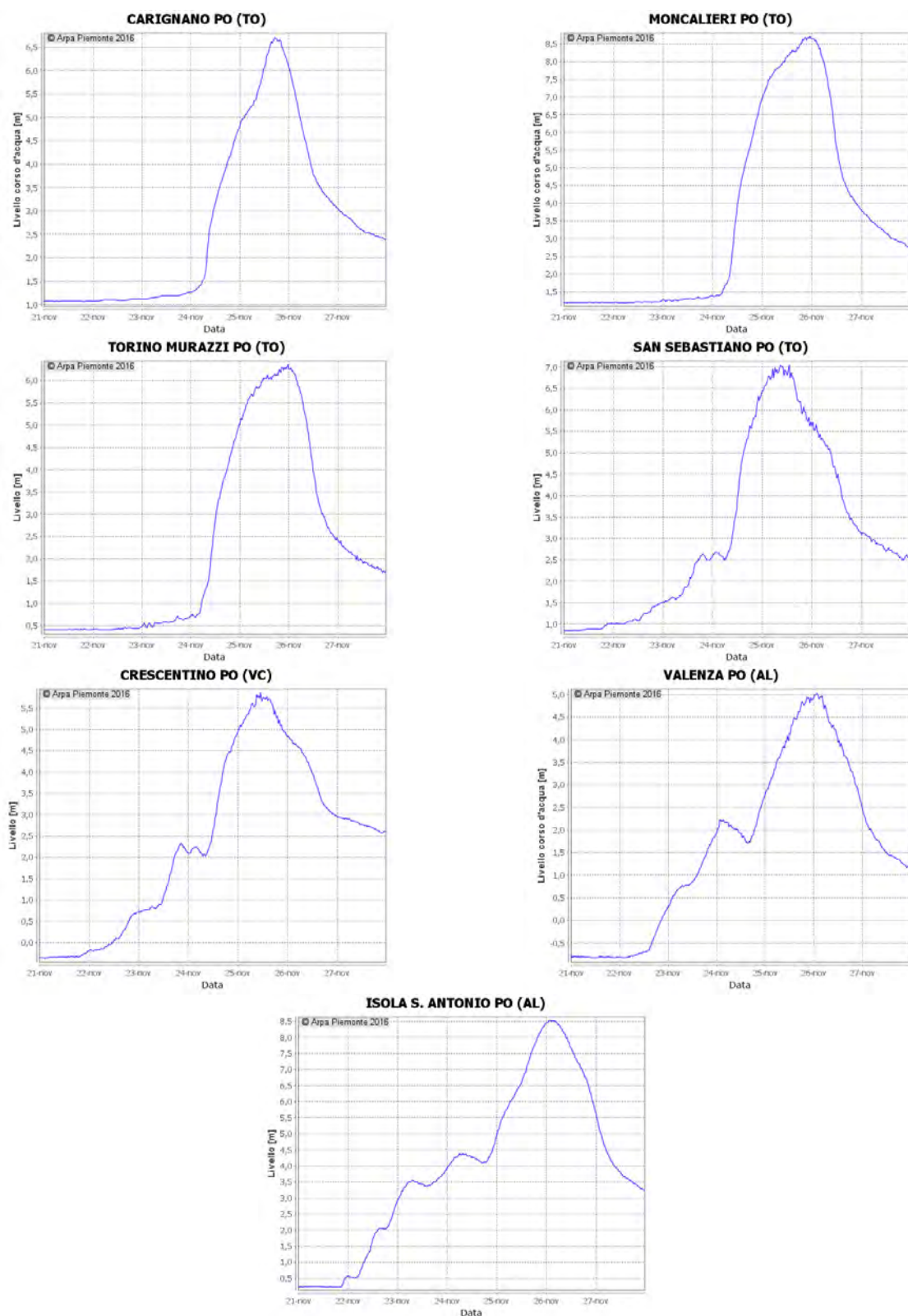
Figura 58. Idrogrammi delle stazioni idrometriche del Po.
