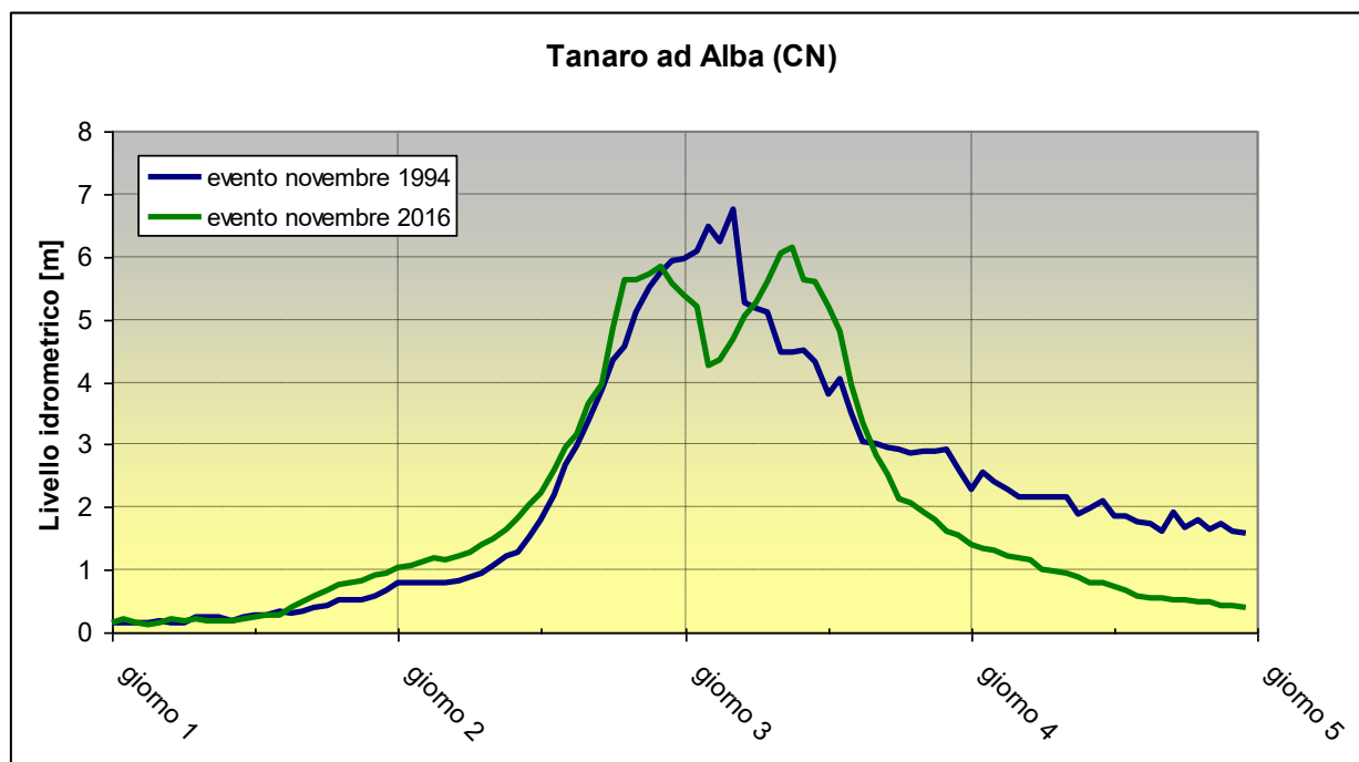
Figura 111. Confronto tra gli idrogrammi del Tanaro ad Alba (CN) registrati a novembre 1994 e a novembre 2016
