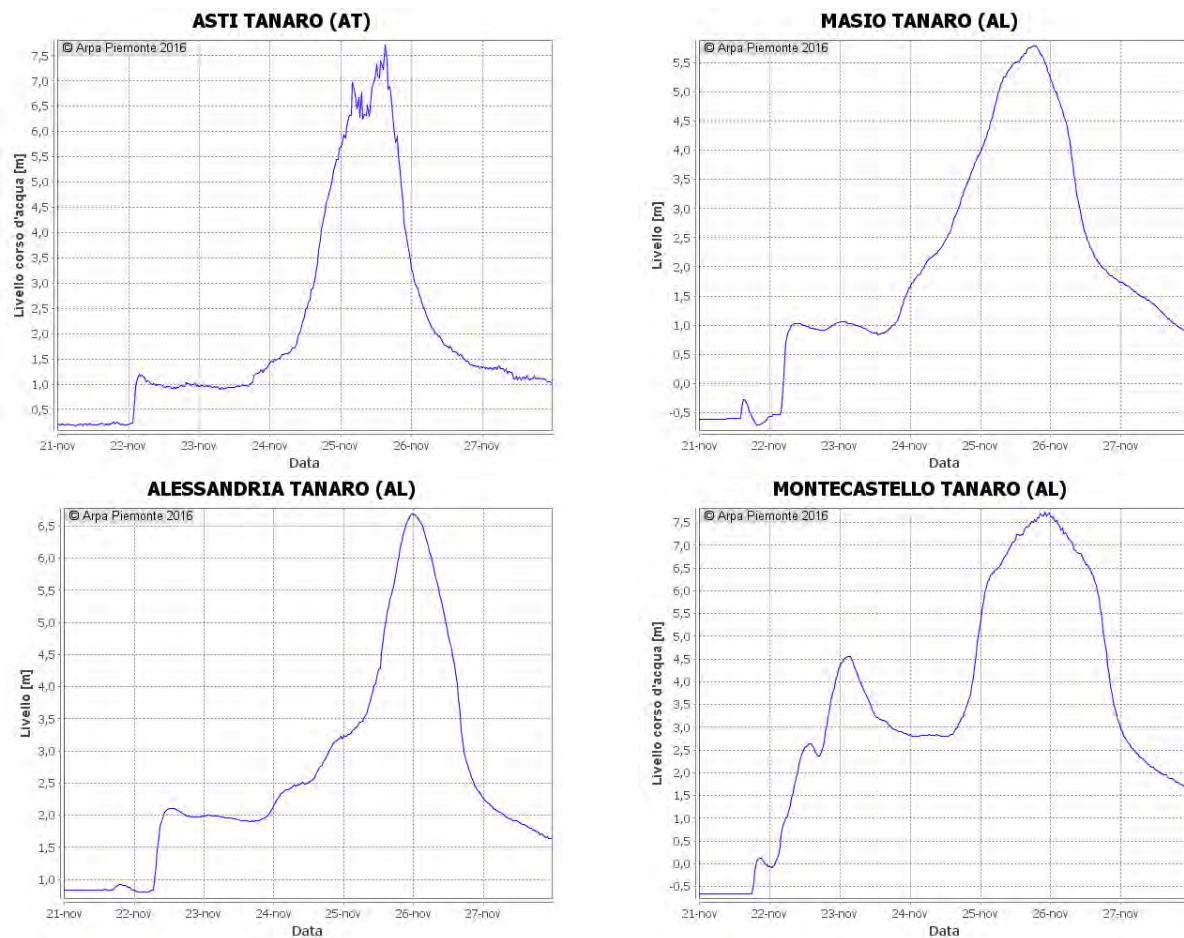
Figura 57. Idrogrammi delle stazioni del Tanaro,
