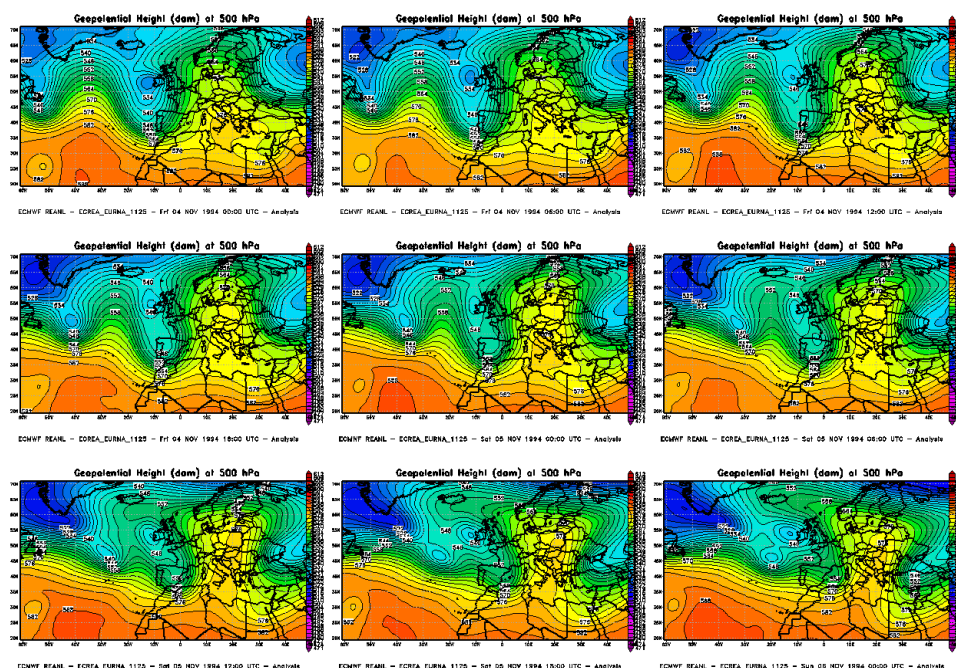
Figura 75. Mappe di analisi di Altezza Geopotenziale a 500hPa dal 4 novembre 1994 00UTC al 6 novembre 1994 00UTC
