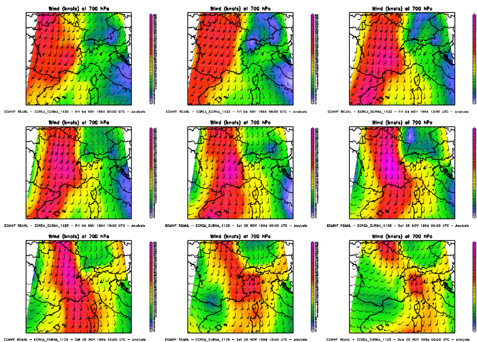
Figura 84. Venti a 700hPa dal 4 novembre 1994 00UTC al 6 novembre 1994 00UTC
