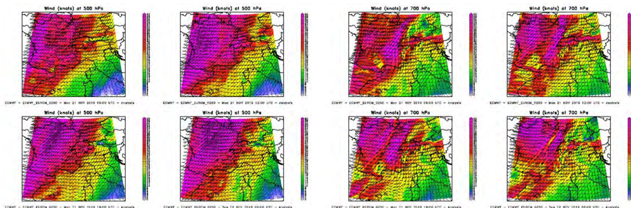
Figura 6. Analisi dei venti a 500hPa (sinistra) e 700hPa (destra) nella giornata del 21 novembre 2016
