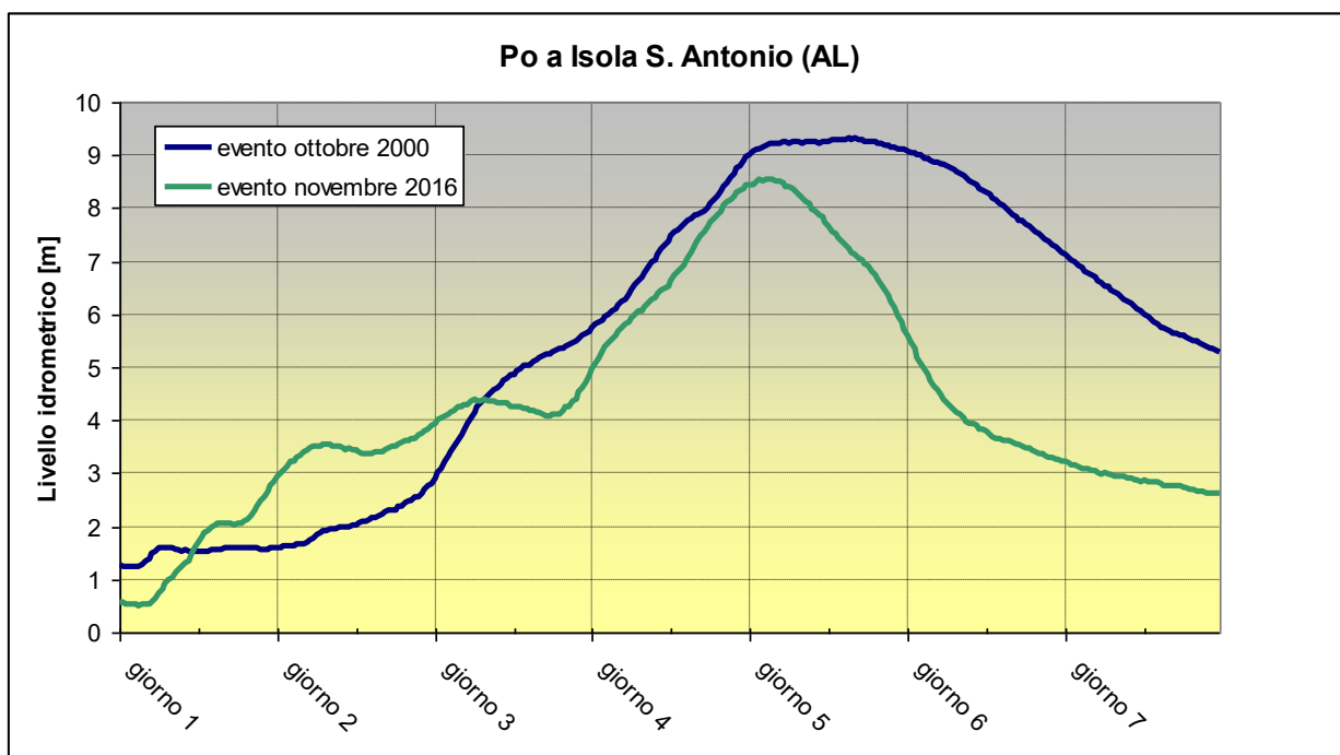
Figura 113. Confronto tra gli idrogrammi del Po a Isola S. Antonio (AL) registrati a ottobre 2000 e a novembre 2016
