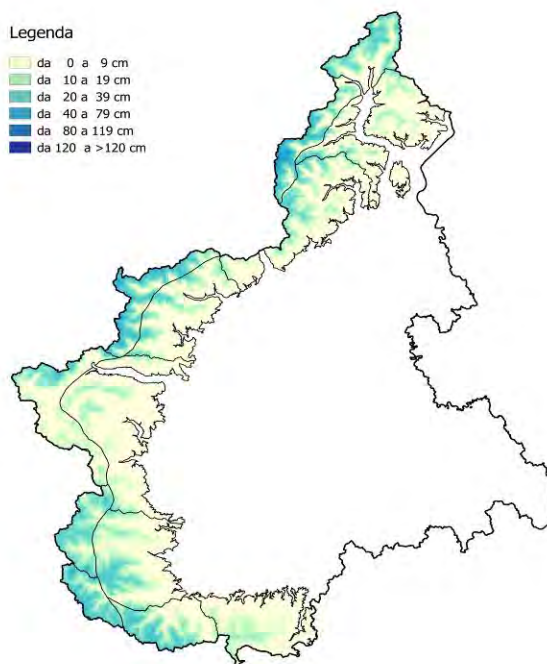
Figura 45. Neve fresca registrata il 22 novembre
