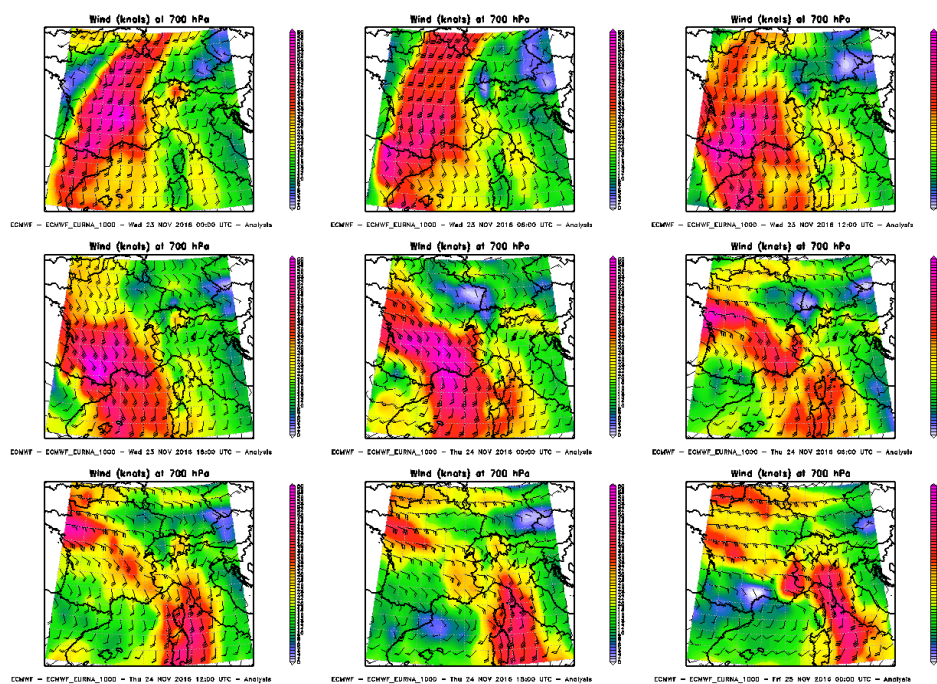
Figura 93. Venti a 700hPa dal 23 novembre 2016 00UTC al 25 novembre 2016 00UTC
