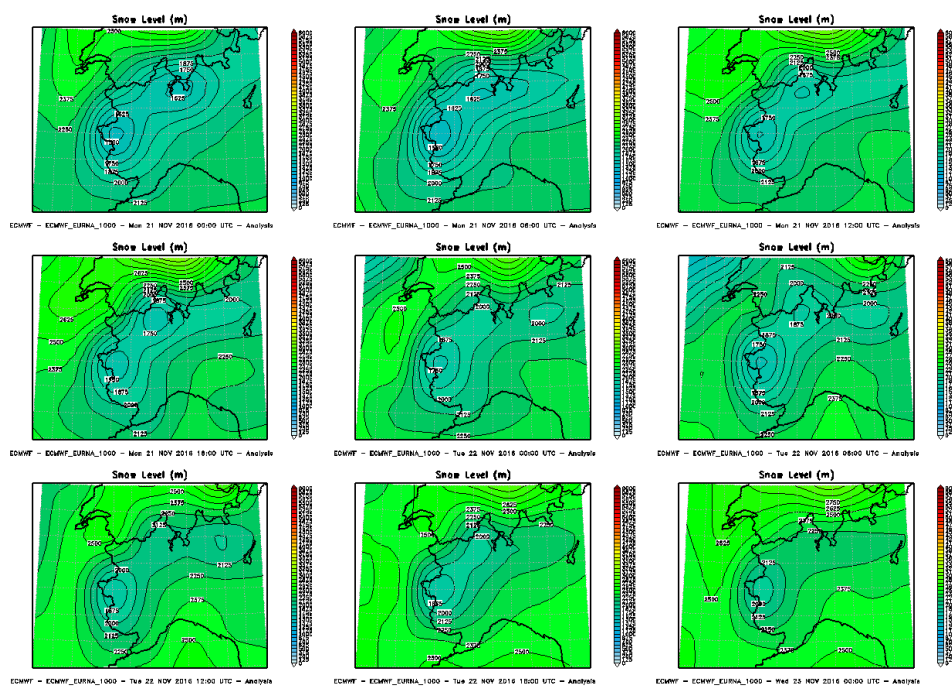
Figura 103. Quota neve dal 21 novembre 2016 00UTC al 23 novembre 2016 00UTC
