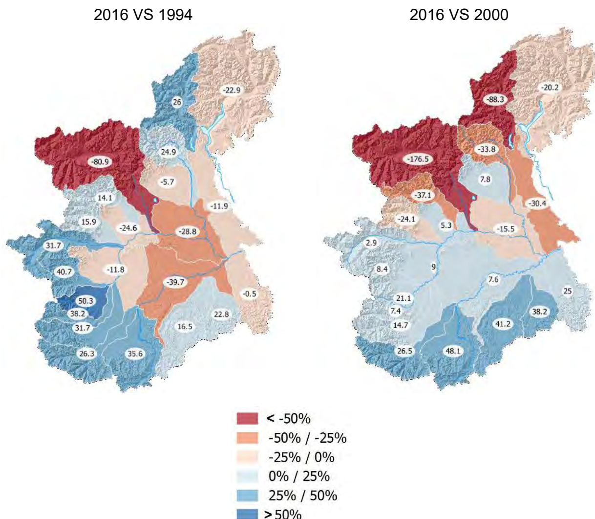
Figura 108. Scarti percentuali tra l'evento di novembre 2016 e gli eventi passati per bacino idrografico
