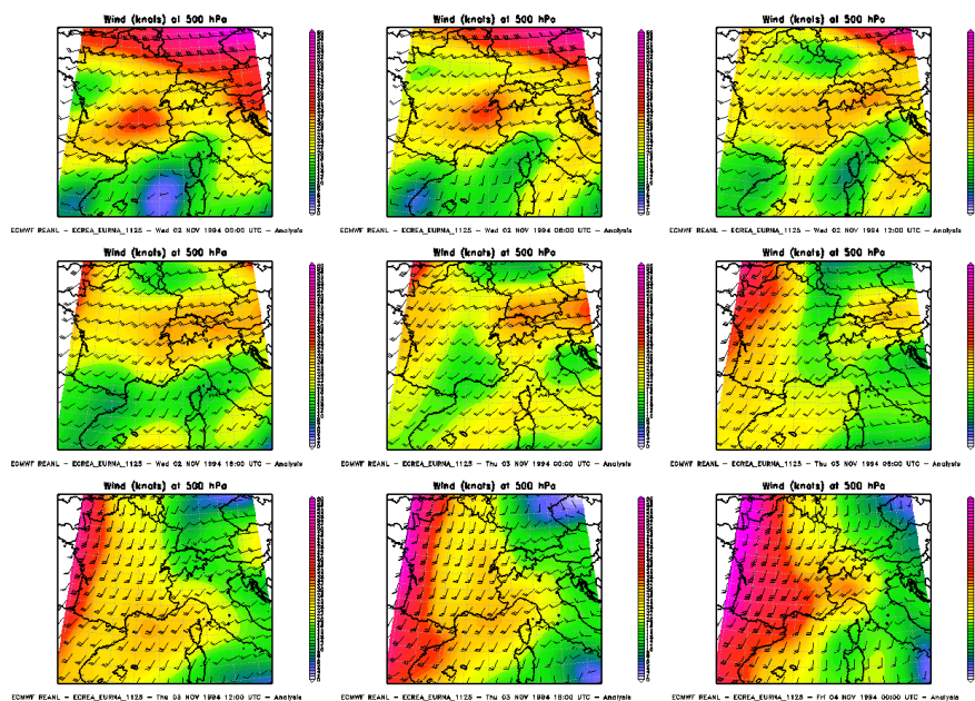
Figura 80. Venti a 500hPa dal 2 novembre 1994 00UTC al 4 novembre 1994 00UTC
