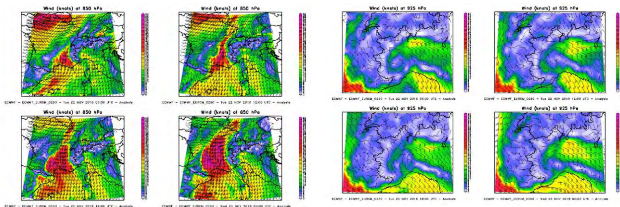
Figura 16. Analisi dei venti a 850hPa (sinistra) e 925hPa (destra) nella giornata del 22 novembre 2016
