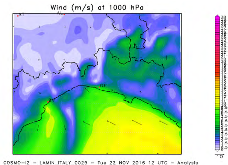
Figura 17. Venti nei bassi strati dell'atmosfera (1000 hPa) alle 12:00 UTC del 22 novembre 2016
