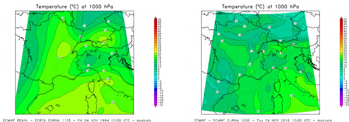
Figura 99. Temperatura dell'aria a 1000hPa il 4 novembre 1994 alle 12UTC (a sinistra) ed il 24 novembre 2016 alle 12UTC (a destra)
