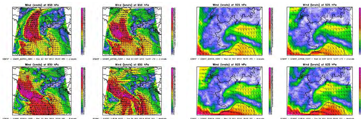
Figura 24. Analisi dei venti a 850hPa (sinistra) e 925hPa (destra) nella giornata del 23 novembre 2016
