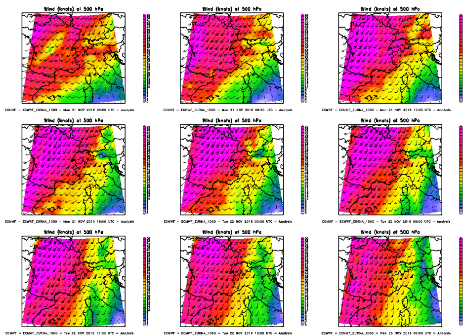
Figura 89. Venti a 500hPa dal 21 novembre 2016 00UTC al 23 novembre 2016 00UTC
