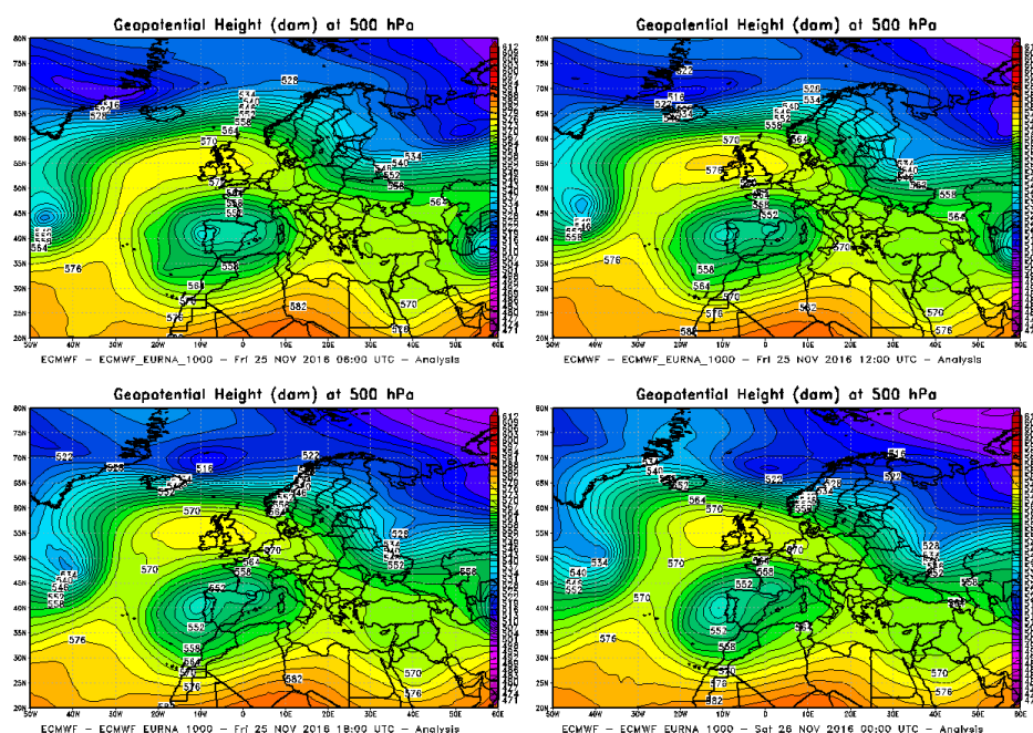
Figura 79. Mappe di analisi di Altezza Geopotenziale a 500hPa dal 25 novembre 2016 06UTC al 26 novembre 2016 00UTC
