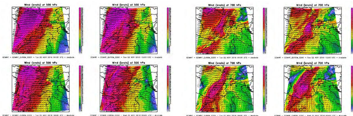
Figura 15. Analisi dei venti a 500hPa (sinistra) e 700hPa (destra) nella giornata del 22 novembre 2016
