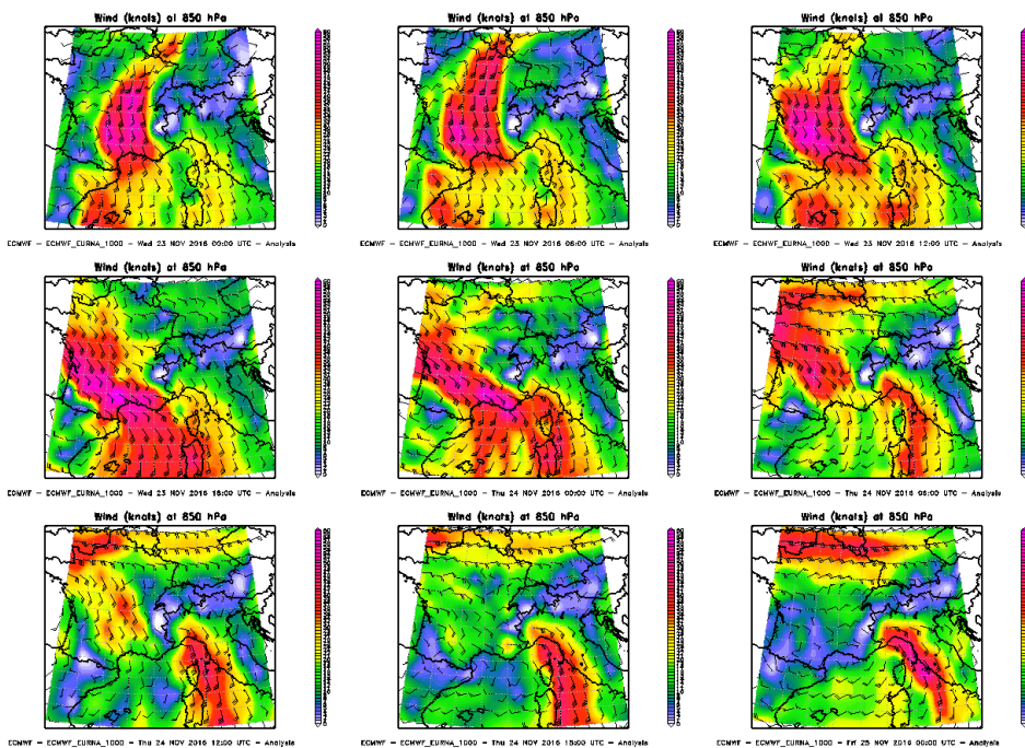
Figura 96. Venti a 850hPa dal 23 novembre 2016 00UTC al 25 novembre 2016 00UTC
