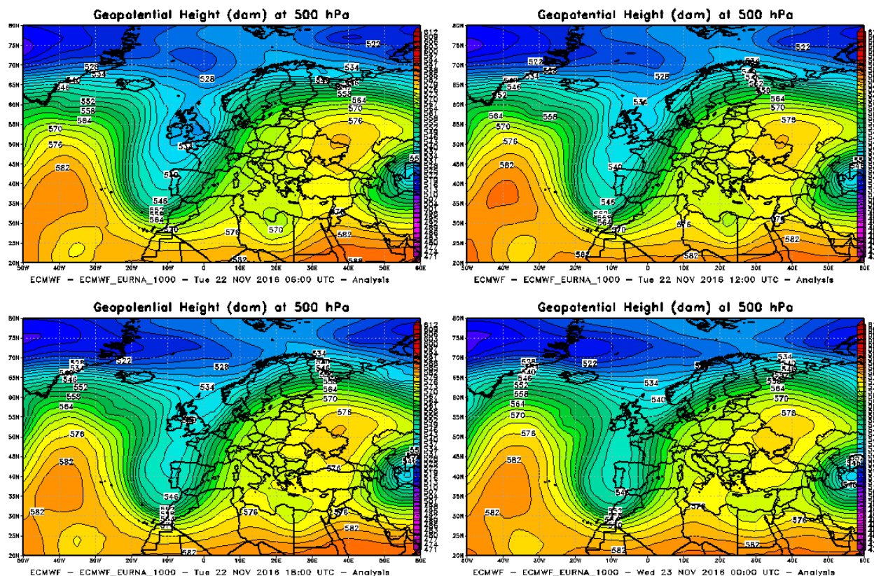
Figura 13. Analisi dell'altezza di geopotenziale a 500hPa nella giornata del 22 novembre 2016
