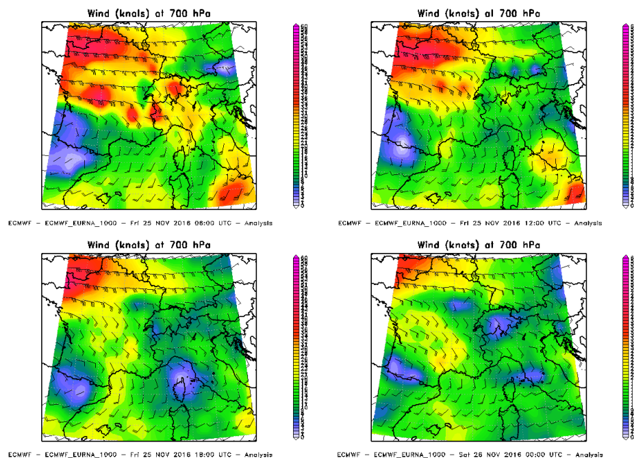
Figura 94. Venti a 700hPa dal 25 novembre 2016 06UTC al 26 novembre 2016 00UTC
