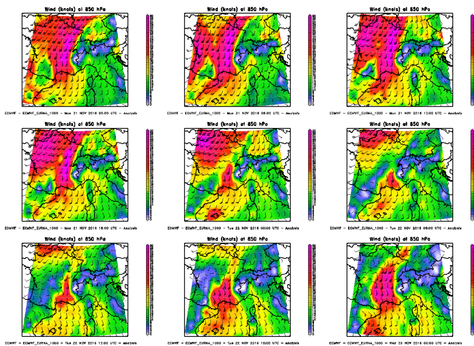
Figura 95. Venti a 850hPa dal 21 novembre 2016 00UTC al 23 novembre 2016 00UTC
