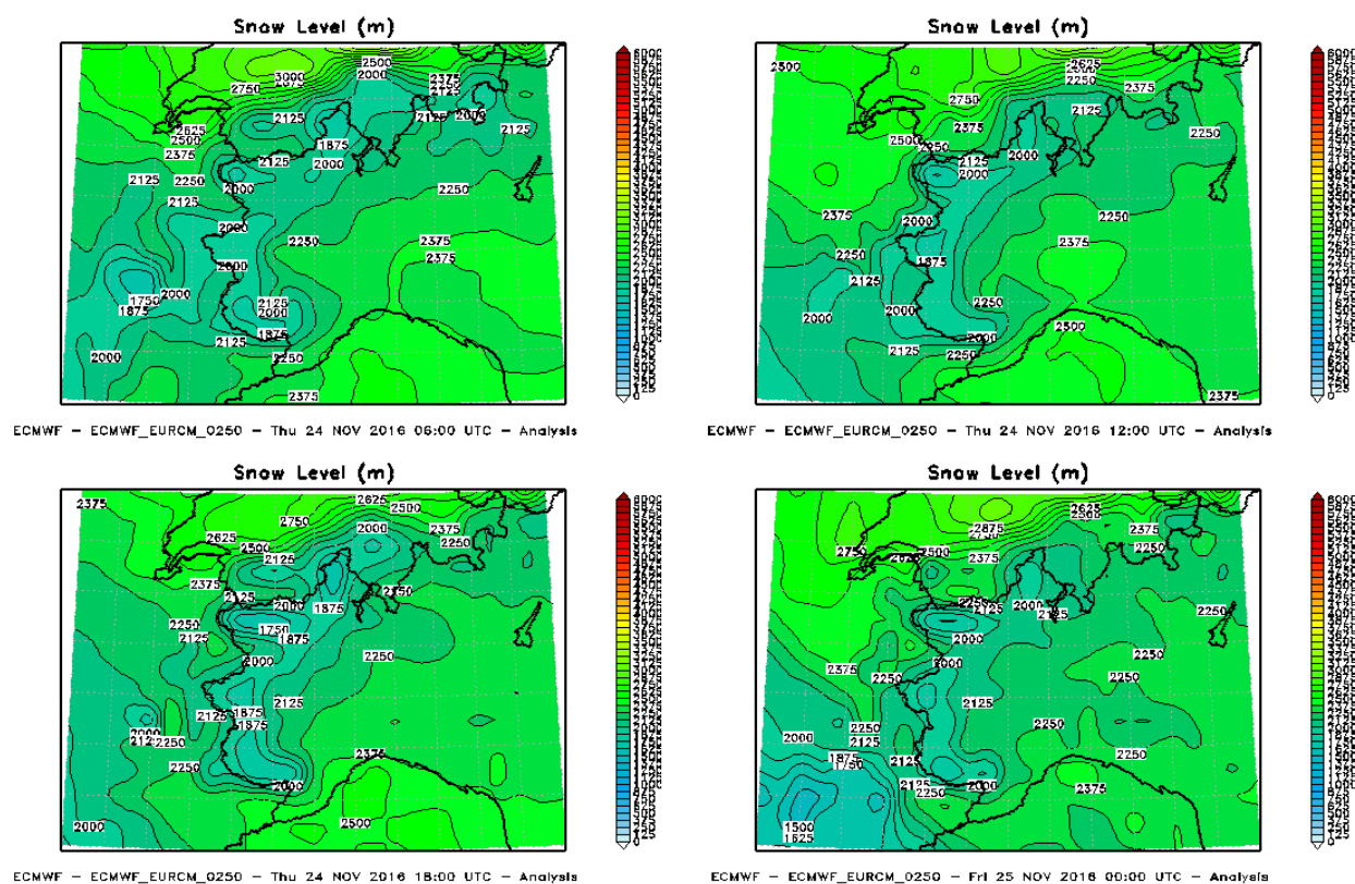
Figura 35. Analisi della quota neve per la giornata del 24 novembre 2016
