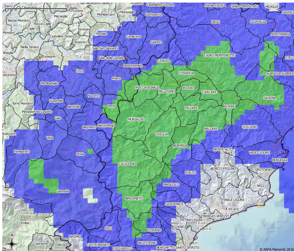
Figura 33. Stima della probabilità di grandine derivata dal sistema radar meteorologico piemontese. Le aree in verde mostrano le zone interessate dal fenomeno della grandine mista a pioggia.
