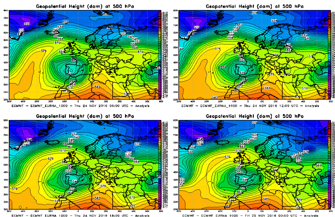
Figura 28. Analisi dell'altezza di geopotenziale a 500hPa nella giornata del 24 novembre 2016
