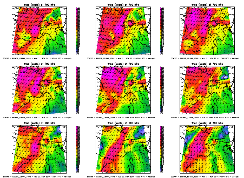
Figura 92. Venti a 700hPa dal 21 novembre 2016 00UTC al 23 novembre 2016 00UTC
