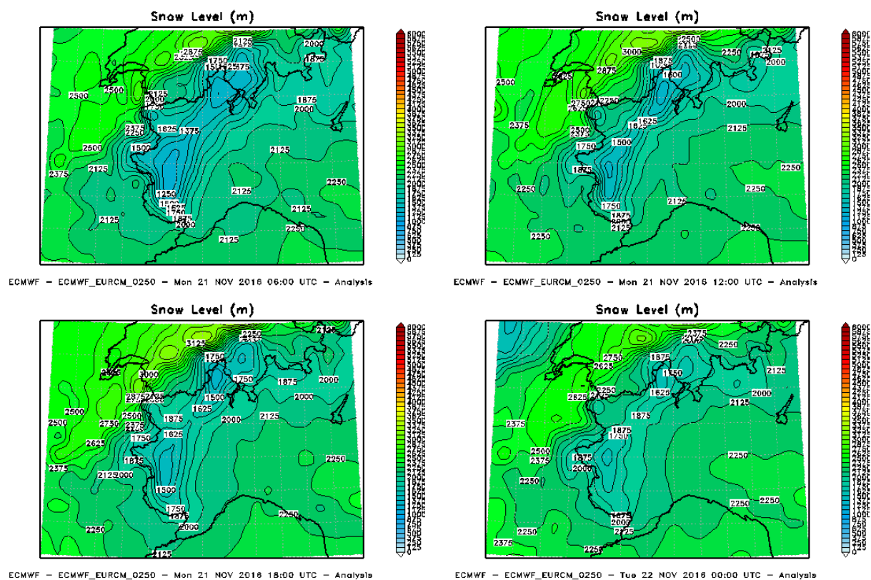
Figura 12. Analisi della quota neve per la giornata del 21 novembre 2016
