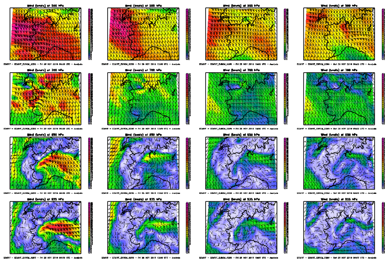
Figura 37. Analisi dei venti alle quote sinottiche principali nella giornata del 25 novembre 2016
