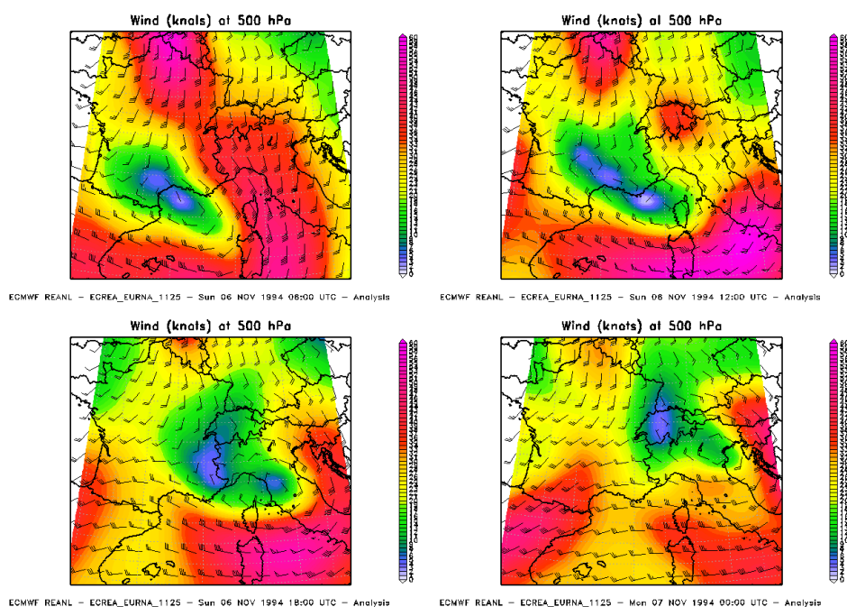
Figura 82. Venti a 500hPa dal 6 novembre 1994 06UTC al 7 novembre 1994 00UTC
