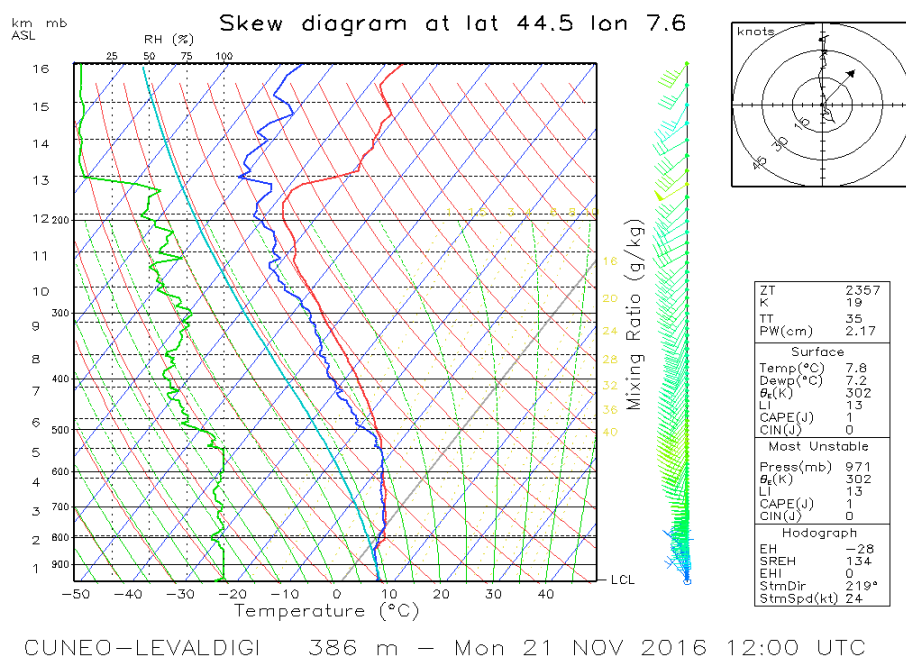
Figura 8. Radiosondaggio di Cuneo Levaldigi delle ore 12UTC del 21 novembre 2016. Si vede bene un cospicuo apporto di umidità su tutta la colonna d'aria dal suolo fino a 500 hPa per venti prevalentemente di Libeccio.
