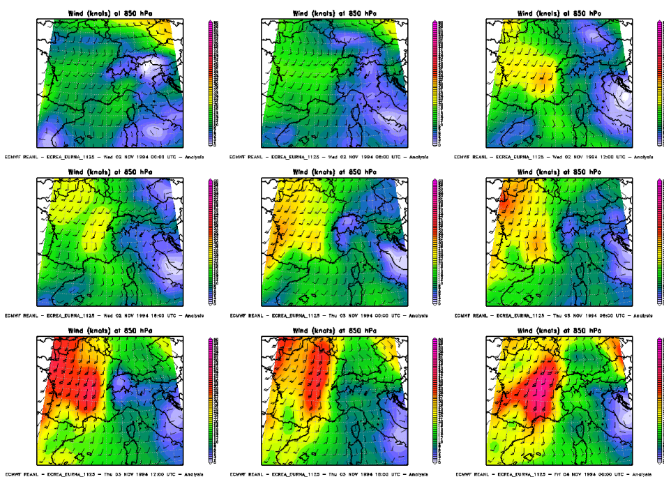
Figura 86. Venti a 850hPa dal 2 novembre 1994 00UTC al 4 novembre 1994 00UTC
