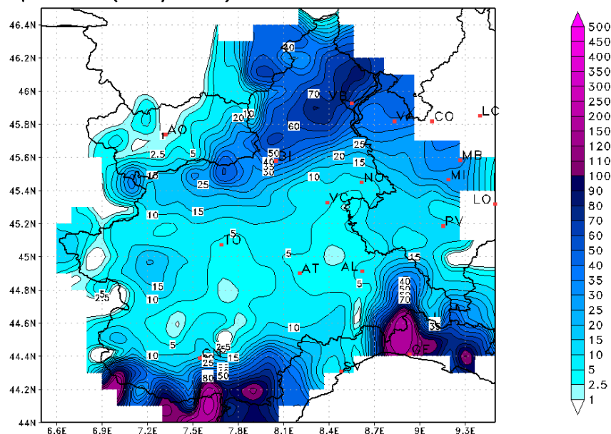
Figura 9. Precipitazioni cumulate durante la giornata del 21 novembre 2016
