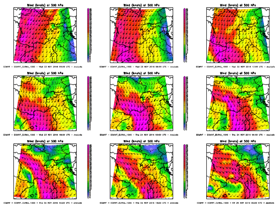
Figura 90. Venti a 500hPa dal 23 novembre 2016 00UTC al 25 novembre 2016 00UTC
