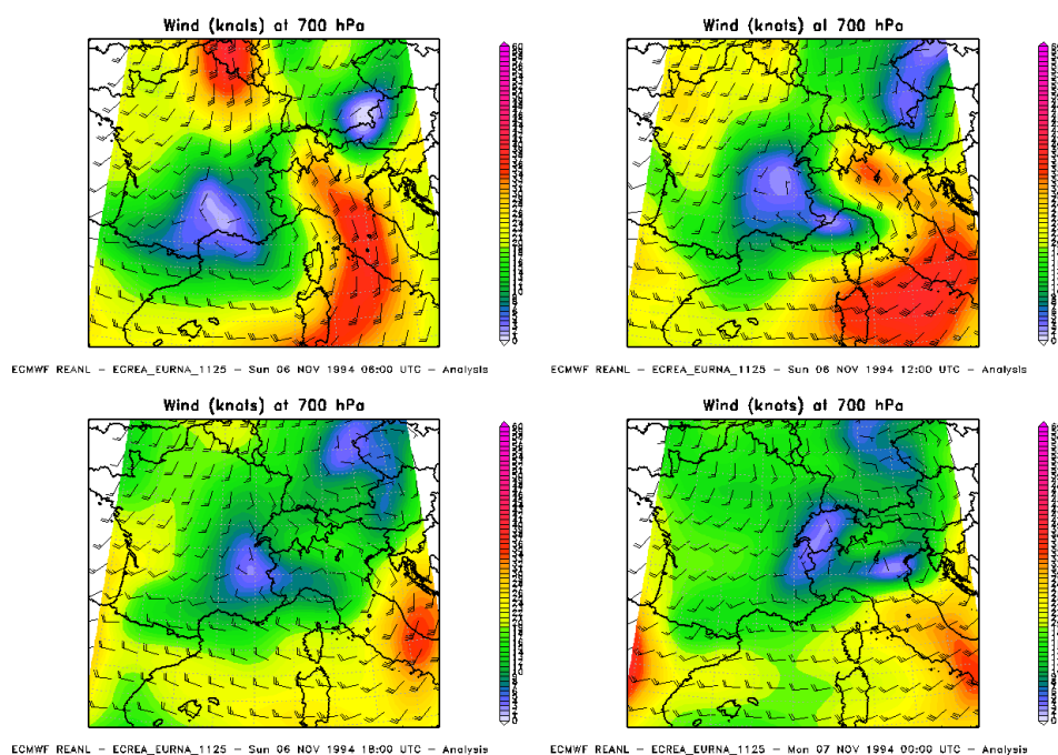
Figura 85. Venti a 700hPa dal 6 novembre 1994 06UTC al 7 novembre 1994 00UTC
