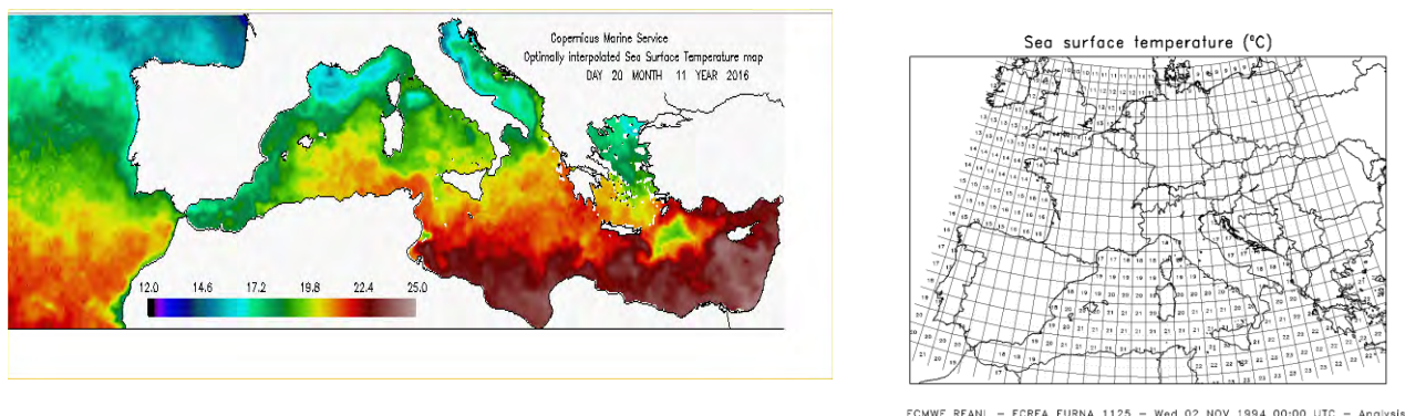
Figura 98. Temperatura superficiale del mare il 20 novembre 2016 (a sinistra) ed il 2 novembre 1994 (a destra)
