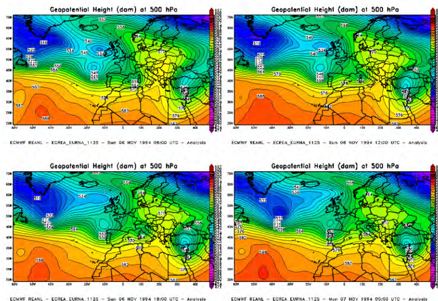
Figura 76. Mappe di analisi di Altezza Geopotenziale a 500hPa dal 6 novembre 1994 06UTC al 7 novembre 1994 00UTC
