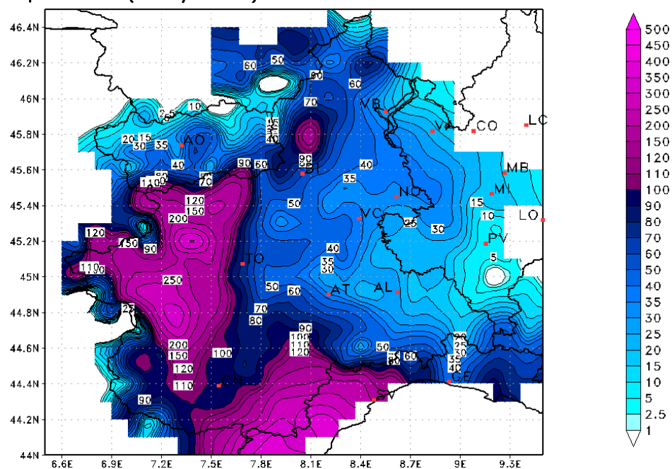
Figura 31. Precipitazioni cumulate durante la giornata del 24 novembre 2016
