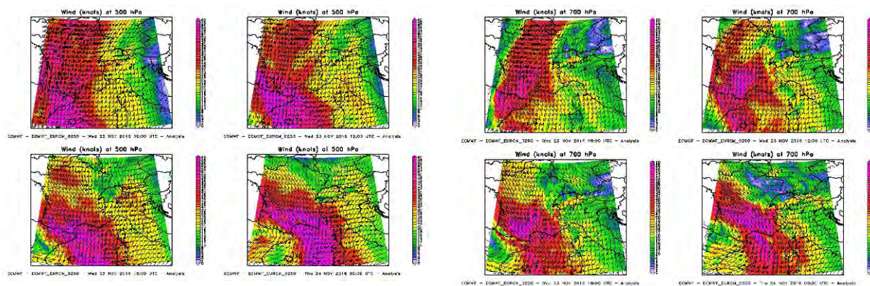
Figura 23. Analisi dei venti a 500hPa (sinistra) e 700hPa (destra) nella giornata del 23 novembre 2016
