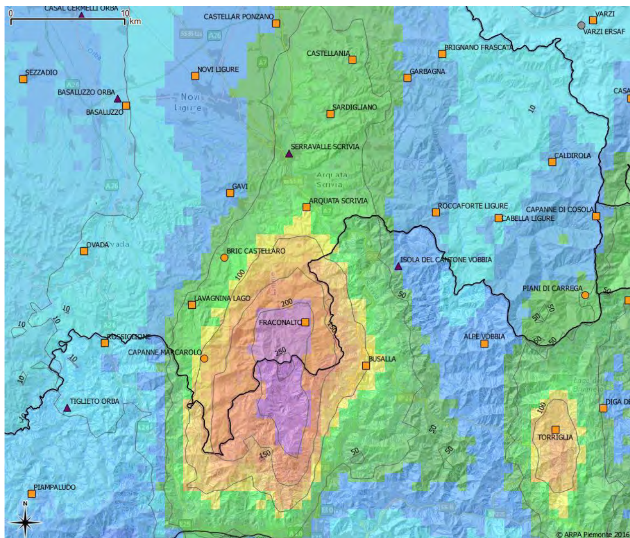
Figura 11. Stima della precipitazione giornaliera del 21 novembre 2016 stimata dal sistema radar meteorologico piemontese e corretta con i pluviometri della rete meteo idrografica
