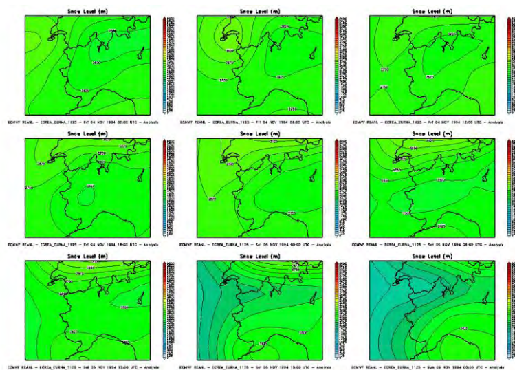
Figura 101. Quota neve tra il 4 novembre 1994 00UTC ed il 6 novembre 1994 00UTC
