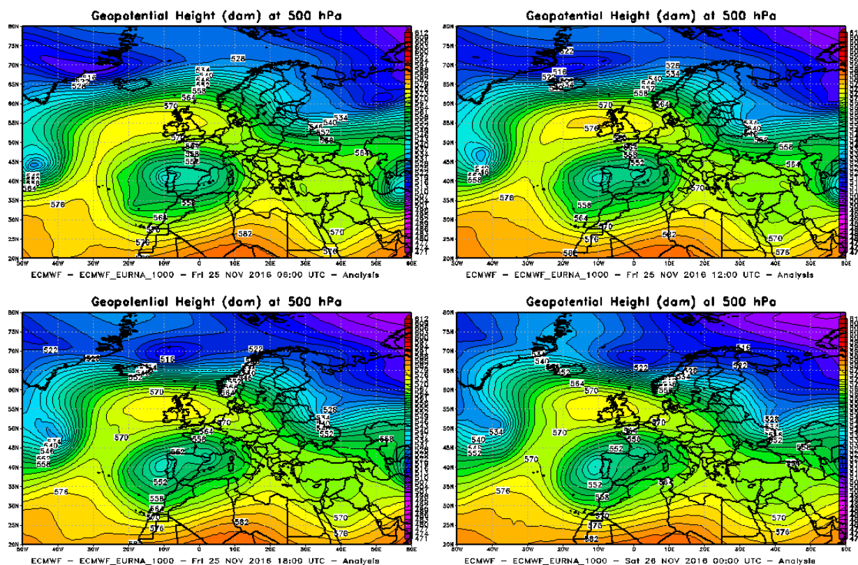
Figura 36. Analisi dell'altezza di geopotenziale a 500hPa nella giornata del 25 novembre 2016
