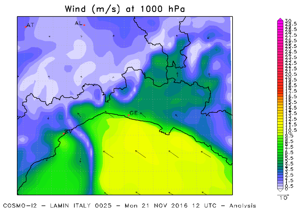
Figura 10. I venti in bassa quota (1000 hPa) alle 12 UTC del 21 novembre 2016 al confine con la Liguria. Si vede molto bene la zona di convergenza sul mare che attraversa il golfo ligure portandosi sul savonese.
