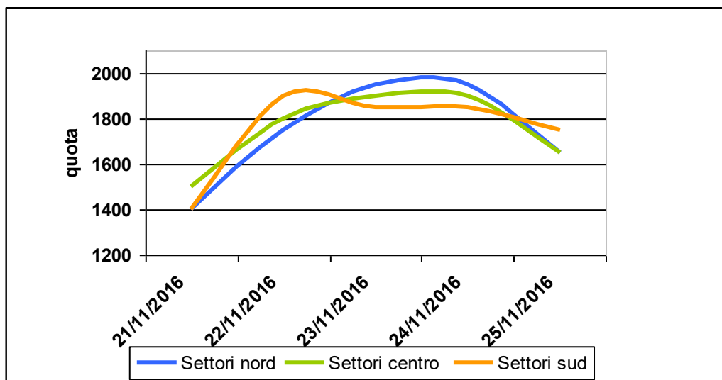
Figura 43. Andamento dello zero termico nei diversi settori durante l'evento
