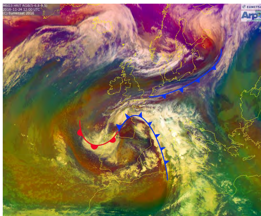
Figura 29. Immagine Meteosat (airmass, composizione di bande di infrarosso) alle 12UTC del 24 novembre 2016 con mappa dei fronti
