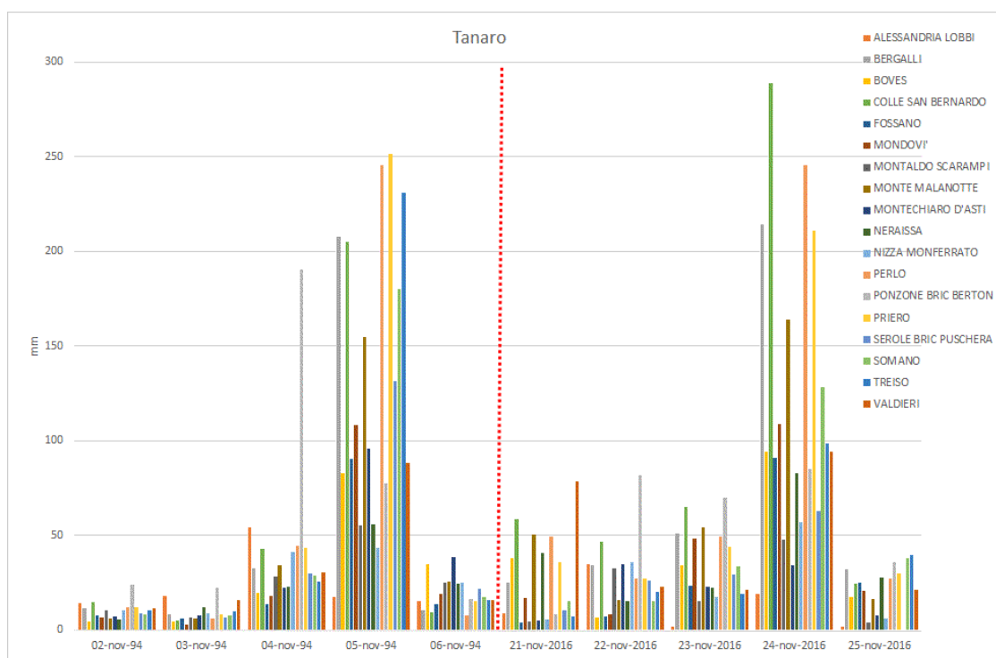
Figura 110. Confronto tra i due eventi alluvionali delle piogge cumulate giornaliere registrate dalle stazioni di monitoraggio installate nel bacino del Tanaro
