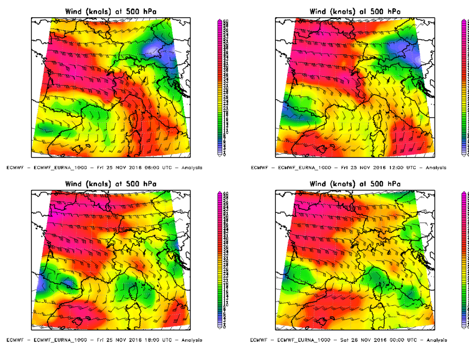
Figura 91. Venti a 500hPa dal 25 novembre 2016 06UTC al 26 novembre 2016 00UTC
