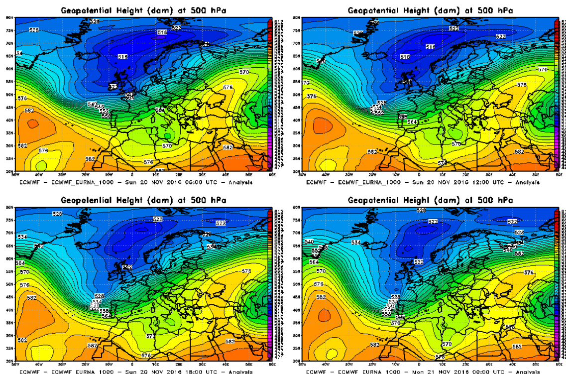
Figura 1. Analisi dell'altezza di geopotenziale a 500hPa nella giornata del 20 novembre 2016
