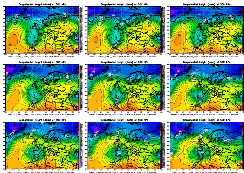
Figura 78. Mappe di analisi di Altezza Geopotenziale a 500hPa dal 23 novembre 2016 16:00UTC al 25 novembre 2016 00UTC
