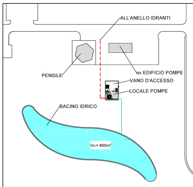
Figura 2-56 – Layout degli interventi previsti
