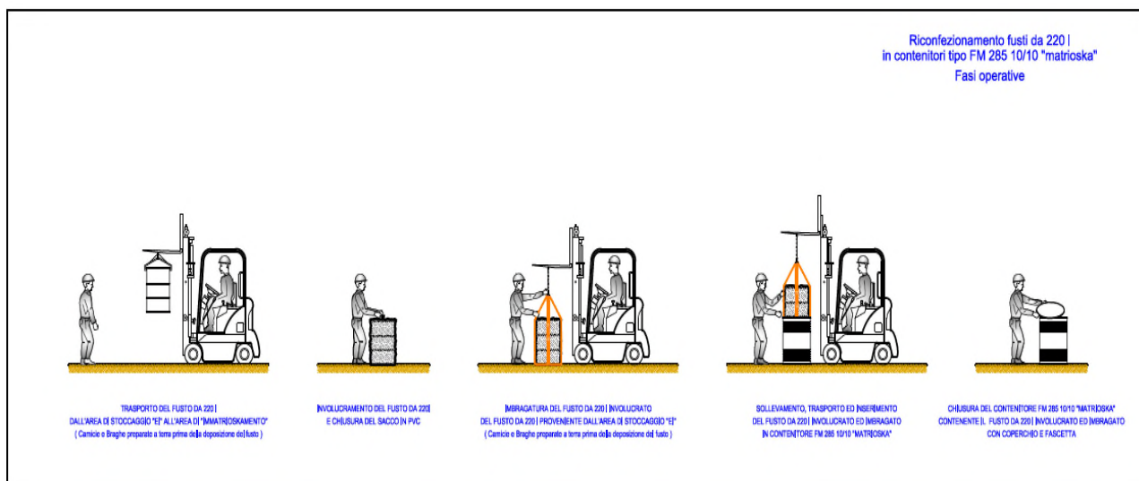
Figura 2-53 – Attività di predisposizione dei fusti al trasporto (schema)
