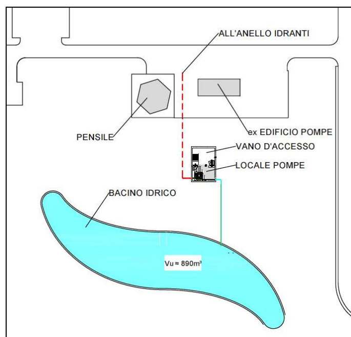
Figura 2-50 – Layout degli interventi previsti
