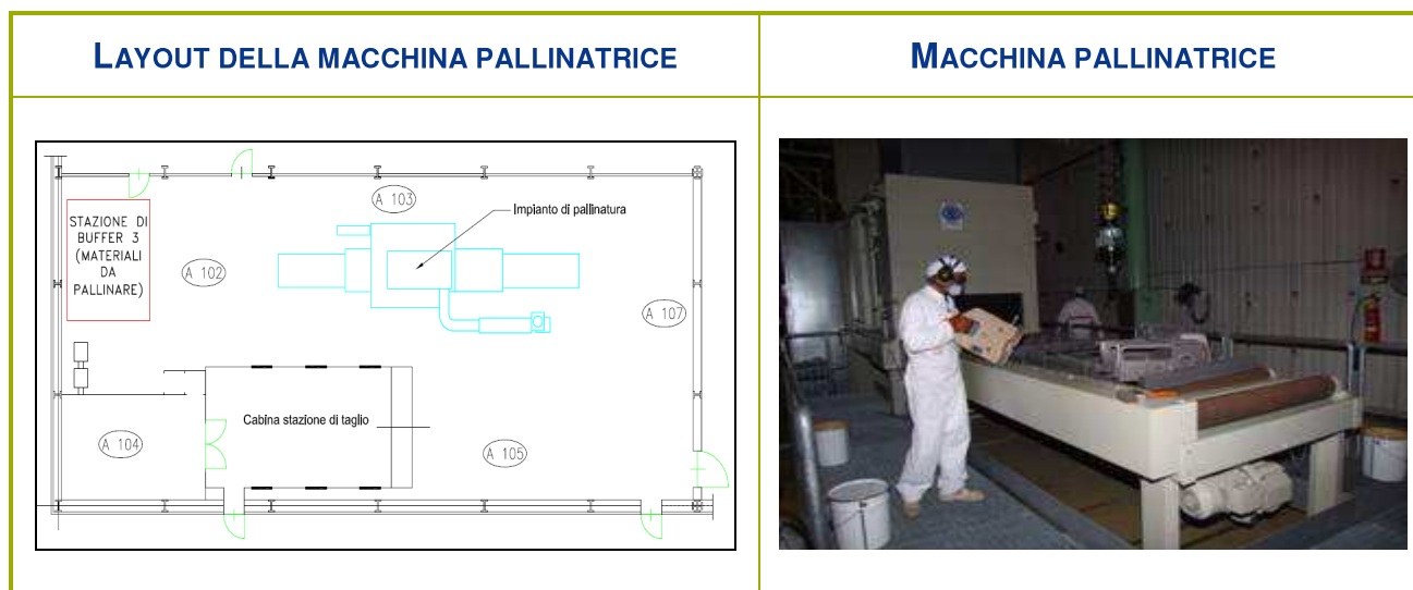
Figura 2-7 – Macchina pallinatrice
