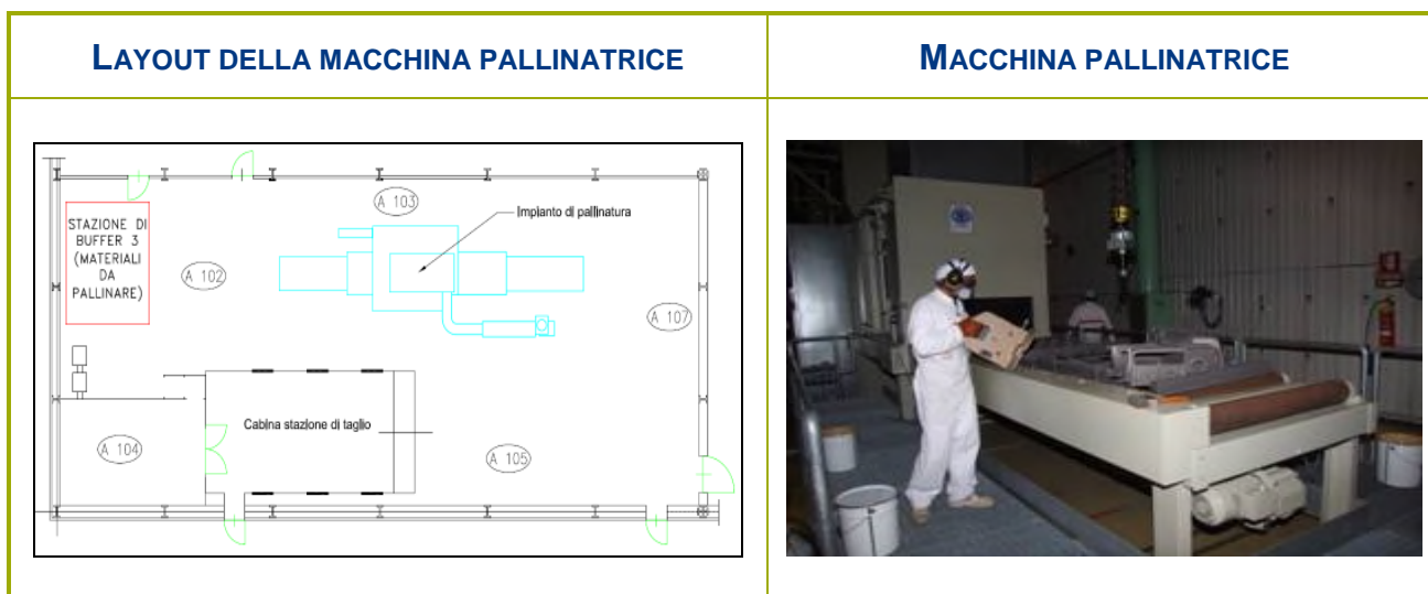
Figura 2-6 – Macchina pallinatrice
