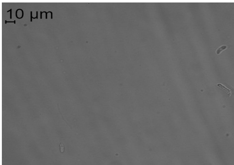
Exidia glandulosa nocciolo fusto conidi 43-sfr
