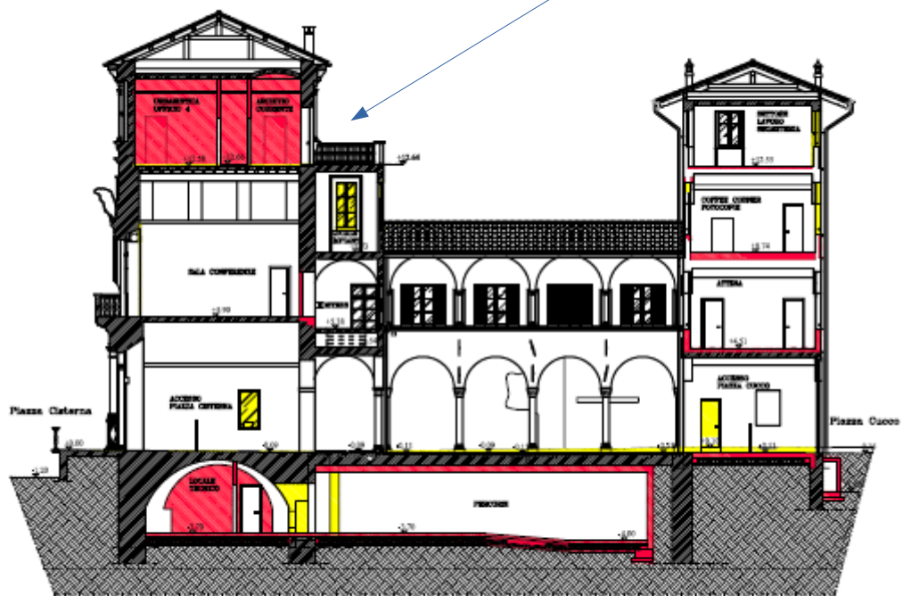
SEZIONE A-A
