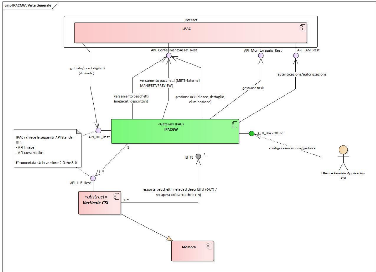
Figura 1- Diagramma di contesto
