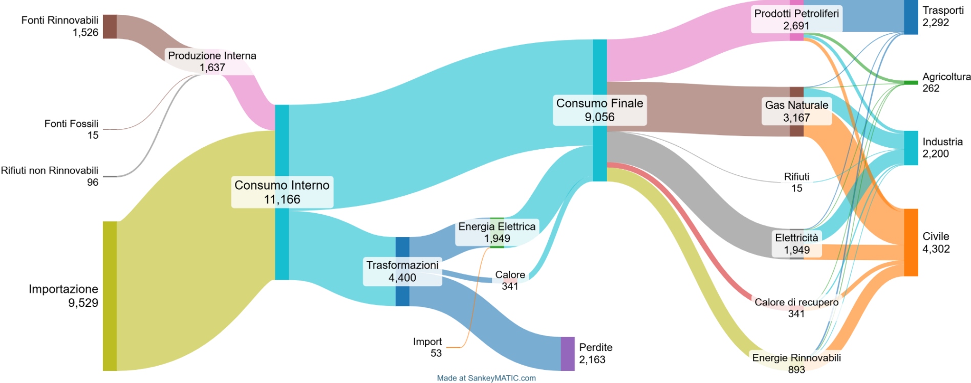
Figura 2.1 – Diagramma Sankey del Bilancio Energetico Regionale 2022 (dati in ktep con virgola usata come separatore delle migliaia)
