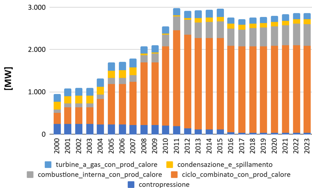
Figura 3.4 – Potenza efficiente lorda in impianti cogenerativi
