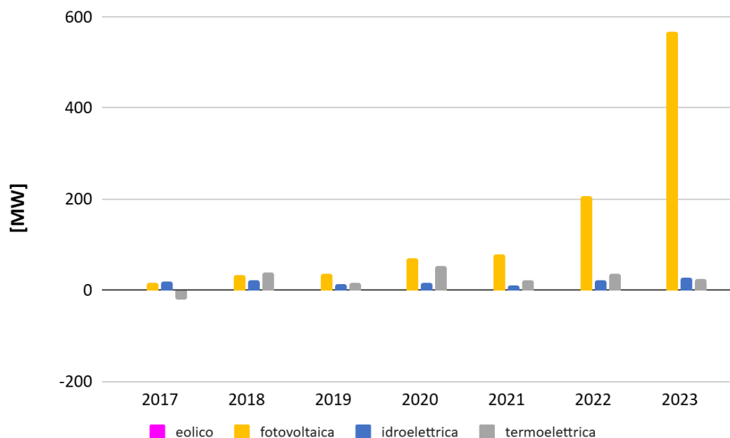
Figura 3.8 – Installazione annua della potenza efficiente lorda
