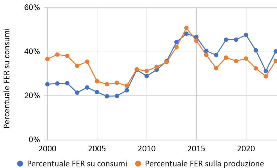
Figura 3.14 – Contributo delle FER su produzione e consumi elettrici
