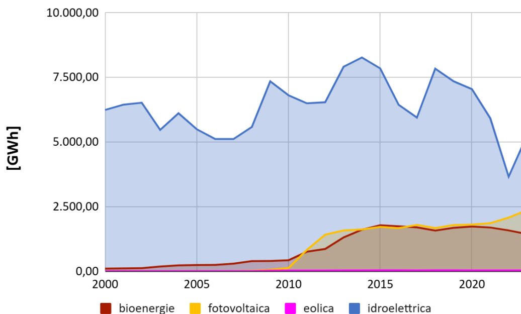
Figura 3.12 – Andamento della produzione rinnovabile elettrica netta
