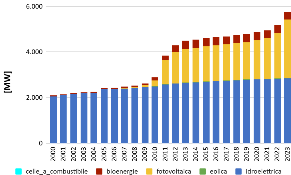
Figura 3.6 – Potenza efficiente lorda in impianti rinnovabili
