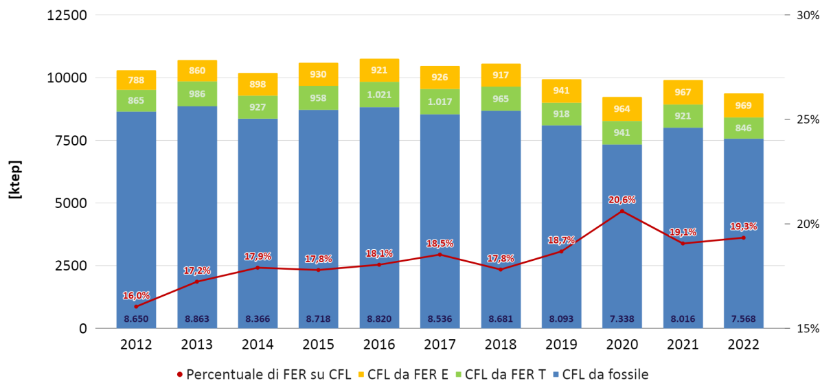
Figura 4.2 – Fonti Energetiche Rinnovabili (FER) e percentuale sui Consumi Finali Lordi
