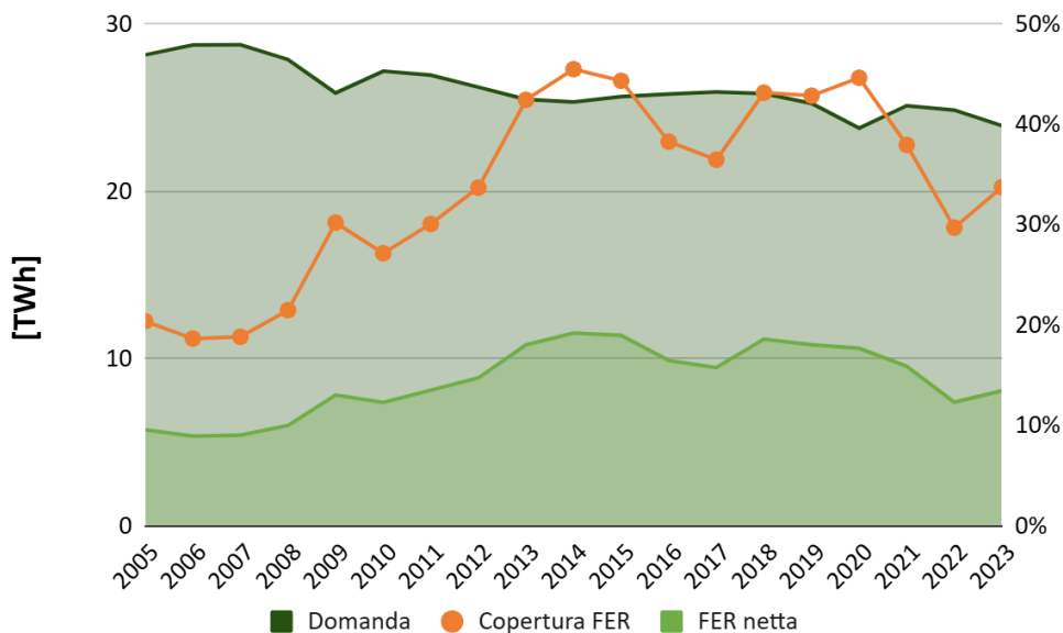
Figura 3.16 – Domanda elettrica e copertura da FER
