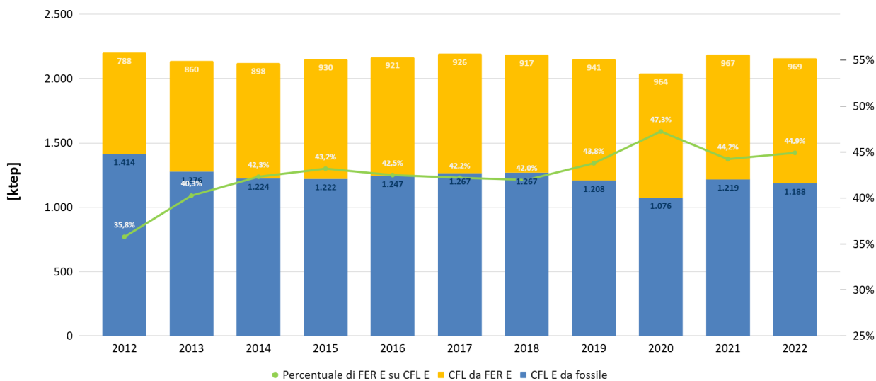
Figura 4.9 – Contributo delle rinnovabili elettriche sul Consumo Finale Lordo elettrico
