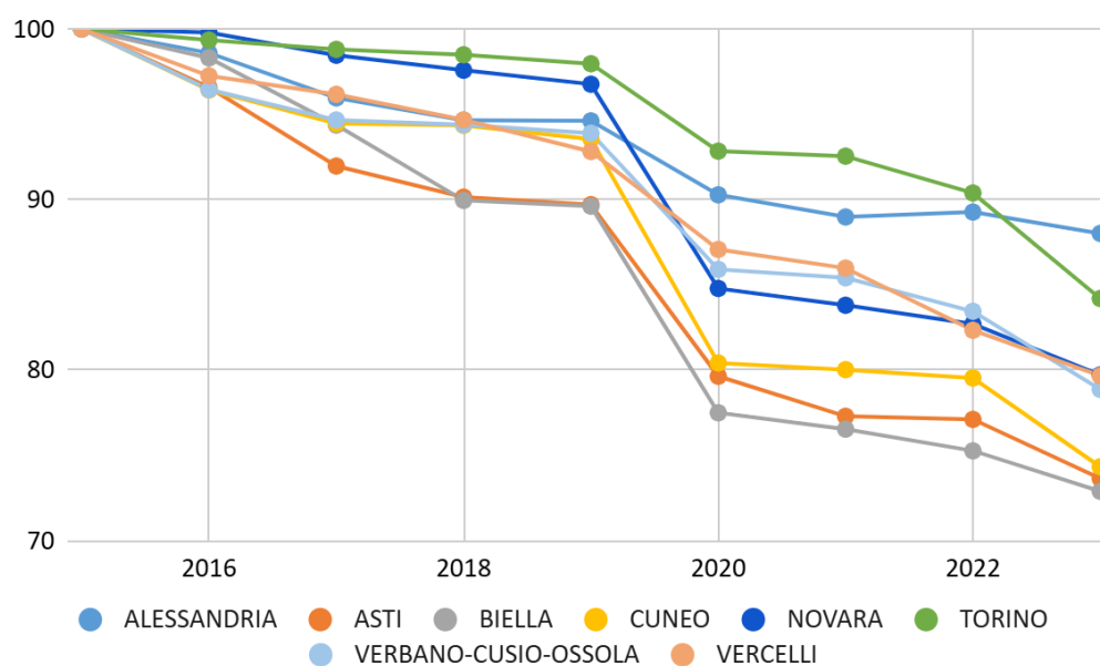
Figura 5.9 - Andamento dei consumi di energia elettrica per Pubblica Illuminazione rispetto al 2015
