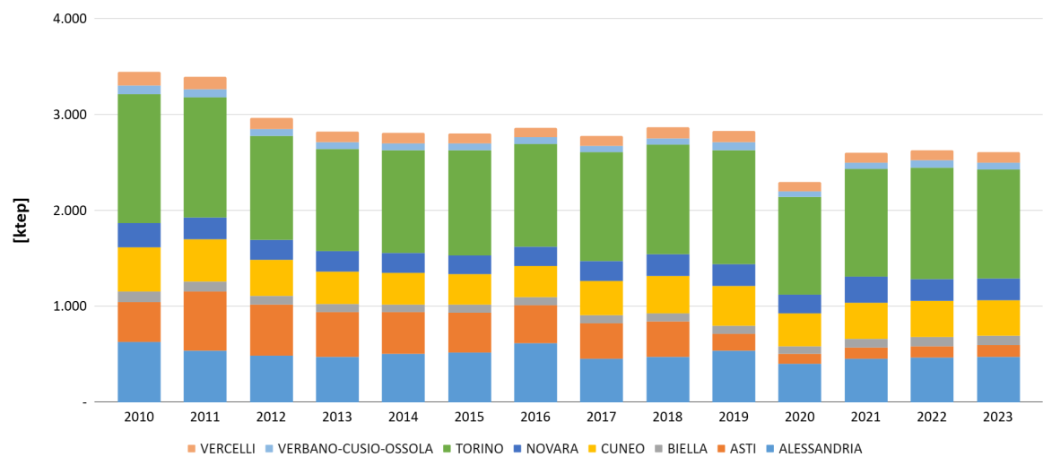
Figura 6.6 - Andamento delle vendite di prodotti petroliferi nelle Province Piemontesi
