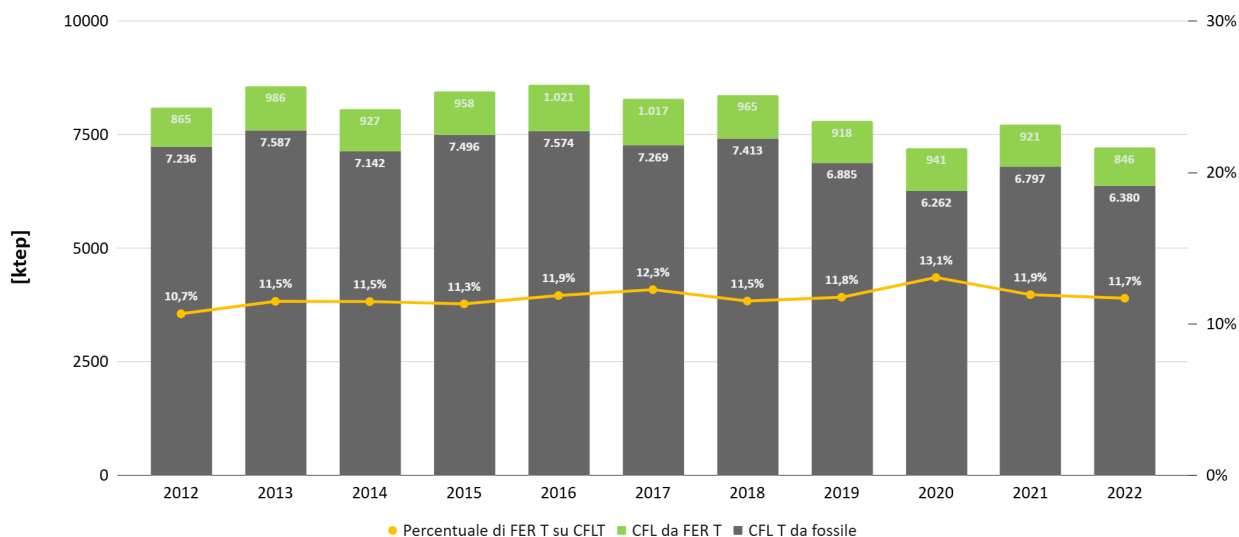
Figura 4.5 – Contributo delle rinnovabili termiche sul Consumo Finale Lordo termico
