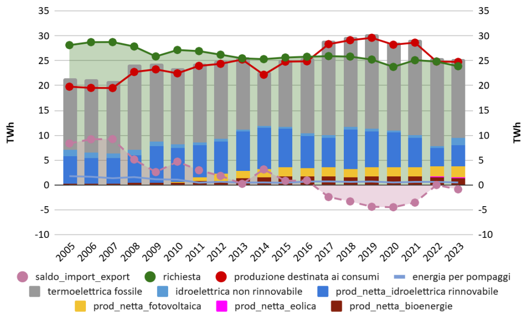
Figura 3.15 – Produzione e domanda elettrica in Piemonte
