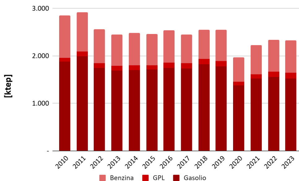
Figura 6.3 - Andamento delle vendite di prodotti petroliferi (autotrazione)
