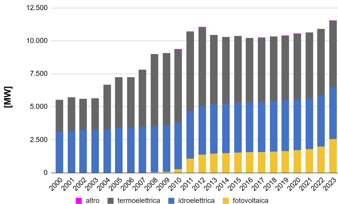
Figura 3.1 – Potenza efficiente lorda
