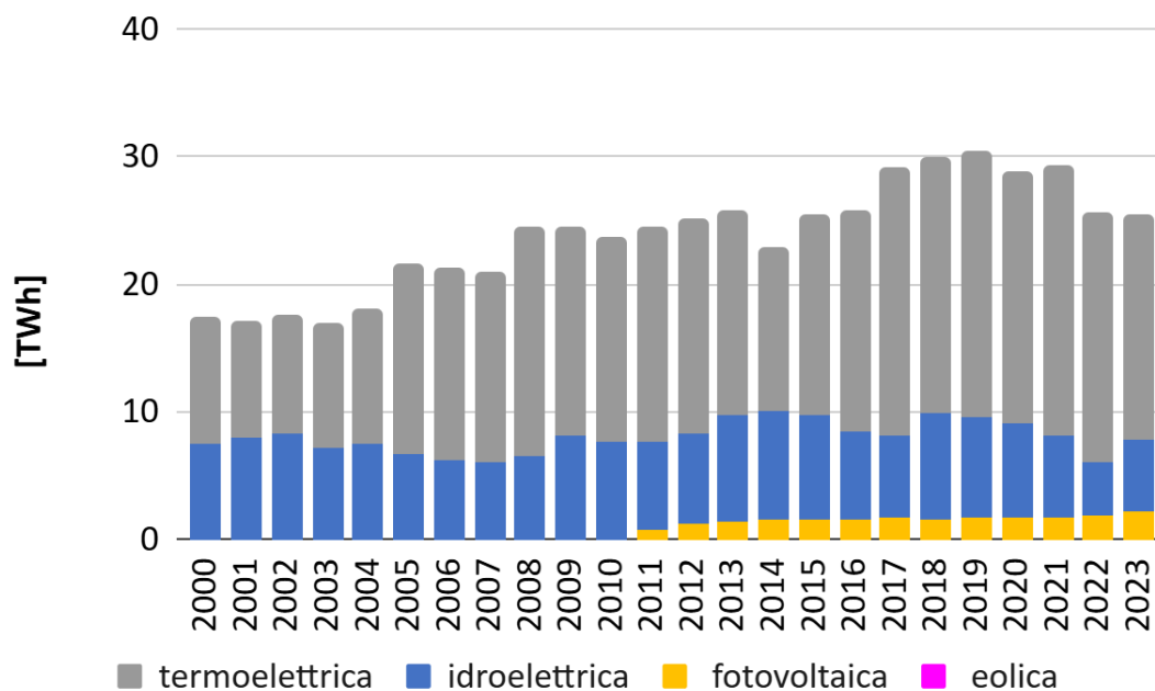
Figura 3.9 – Andamento della produzione elettrica netta
