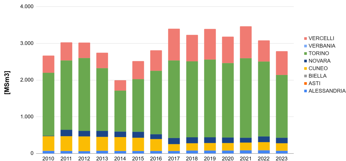
Figura 7.3 - Consumo di gas naturale per produzione termoelettrica per provincia (Dati in MSm3)
