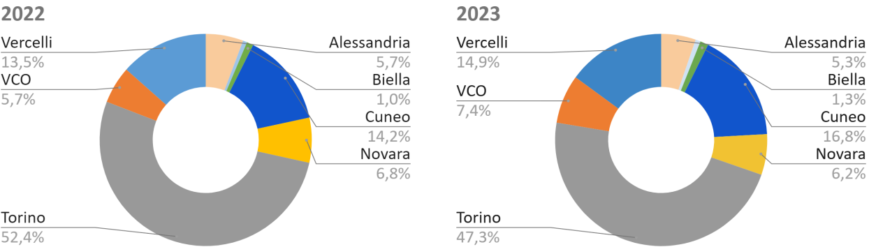
Figura 3.19 – Ripartizione della produzione elettrica netta tra province
