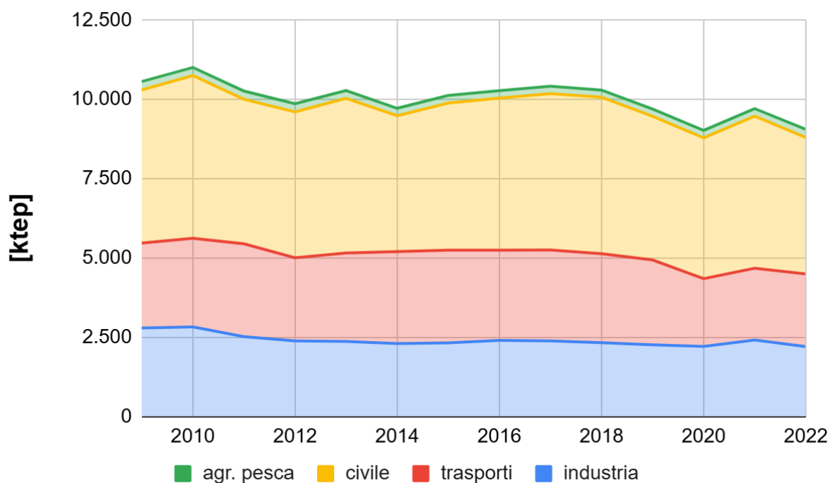
Figura 2.6 – Andamento dei consumi finali per settori. Valori assoluti
