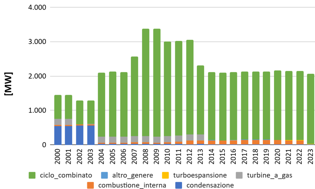
Figura 3.5 – Potenza efficiente lorda in impianti non cogenerativi
