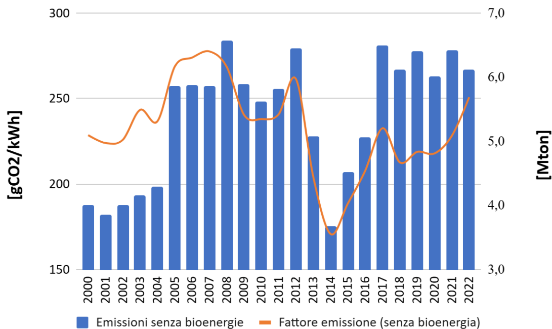
Figura 3.17 – Emissioni di CO2 e fattore di emissione nella generazione elettrica
