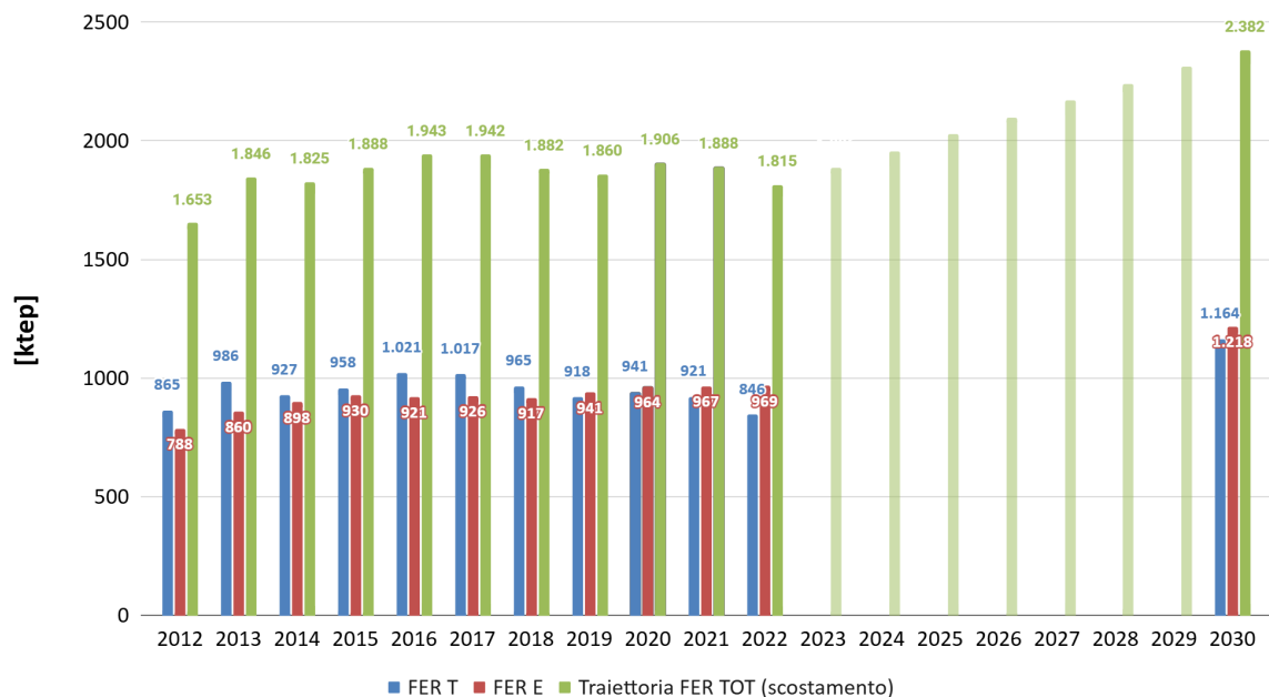
Figura 8.1 – Confronto con gli obiettivi del PEAR. Fonti Energetiche Rinnovabili
