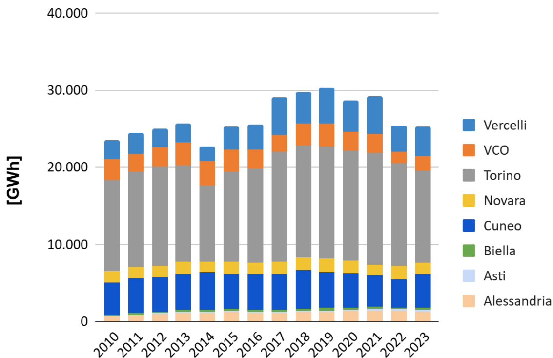
Figura 3.18 – Produzione elettrica netta per provincia
