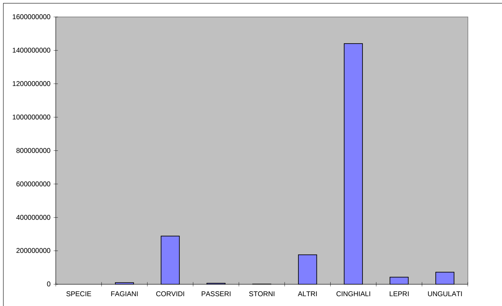
ANNO 1999 SPECIE FAUNISTICHE CAUSA DI DANNI NEL TERRITORIO DI COMPETENZA DEGLI ATC E DEI CA
