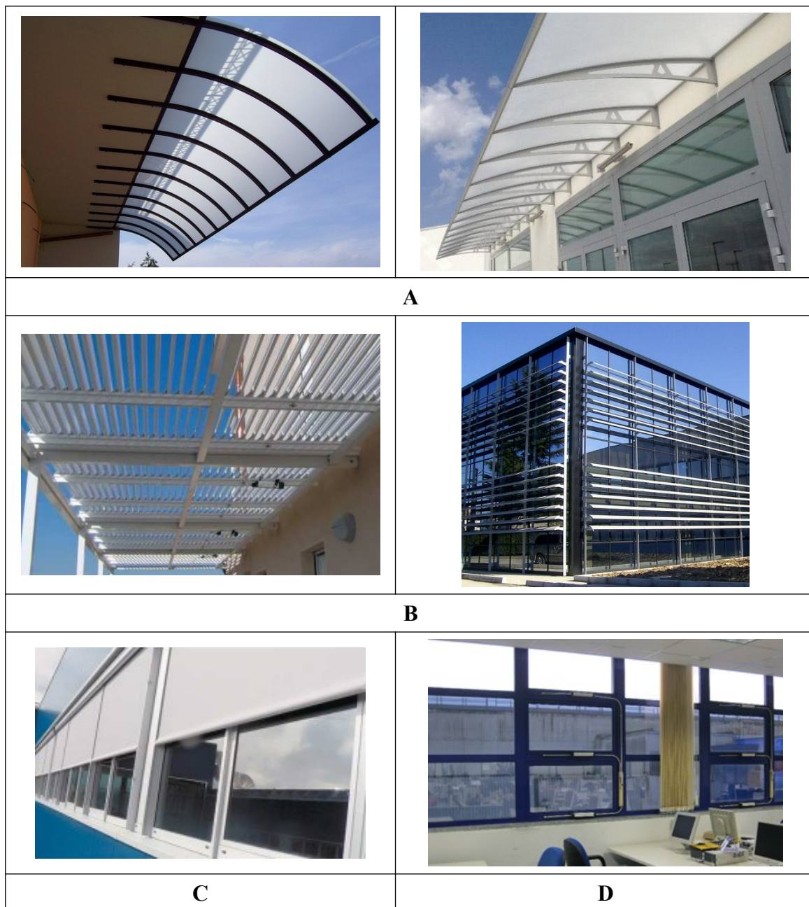
Figura 3 – Esempi di misure tecniche di contenimento dell’irraggiamento solare
