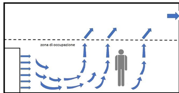
Figura 4. Sistema a dislocazione
