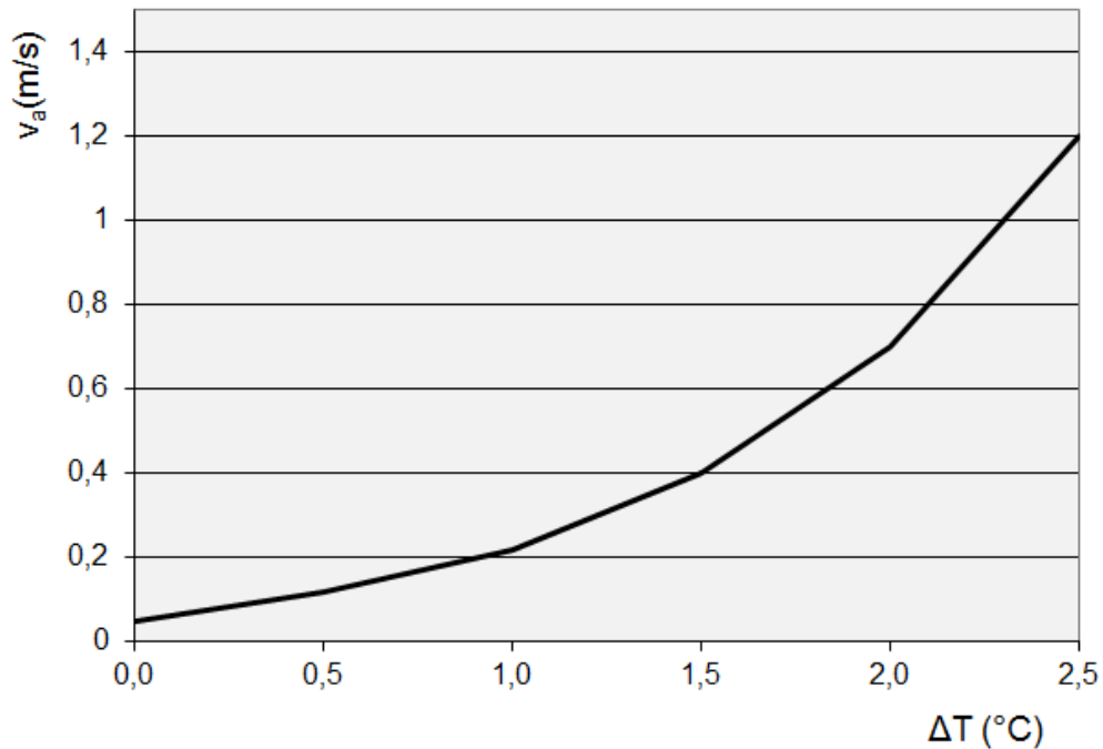
Figura 4 – Velocità dell’aria richiesta per compensare un aumento di temperatura
