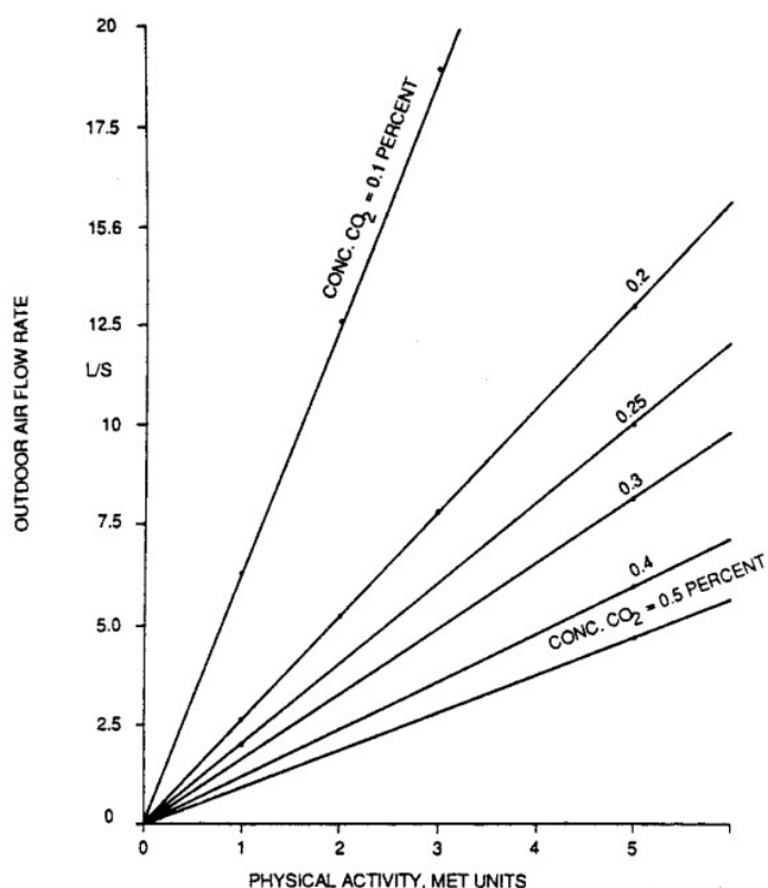
Figura 1. Requisiti per la ventilazione in funzione dell'attività
