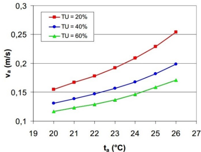
Figura 2. Valori limite della velocità dell'aria per l'accettabilità delle correnti d'aria
