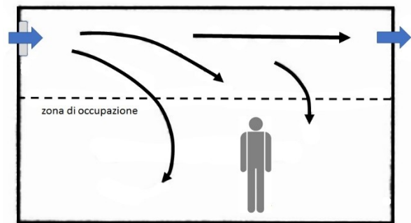
Figura 6. Sistema con corto circuito
