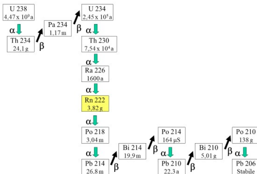
Figura 1 – Famiglia radioattiva dell'uranio: a metà catena è evidenziato il radon ( ^{222}\text{Rn} )
