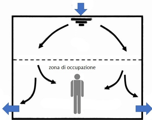
Figura 3. Sistema a miscelazione
