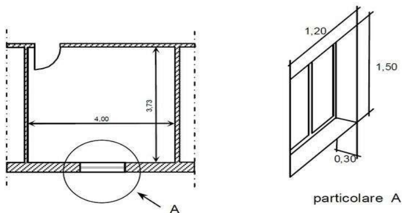
Pianta e dettaglio della finestra
