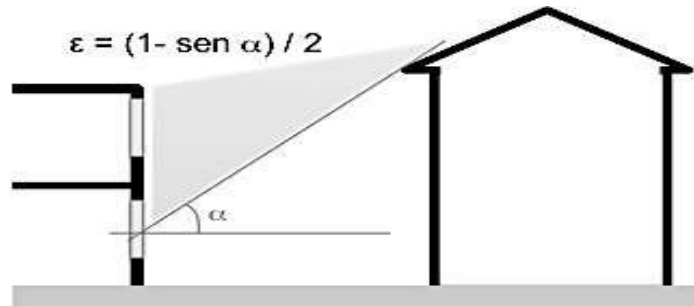
Figura D.4.1.c – Con ostruzione frontale (caso 1) (Formula alternativa al grafico di fig. D.4.1.a)
