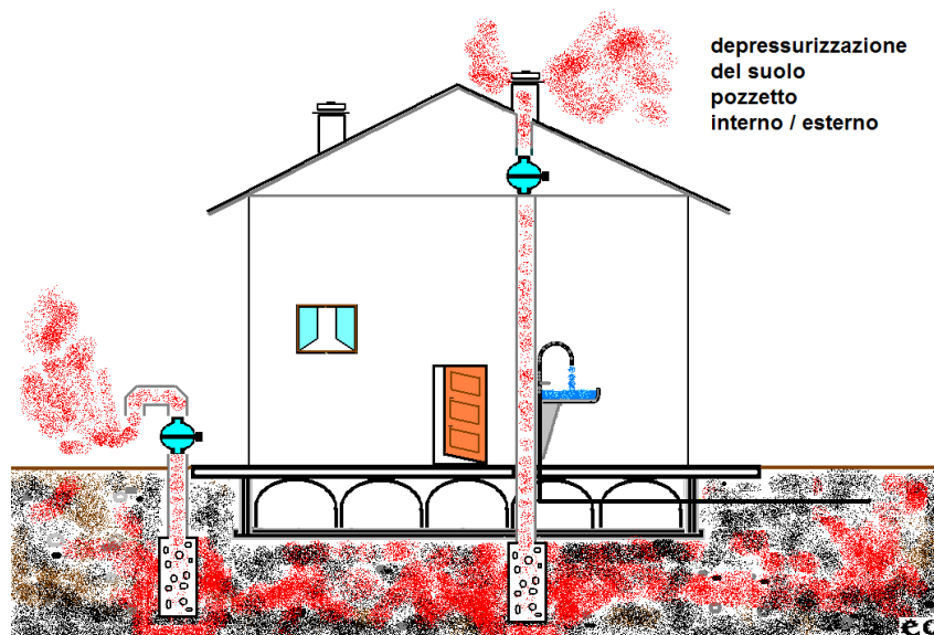
Figura 5 – Metodi attivi: depressurizzazione del suolo mediante pozzetto
