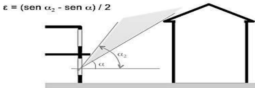
Figura D.4.1.e – Con ostruzione frontale e superiore (caso 3)
