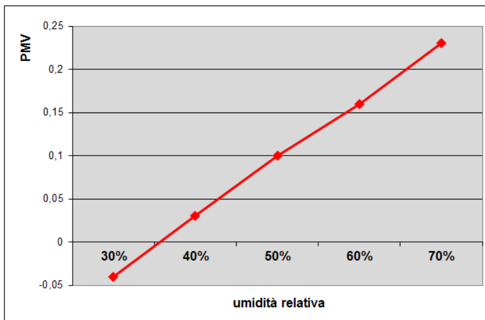
Figura 2 – Variazione dell'indice PMV in funzione dell'umidità relativa
