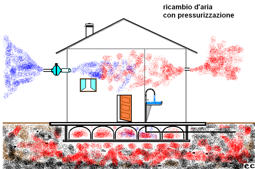
Figura 4 – Metodi attivi con ricambio aria e pressurizzazione: viene immessa aria dall'esterno
