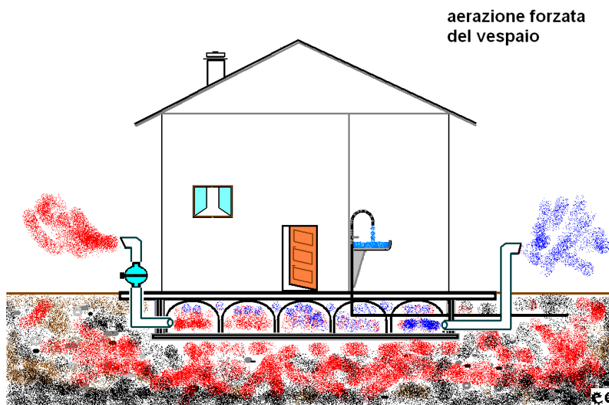
Figura 6 – Metodi attivi: aerazione forzata del vespaio
