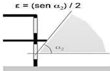
Figura D.4.1.d – Con ostruzione superiore (caso 2)
