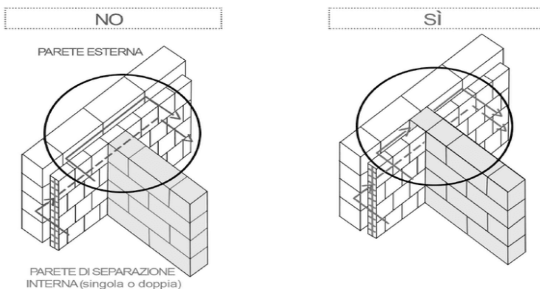
Realizzazione giunti: esempi di buone / cattive prassi
