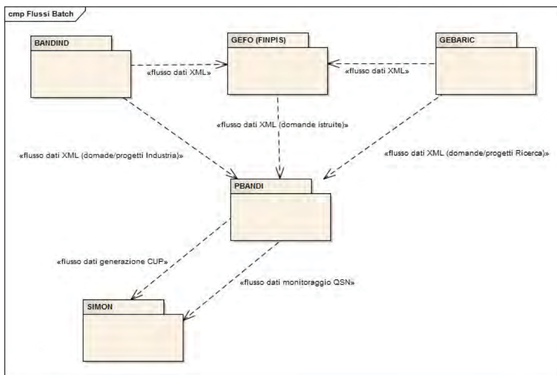
Figura 5 – Diagramma di contesto (parte flussi)
