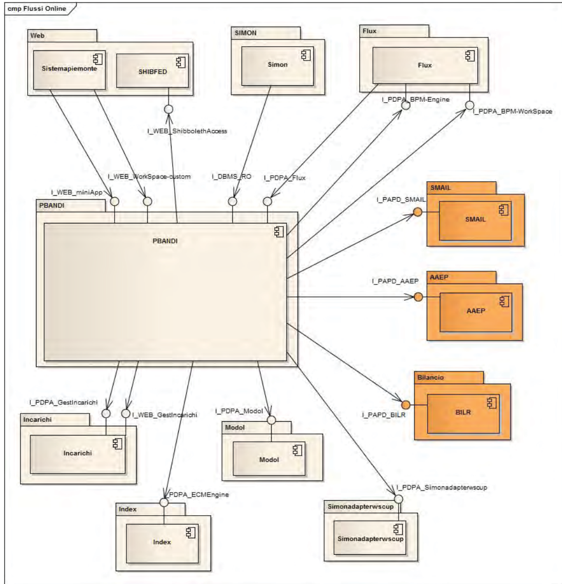
Figura 4 – Diagramma di contesto (parte online)
